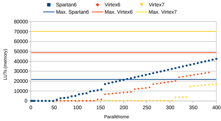
(a) MLUTs
