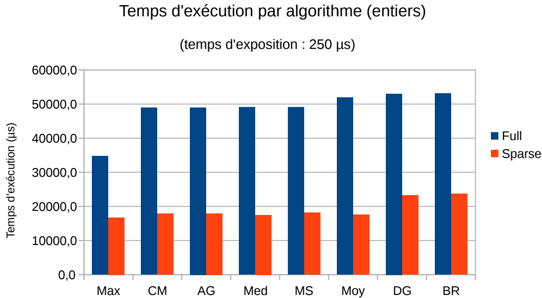
FIGURE 2.18 – Temps d'exécution en \mu s sur CPU pour la version entière des algorithmes
