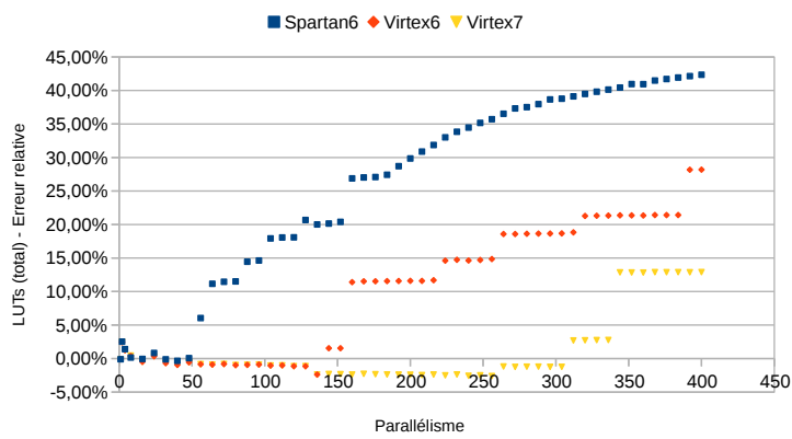
(b) LUTs
