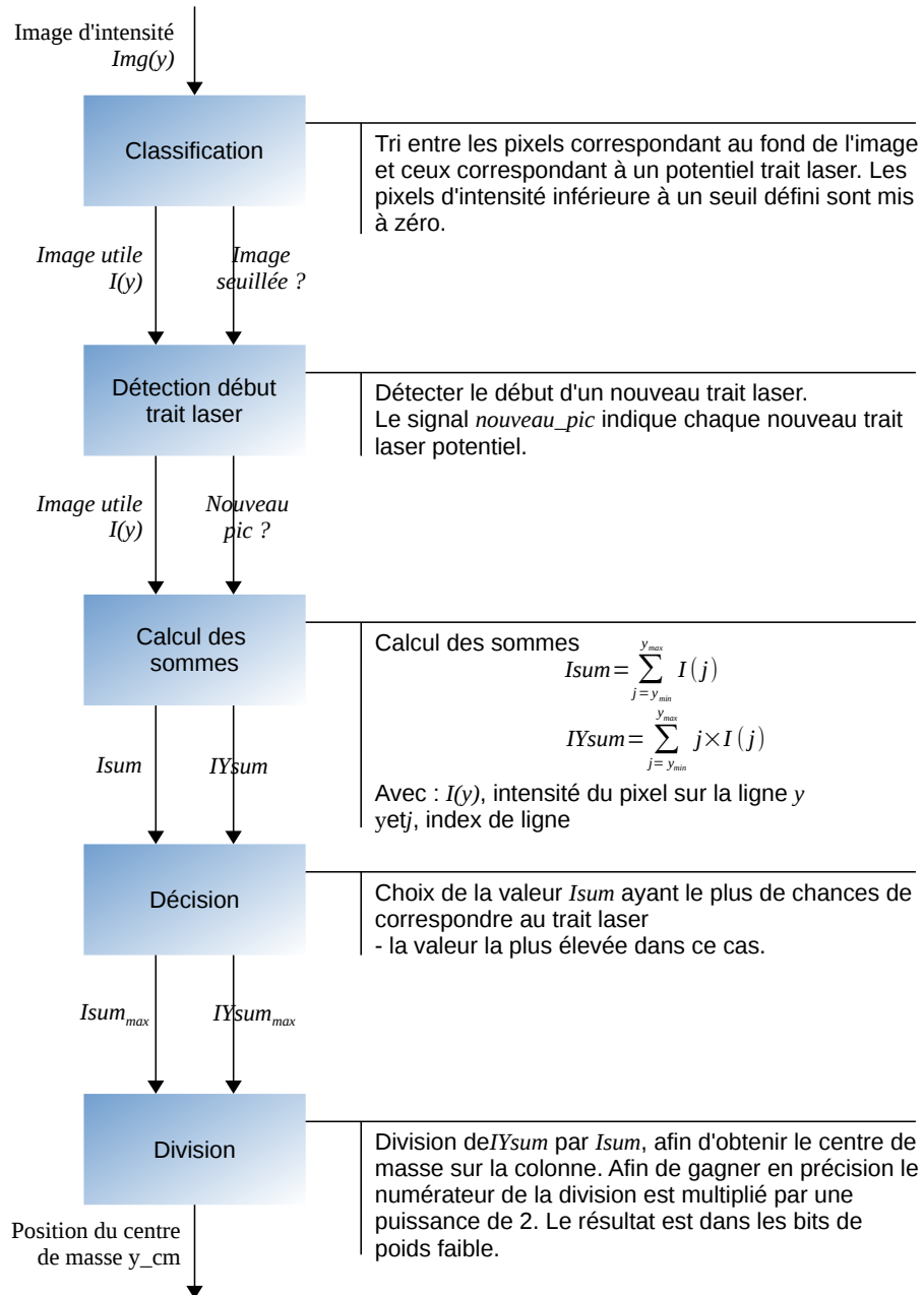
FIGURE 4.5 – Algorithme de détection de trait laser mis en œuvre sur une colonne d'image
