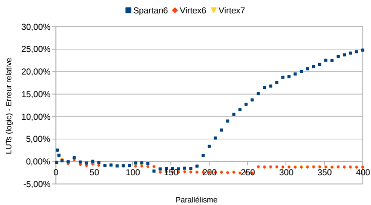
(c) LLUTs
