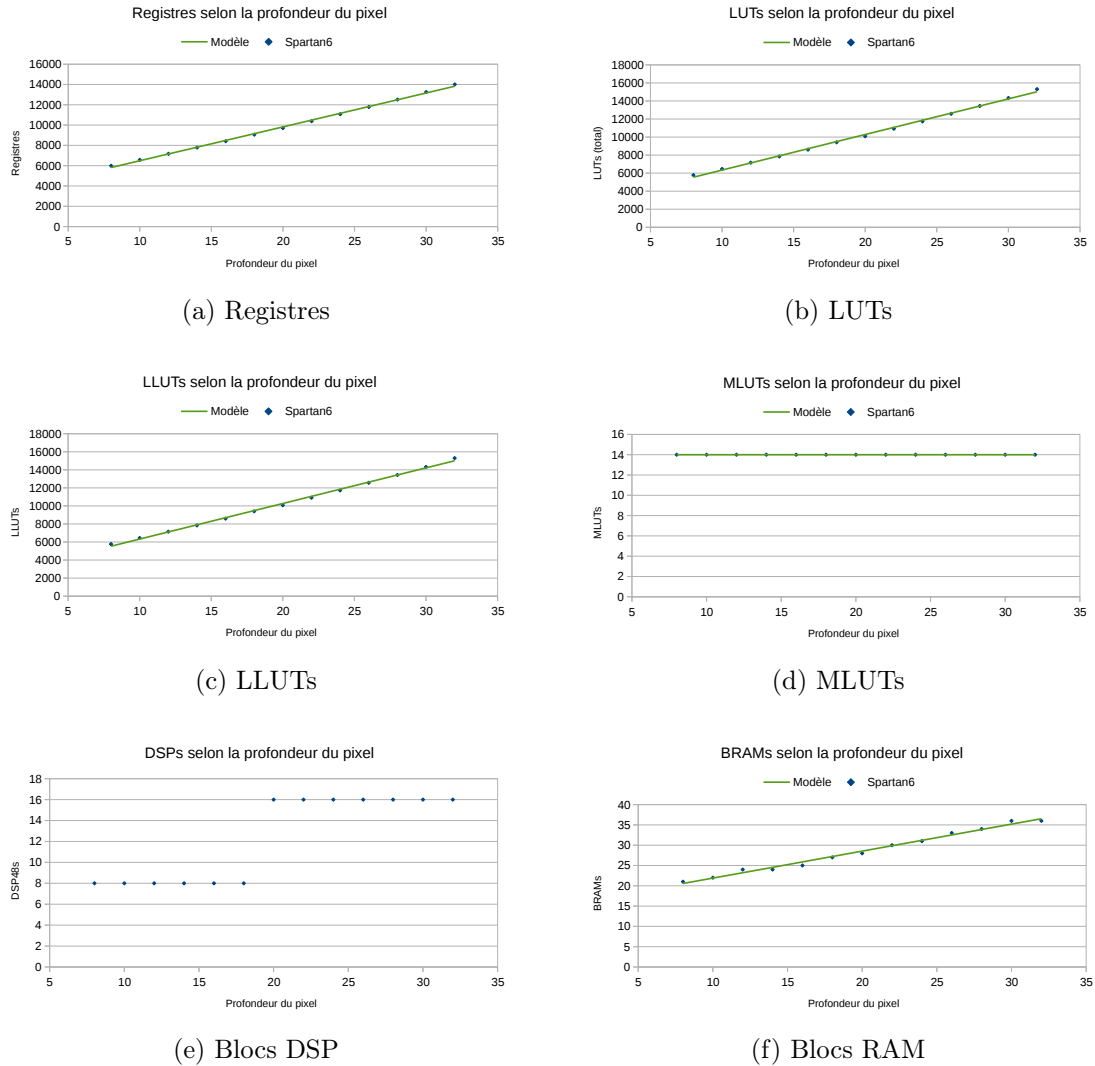
FIGURE 5.17 – Utilisation des ressources selon la profondeur des pixels pour un FPGA Spartan6 et modèles associés obtenus partie 5.6.1.2 avec les données du Spartan6.
