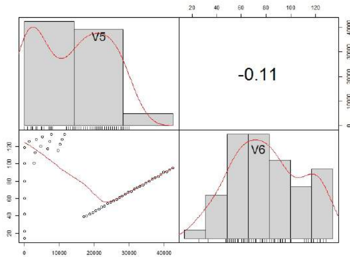
FIGURE 5.4 – Corrélations entre l'utilisation des MLUTs (V5) et des BRAMs (V6) pour les données du FPGA Spartan6. Figure obtenue avec le logiciel R pour le paramètre « nombre de pixels en parallèle ».
