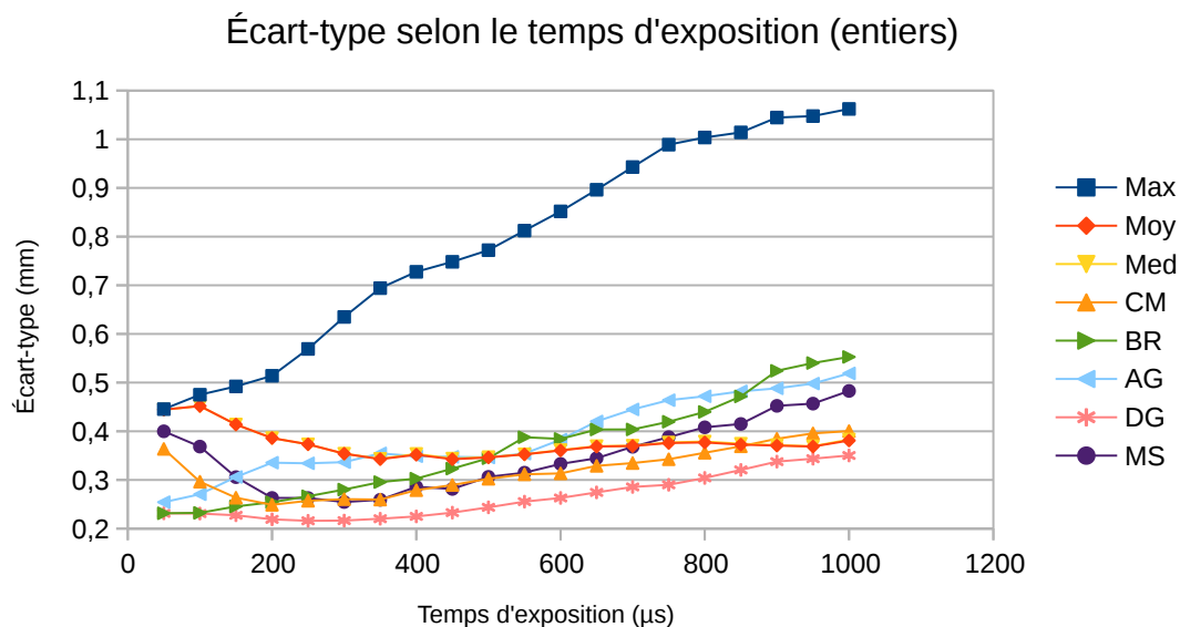
FIGURE 2.10 – Écart-type selon le temps d'exposition pour la version virgule fixe des algorithmes
