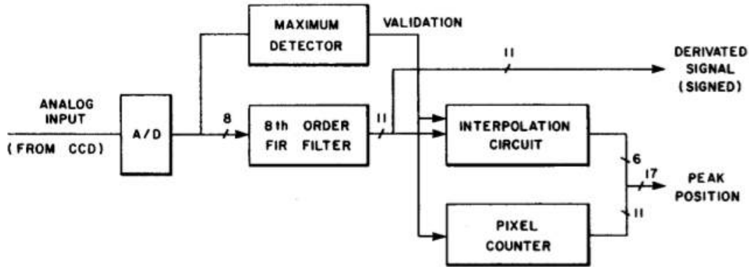
FIGURE 2.4 – Système de détection de trait laser mis en place par [BR86].
