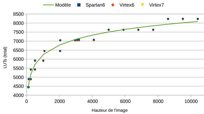
(b) LUTs
