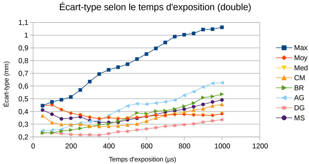
FIGURE 2.14 – Écart-type selon le temps d'exposition pour la version flottante double précision des algorithmes
