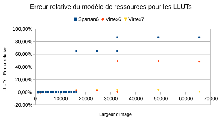
(b) LLUTs
