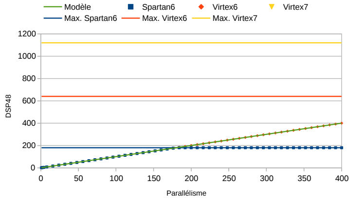
(b) Blocs DSP
