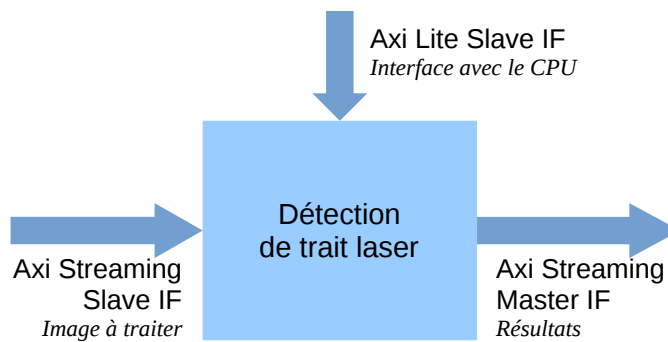
FIGURE 4.4 – Interfaces du module de détection de trait laser
