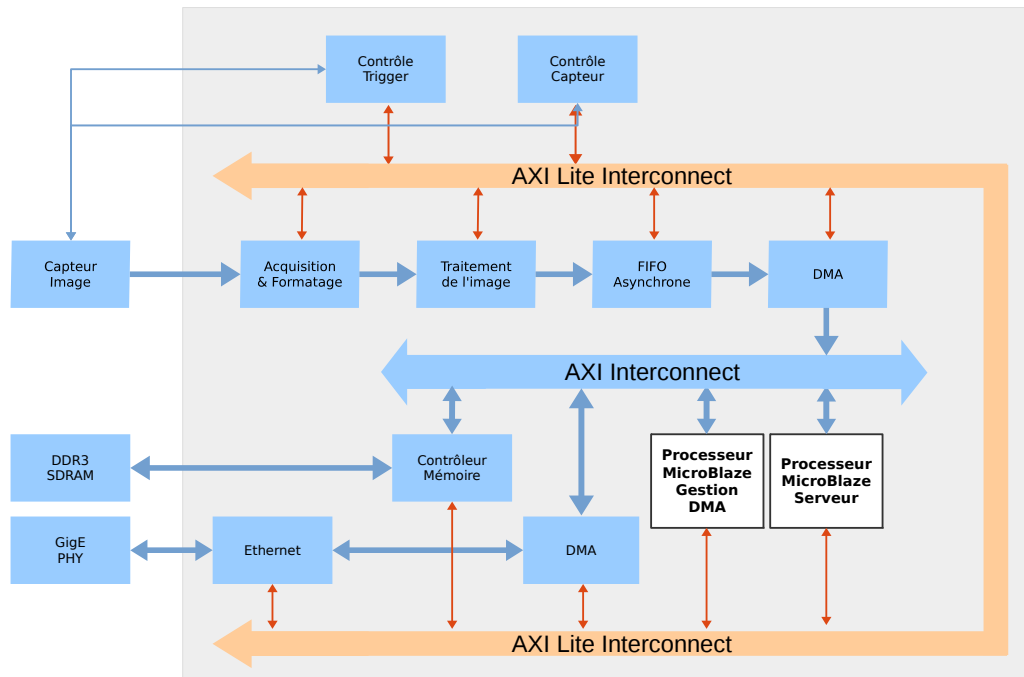
FIGURE 4.2 – Architecture matérielle présente dans le FPGA
