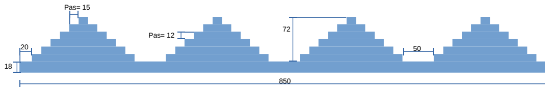
FIGURE 2.8 – Dimensions de la mire utilisée
