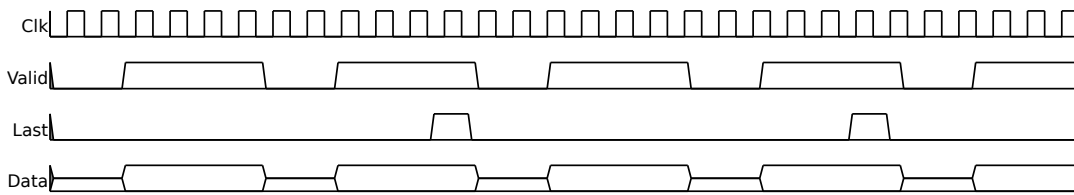
FIGURE 4.3 – Exemple de chronogramme des signaux utilisés pour le transfert d’image entre IPs. Cet exemple est pour une image de résolution 4x2 avec transfert d’1 pixel par cycle d’horloge.
