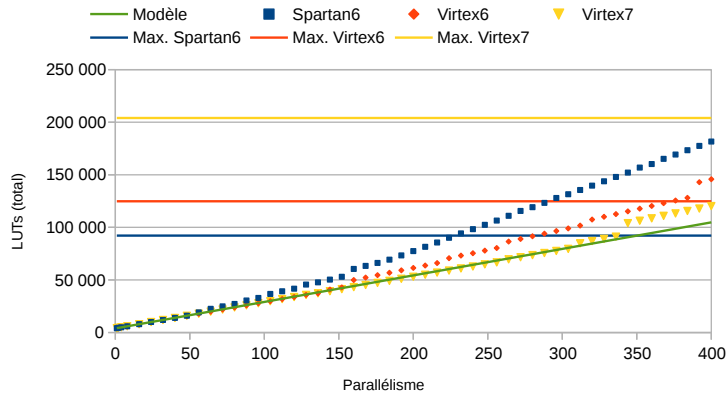
(b) LUTs
