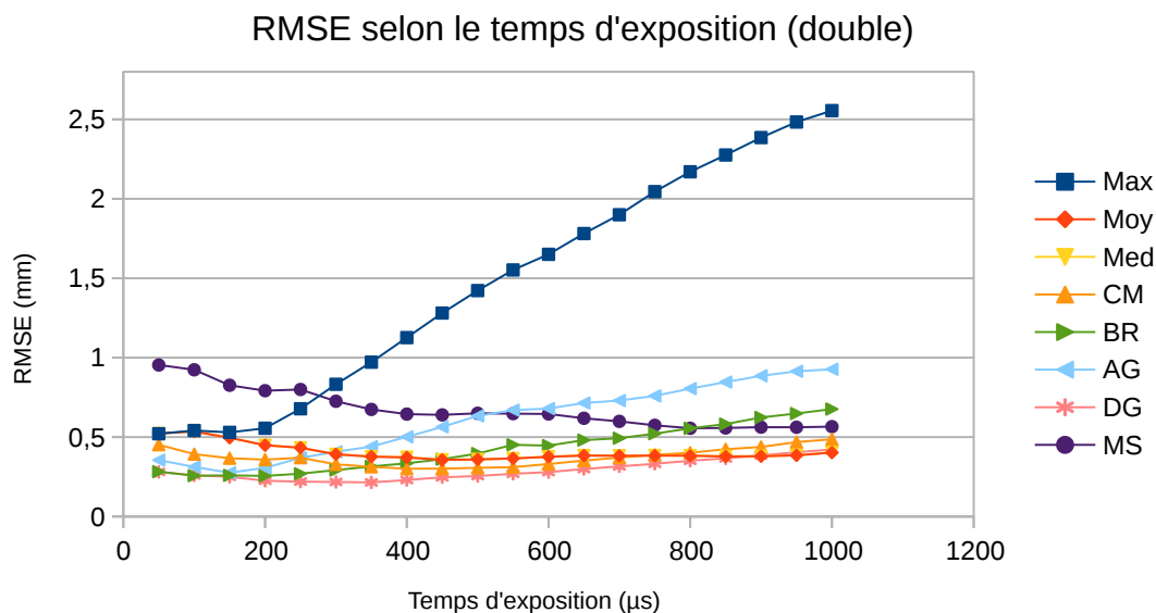
FIGURE 2.16 – Racine de l’erreur quadratique moyenne selon le temps d’exposition pour la version flottante double précision des algorithmes
