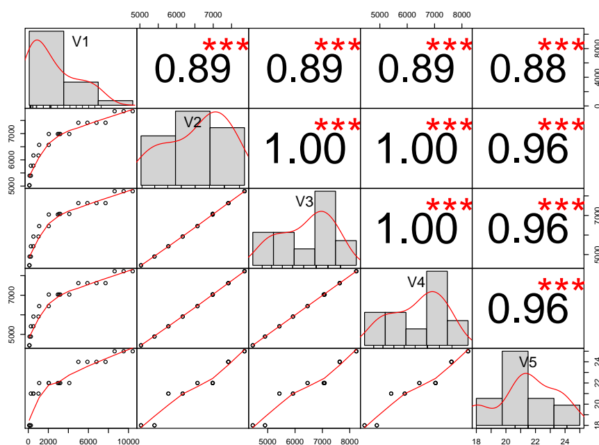
FIGURE 5.14 – Corrélations entre les valeurs du paramètre et les ressources utilisées pour le FPGA Spartan6. Figure obtenue avec le logiciel R pour le paramètre « hauteur d'image ».
