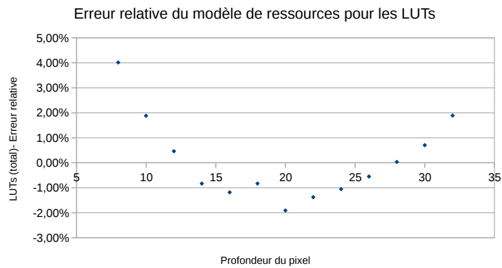
(b) LUTs
