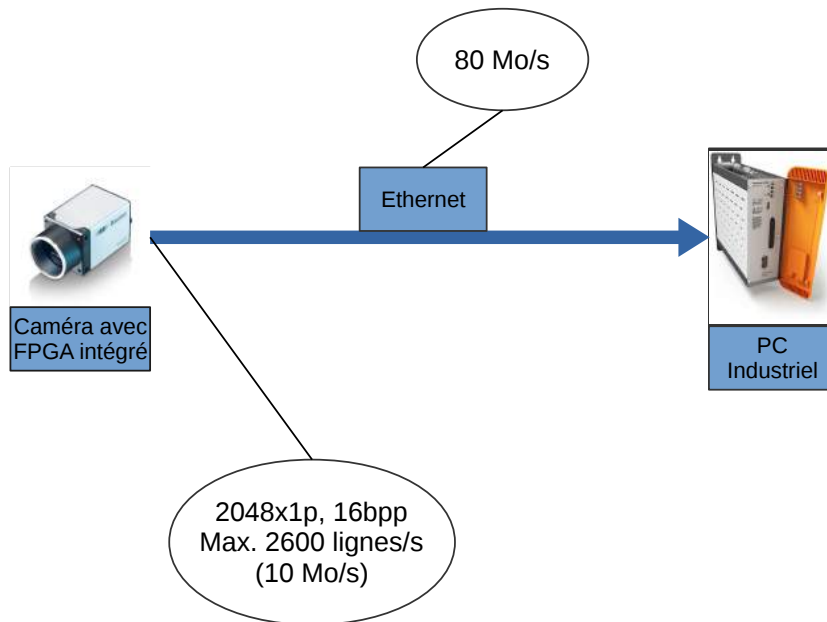
FIGURE 1.2 – Système de vision souhaité.
