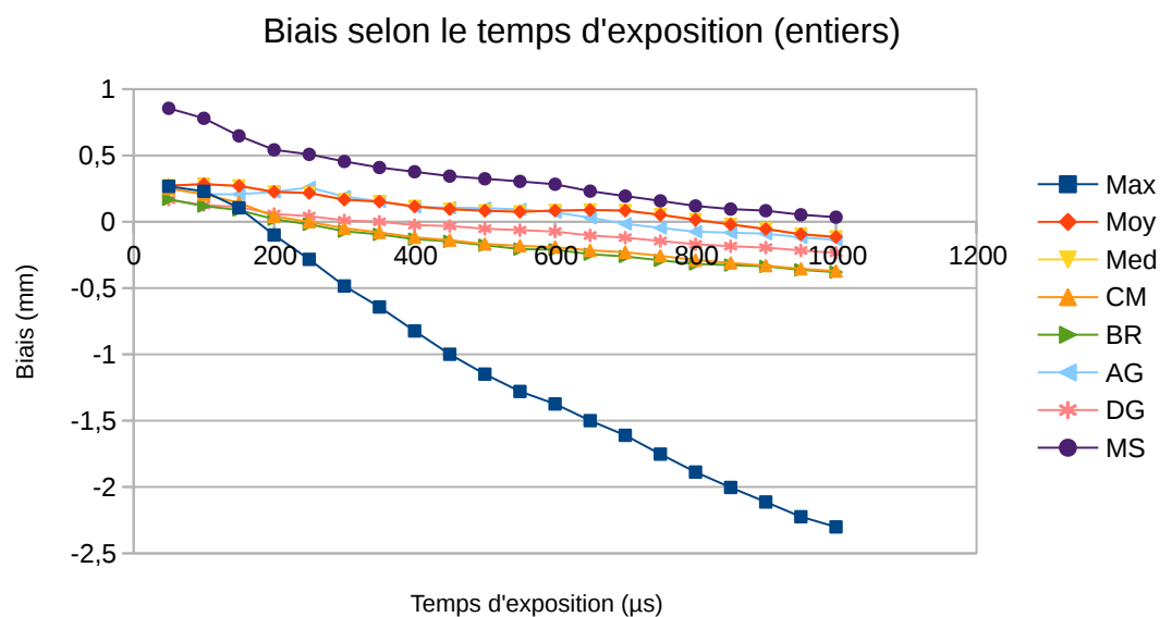
FIGURE 2.11 – Biais selon le temps d'exposition pour la version virgule fixe des algorithmes
