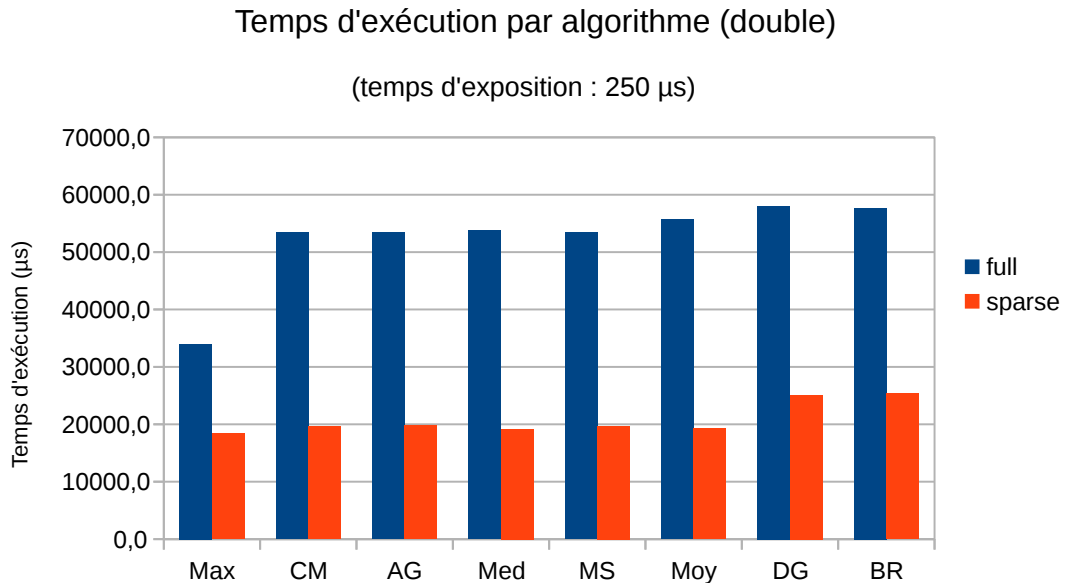
FIGURE 2.19 – Temps d'exécution en \mu s sur CPU pour la version flottante double précision des algorithmes
