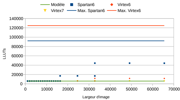
(c) LLUTs
