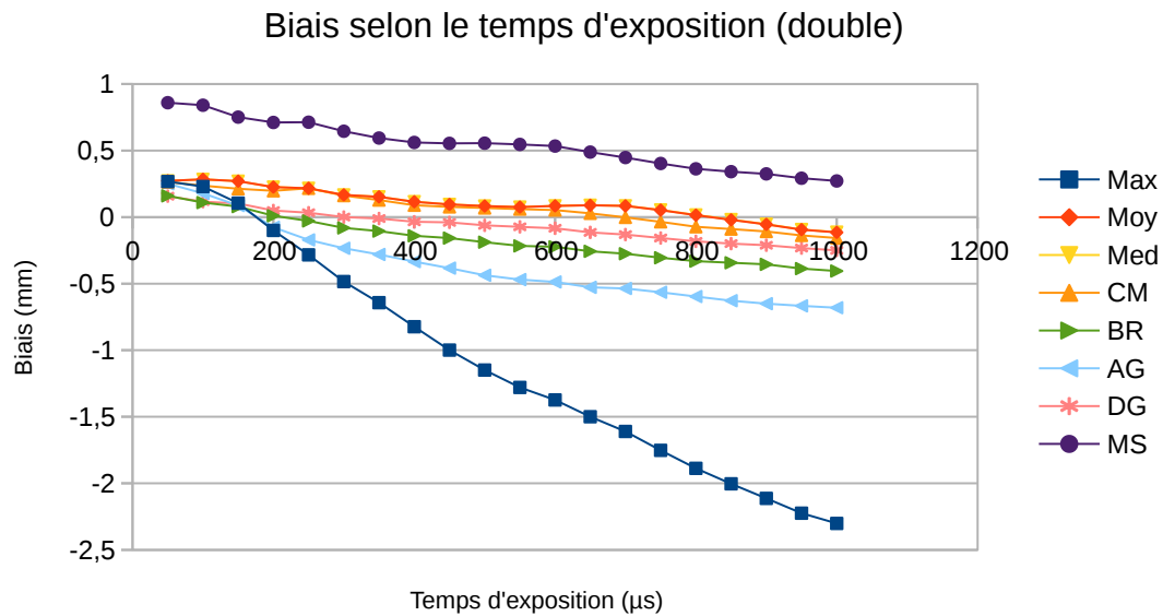
FIGURE 2.15 – Biais selon le temps d'exposition pour la version flottante double précision des algorithmes
