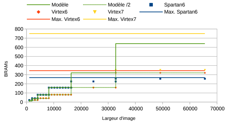
(b) Blocs RAM
