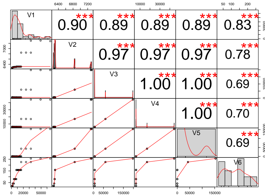
FIGURE 5.10 – Corrélations entre les valeurs du paramètre et les ressources utilisées pour les données du FPGA Spartan6. Figure obtenue avec le logiciel R pour le paramètre « largeur d'image ».
