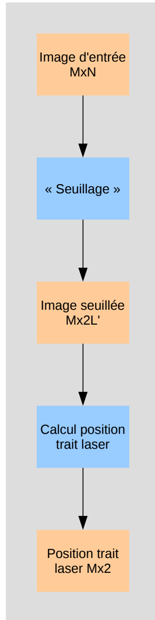
FIGURE 2.21 – Utilisation d’espace mémoire entre les fonctions pour les algorithmes développés en version sparse . Les tableaux sont sur fond orange.
