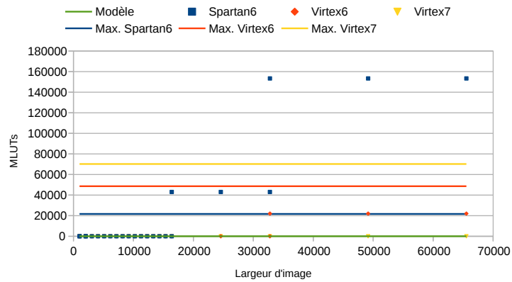
(a) MLUTs
