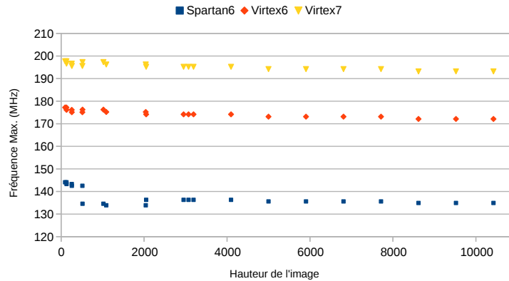
FIGURE 5.16 – Fréquence maximale après synthèse selon la hauteur d’image pour trois familles de FPGA.
