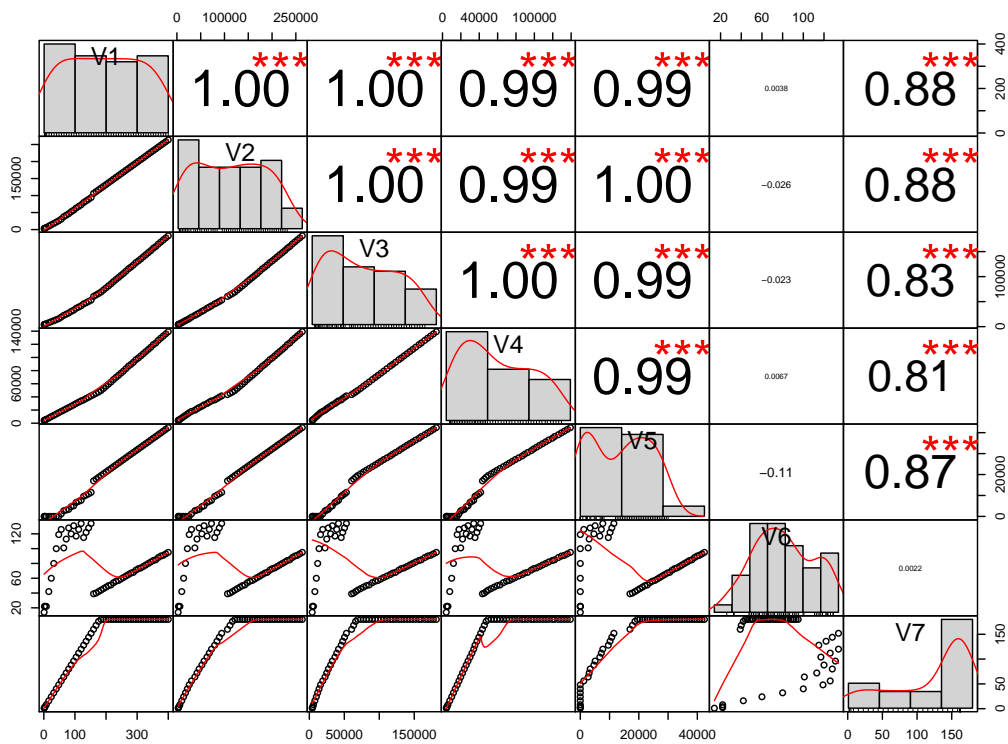
FIGURE 5.3 – Corrélations entre les valeurs du paramètre et les ressources utilisées pour les données du FPGA Spartan6. Figure obtenue avec le logiciel R pour le paramètre « nombre de pixels en parallèle ».
