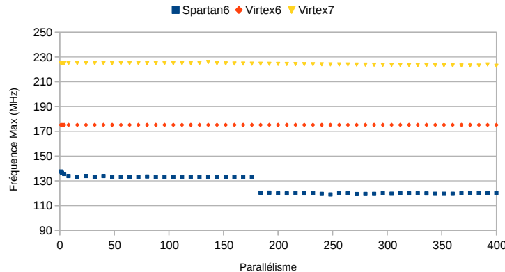
FIGURE 5.7 – Fréquence maximale après synthèse selon le nombre de pixels en parallèle pour trois familles de FPGA.
