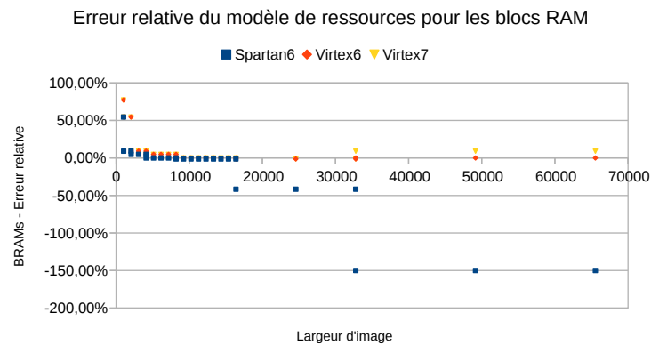
(a) Blocs RAM
