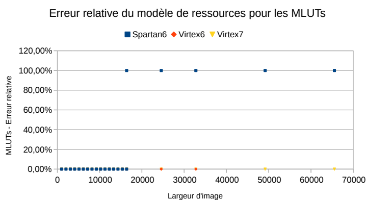
(c) MLUTs
