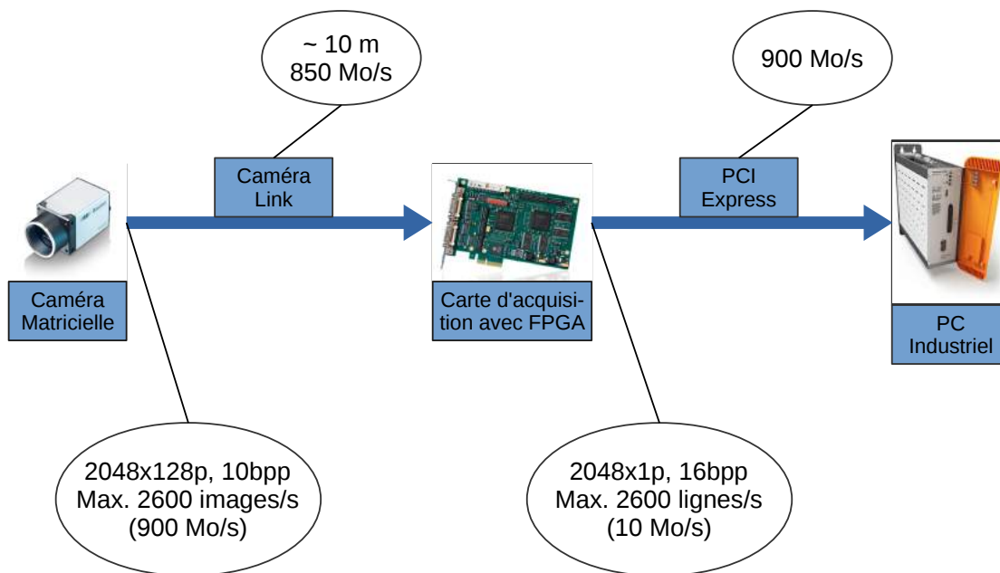
FIGURE 1.1 – Système de vision actuellement en place dans les machines Pattyn Bakery Division.
