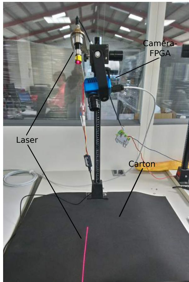
FIGURE 4.6 – Banc de test mis en place
