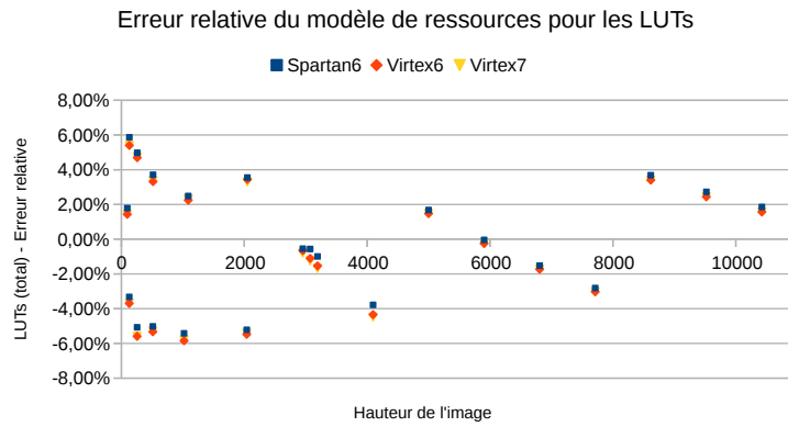
(b) LUTs
