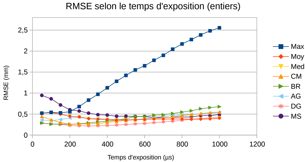
FIGURE 2.12 – Racine de l’erreur quadratique moyenne selon le temps d’exposition pour la version virgule fixe des algorithmes
