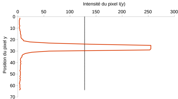
FIGURE 2.3 – Intensité des pixels sur une colonne d’image comprenant un trait laser
