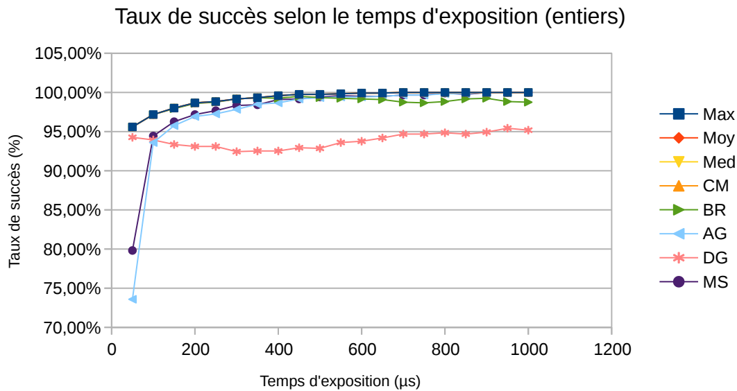
FIGURE 2.13 – Taux de succès selon le temps d’exposition pour la version virgule fixe des algorithmes
