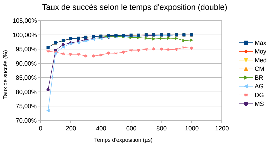
FIGURE 2.17 – Taux de succès selon le temps d’exposition pour la version flottante double précision des algorithmes
