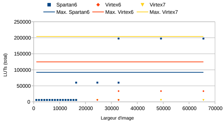
(b) LUTs
