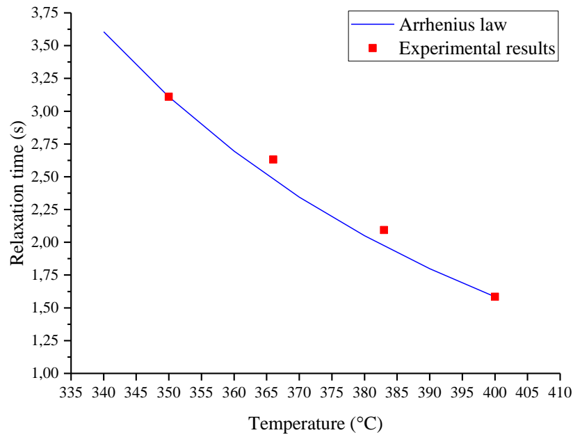
Figure 7: Le temps de relaxation en fonction de la température détermine étude expérimentale et loi d'Arrhenius
