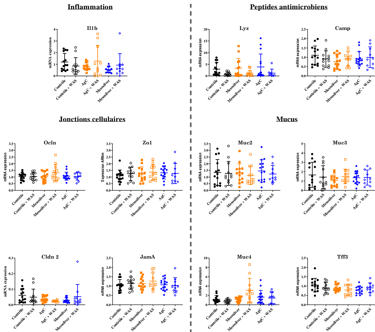
Figure 36 : effet d'une exposition sub-chronique d'une durée de 28 jours à 0,15 mg/kg p.c./jour de Mesosilver™ ou d'AgC sur l'expression d'ARNm dans le jéjunum. Les niveaux d'expression de gènes impliqués dans l'inflammation, la production de peptides antimicrobiens, la formation des jonctions serrées et la production de mucus ont été analysés. L'expression des gènes d'intérêt a été normalisée par celle du gène de référence Hprt et exprimée en 2^{44Ct} . Les différences significatives ont été évaluées par ANOVA à 1 facteur. n=12 animaux par groupe.
