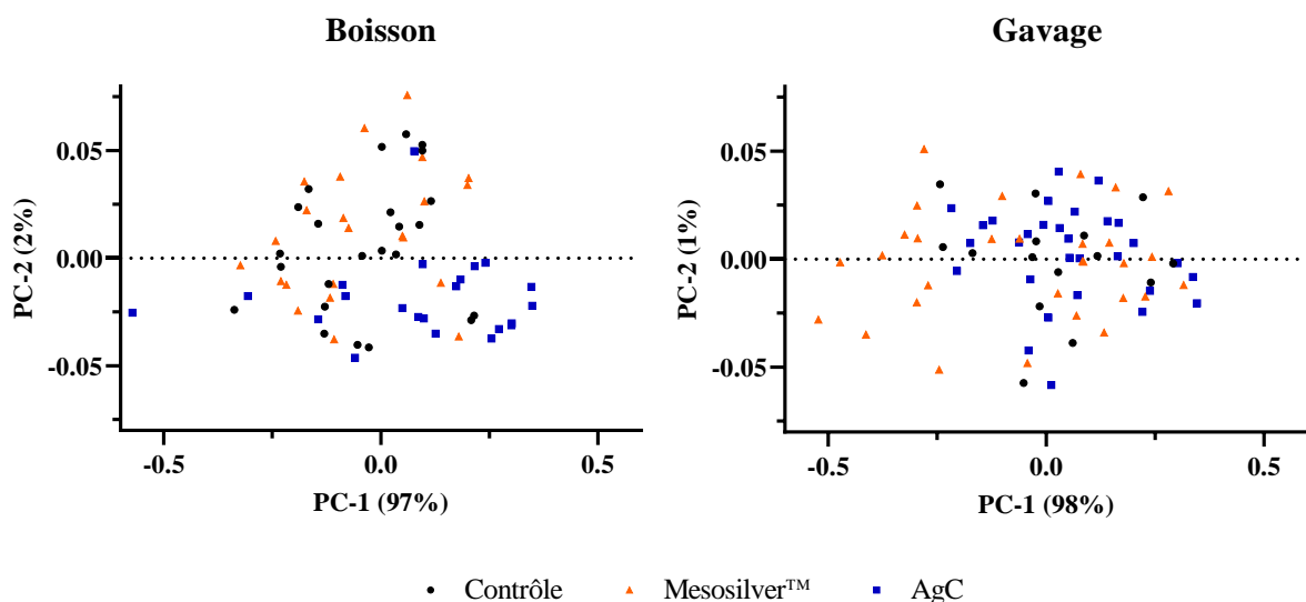
Figure 32 : analyse en composantes principales des spectres obtenus par spectroscopie proche infrarouge sur les animaux contrôles, exposés au Mesosilver™ ou à l'AgC par la boisson (environ 3 mg/kg p.c./jour) (A) ou par gavage (0,15 mg/kg p.c./jour) (B) sur une durée totale de 28 jours.
