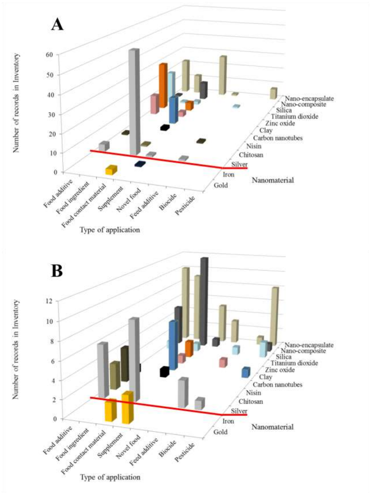
Figure 12 : nombre de produits contenant des nanomatériaux, et plus particulièrement des nanoparticules d'argent, dans le secteur agro-alimentaire sur le marché (A) et en développement (B) au cours de l'année 2014. (Peters et al., 2014)
