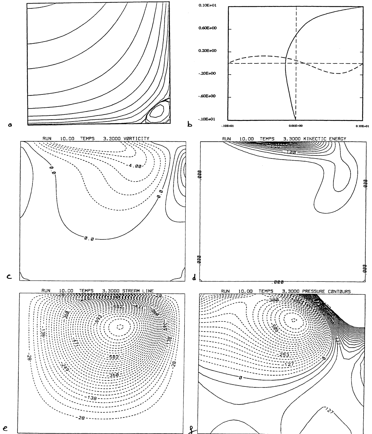
Figure II.16: Cavit  B) pour Re = 100   t = 3.3 ; h = 1/64 ; a) Lignes de courant coin inf rieur droit ; b) Profils m dians de la vitesse ; c) Isovorticite ; d) Energie ; e) Lignes de courant ; f) Isobares.
