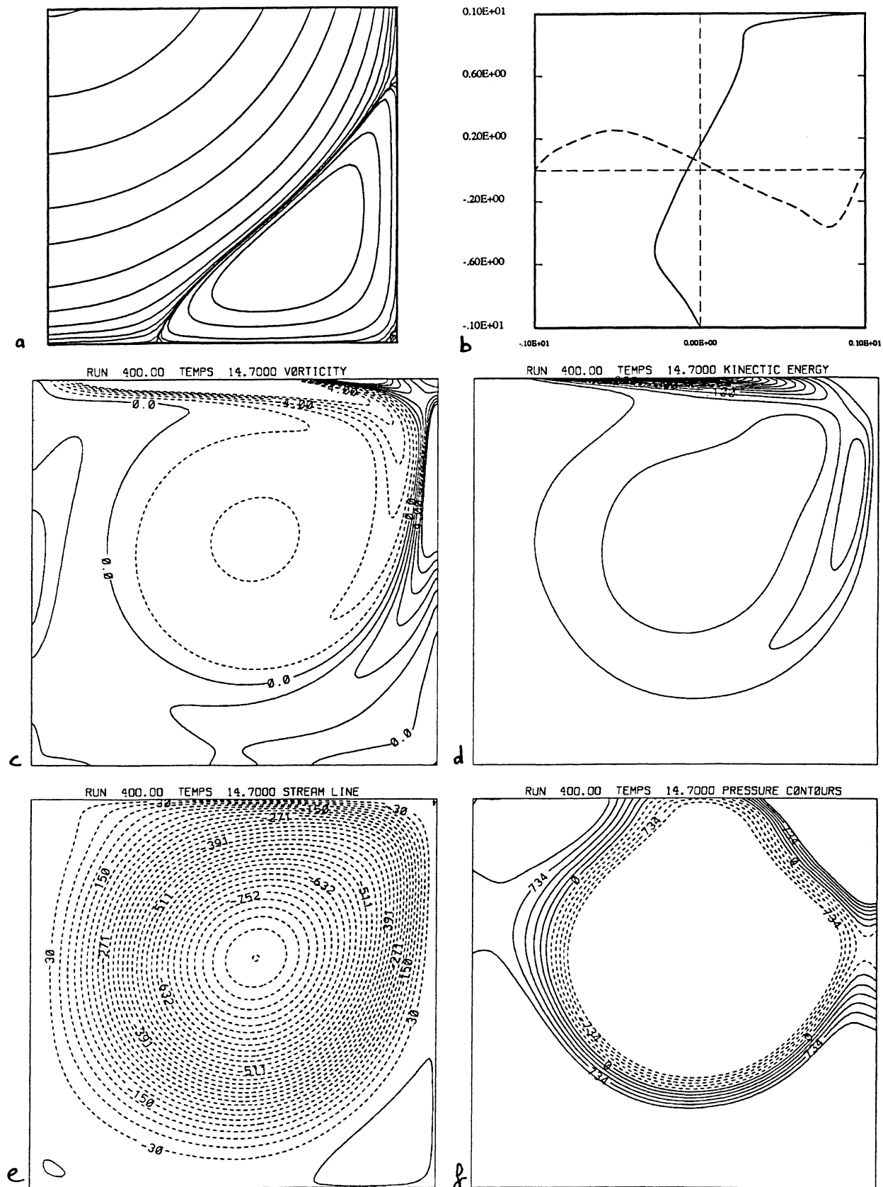
Figure II.18: Cavit  B) pour Re = 1000   t = 14.7 ; h = 1/128 ; a) Lignes de courant coin inf rieur droit ; b) Profils m dians de la vitesse ; c) Isovorticit  ; d) Energie ; e) Lignes de courant ; f) Isobares.
