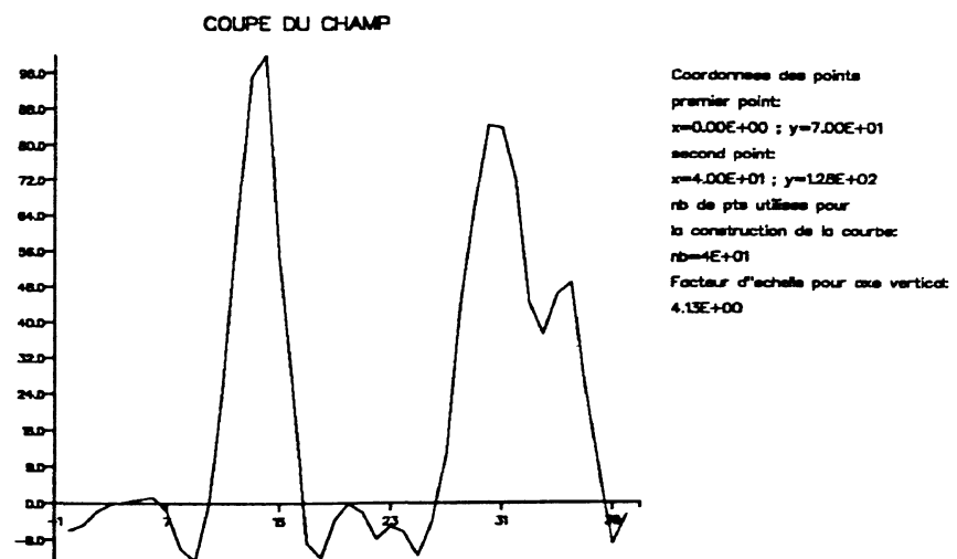
Figure I.16: Turbulence libre. Galerkin classique ( p = 4 ). Projection sur les 48 2 premiers modes : Champ et coupes à t = 0.6
