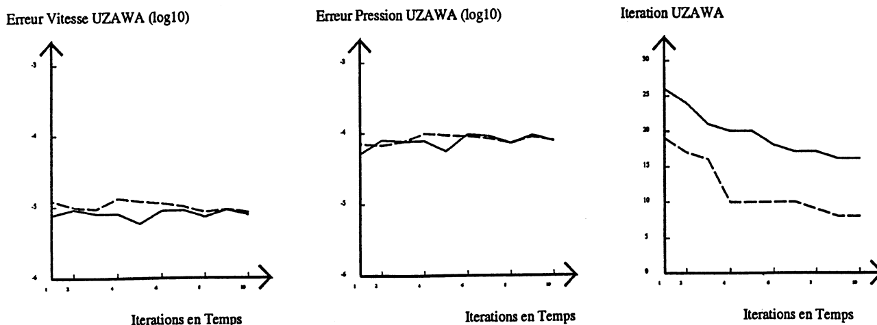
Figure II.9: PROBLEME DE STOKES GENERALISE dans la cavité B ) ; Erreurs et itérations de la méthode d'Uzawa pour 10 pas de temps de Navier-Stokes. En trait continue : sans préconditionnement ; En trait discontinue : préconditionnement de Labadie ; En trait pointillé : préconditionnement de Cahouet.
