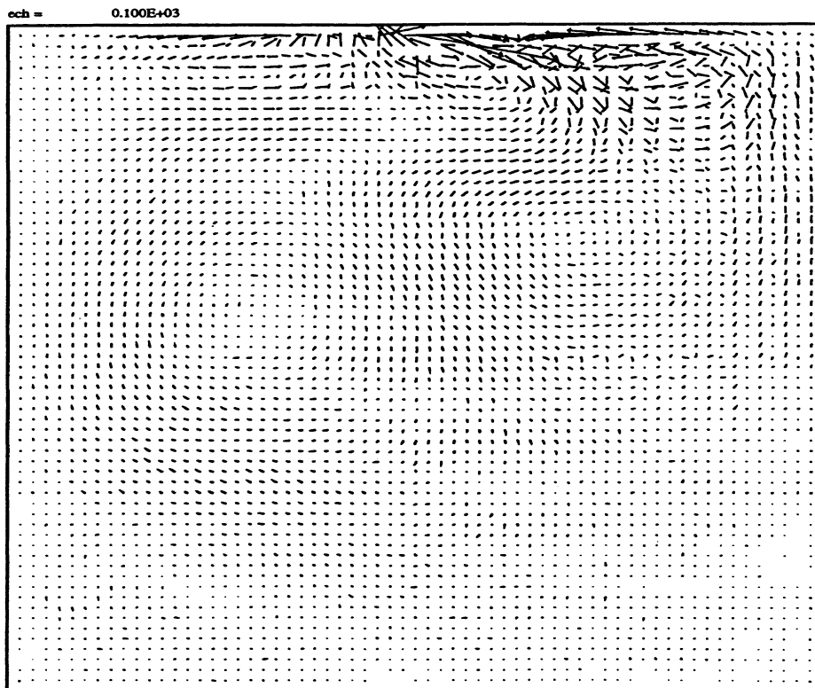
Figure IV.15: Cavité entraînée B) avec Re = 100 . Champ de différence ( \times 100 ) entre la vitesse obtenue par la méthode de Galerkin classique et celle obtenue par GNL3.
