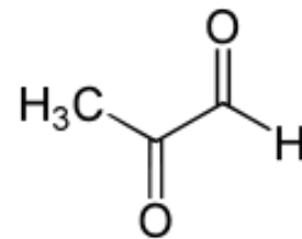
Methylglyoxal
