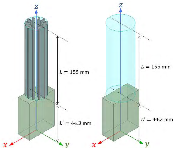
Figure 4.30 – Sonde corruguée de rayon 11.7 mm et sonde métallique de rayon 14.65 mm.
