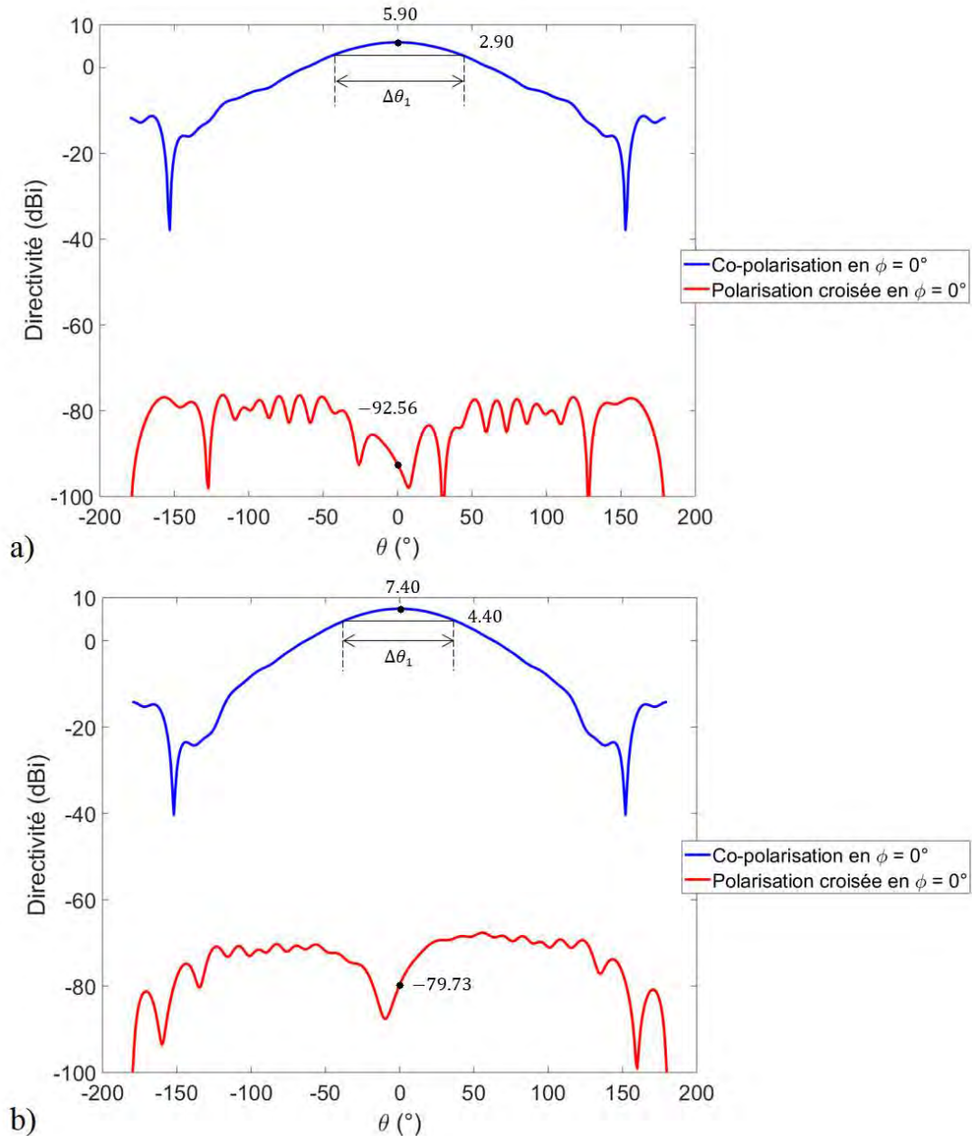
Figures 4.33 – Directivité (en dBi) de a) la sonde à métamatériaux et b) la sonde métallique à 6.5 GHz.
