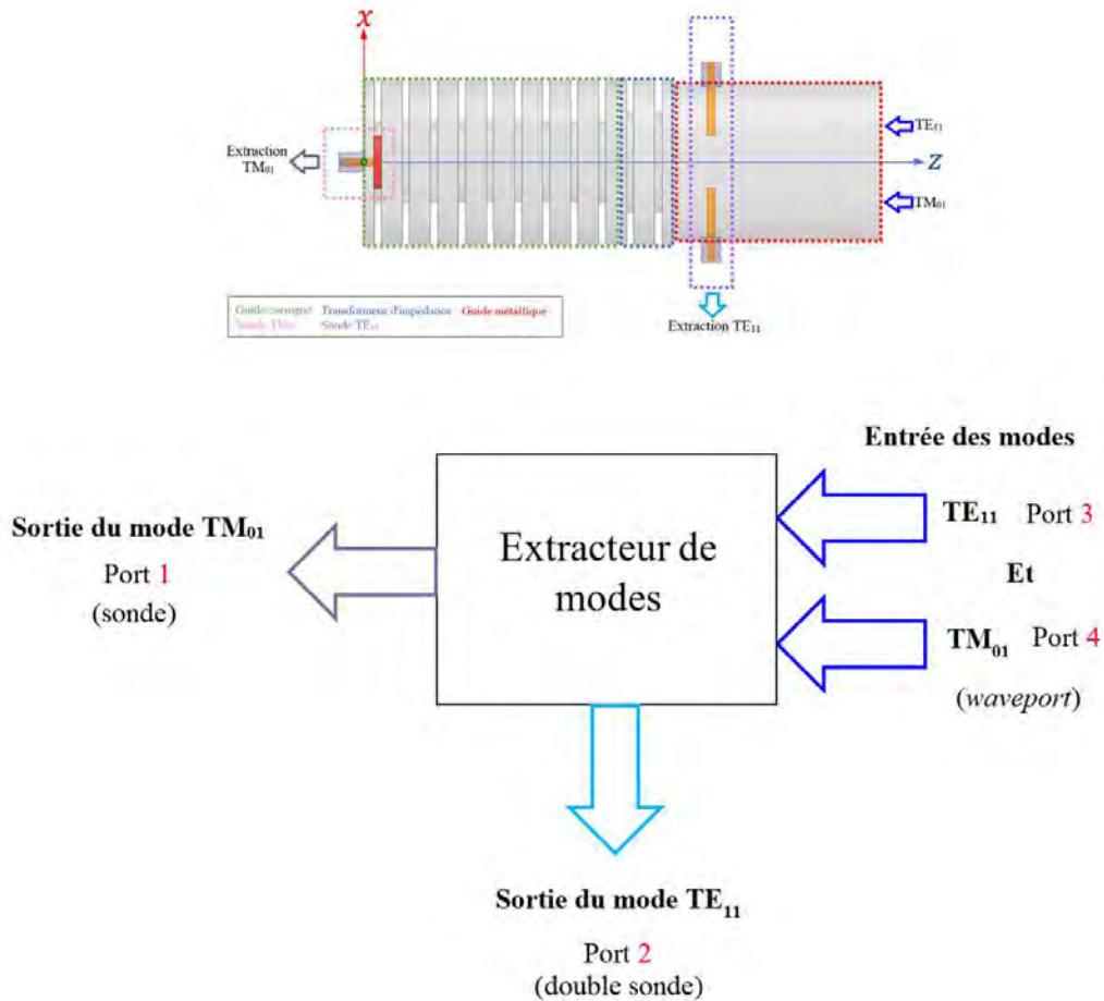
Figure 3.43 – Schéma de l'extracteur et numérotation des ports.
