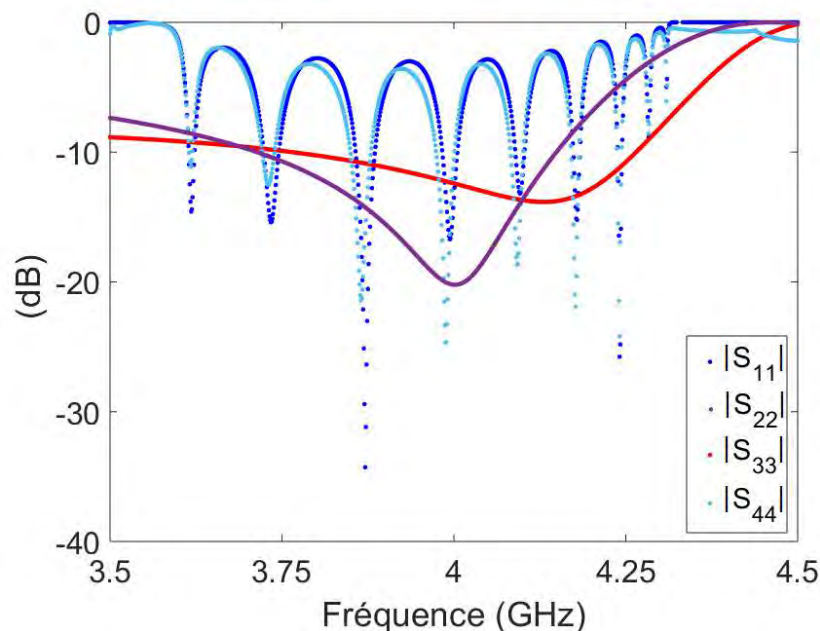
Figure 3.45 – Paramètres d'adaptation des sondes et à l'entrée de l'extracteur.
