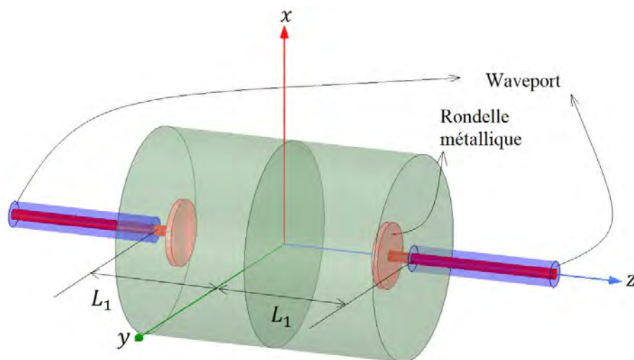
Figure H.2 – Simulation « TGC-TGC » avec L_1 = 45.4 mm.
