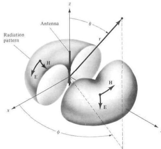
Figure 1.19 – Rayonnement omnidirectionnel [9].
