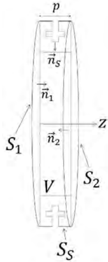
Figure 3.2 – V volume de la cellule élémentaire.
