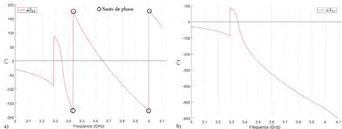
Figure H.6 – Phase du paramètre S_{21} a) avec sauts de phase de 2\pi et b) sans saut de phase grâce à la fonction unwrap .
