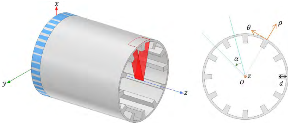
Figure 4.15 – Guide d'onde à corrugations longitudinales. La section en pointillés bleus est celle utilisée dans HFSS et celle en rouge dans la TME. La périodicité angulaire de ce métamatériau est de \alpha = 30^\circ , la profondeur de corrugation est de d = 18.2 \text{ mm} .
