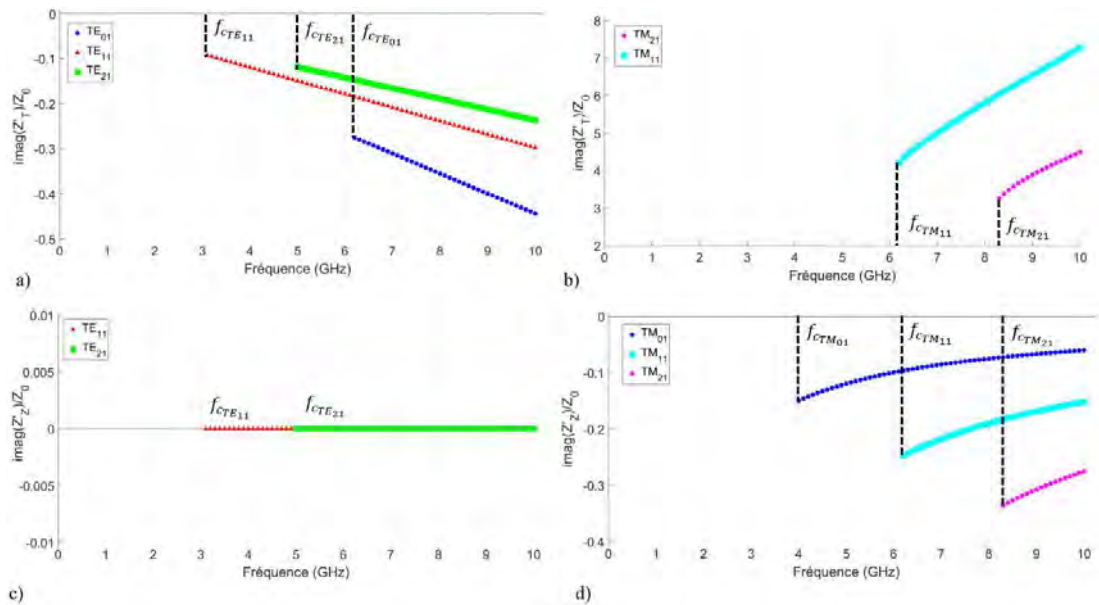
Figures 2.19 – Parties imaginaires des impédances de surface normalisées a) Z'_T (modes TE), b) Z'_T (modes TM), c) Z'_Z (modes TE) et d) Z'_Z (modes TM) des 6 premiers modes propagatifs d'un guide métallique de rayon A = 30 mm.
