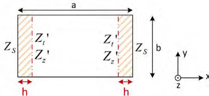
Figure 5.4 – Coupe transversale d'un guide rectangulaire avec deux parois à métamatériaux [1].
