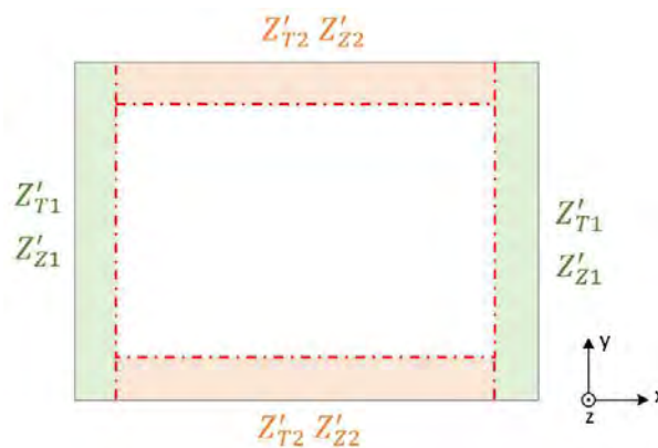
Figure 5.5 - Coupe transversale d'un guide rectangulaire avec quatre parois à métamatériaux.
