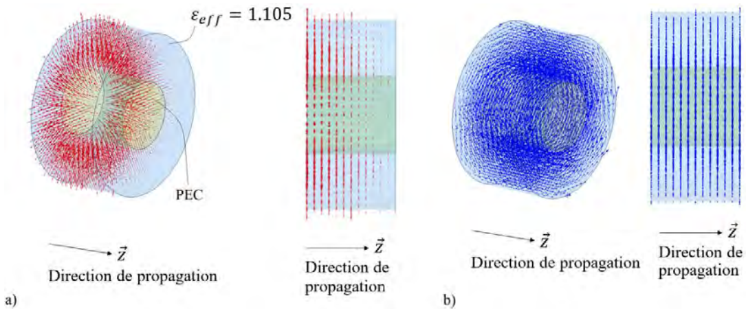
Figures 1.3 – Distributions du mode TEM dans un câble coaxial a) champ électrique et b) champ magnétique.
