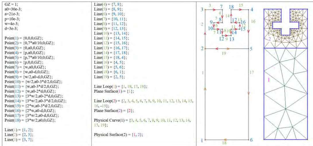
Figure G.6 – Fichier « .geo » et sa cellule élémentaire maillée sur GMSH.
