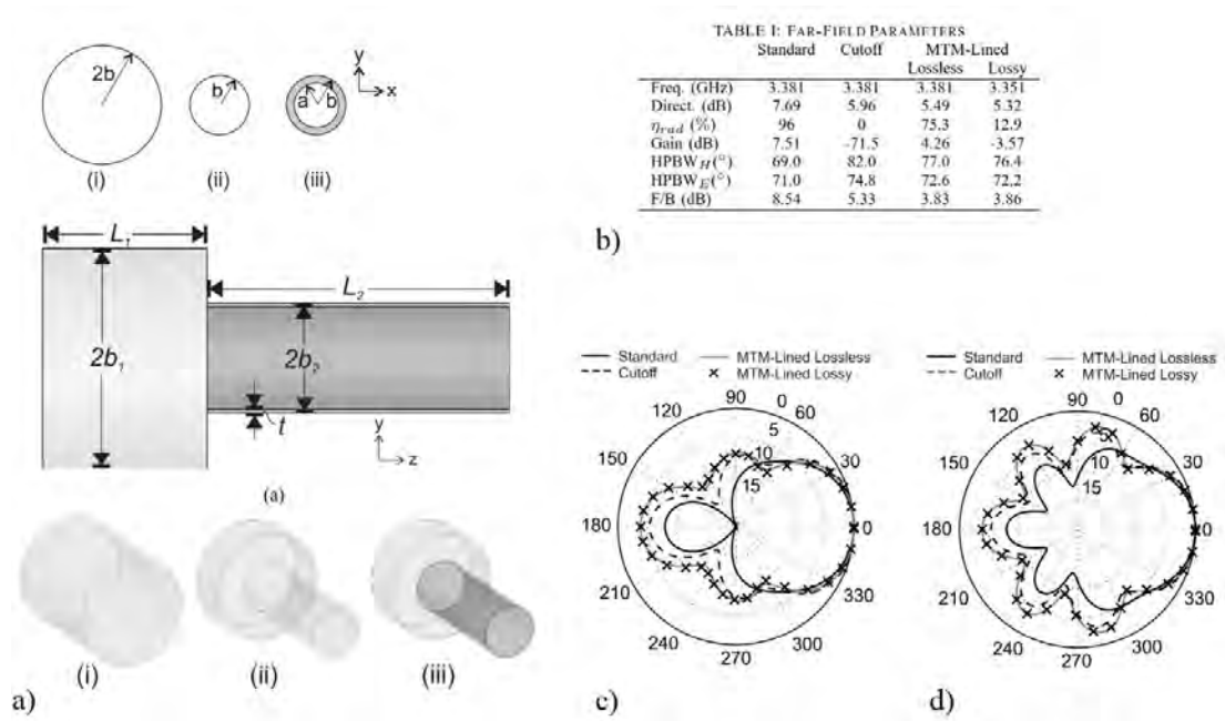
Figures 1.26 – a) OEWG (i) standard, (ii) sous coupure et (iii) à métamatériaux, b) tableau des paramètres de rayonnement ; c) coupe plan E et d) coupe plan H du diagramme de rayonnement [35].
