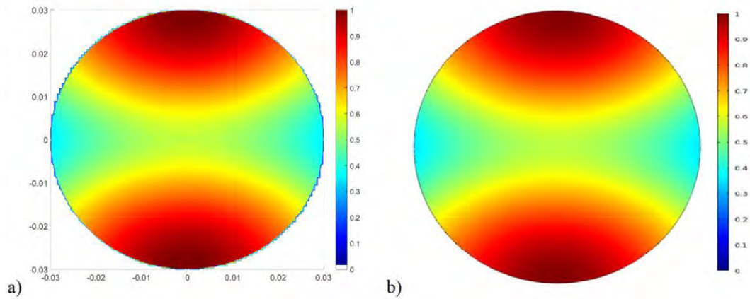
Figures 2.5 – Amplitude normalisée du champ magnétique du mode TE 11 dans un guide métallique, à la fréquence f = 3.5 GHz avec a) TME et b) COMSOL.
