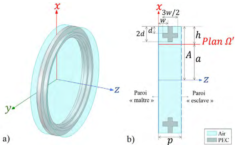
Figure 3.12 – Cellule élémentaire 3-D utilisée dans HFSS.
