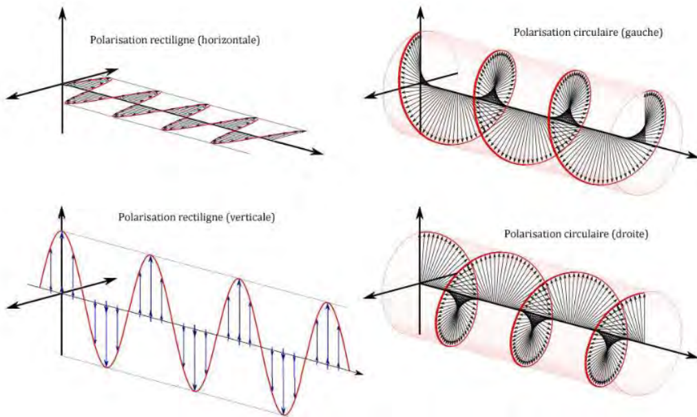
Figure 1.24 – Exemple de polarisations.
