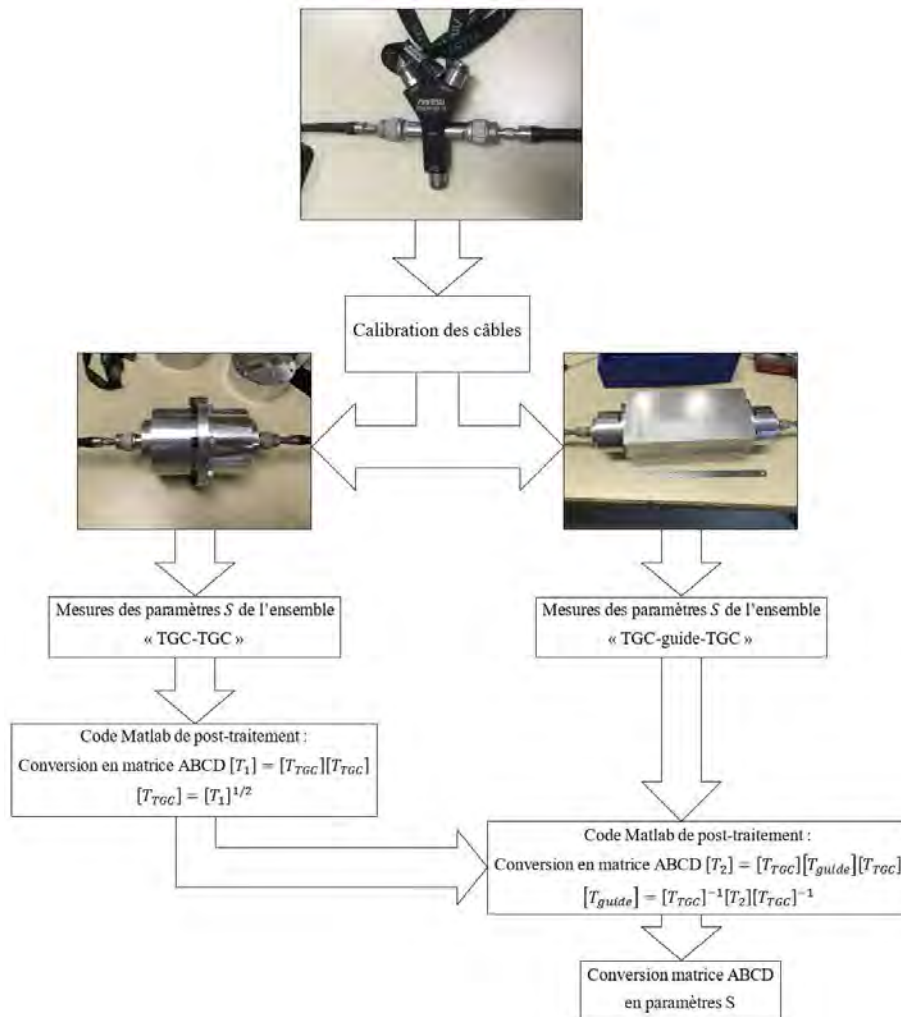
Figure 3.33 – Schéma de principe pour obtenir les paramètres S des guides métallique ou corrugué entre les deux TGC.
