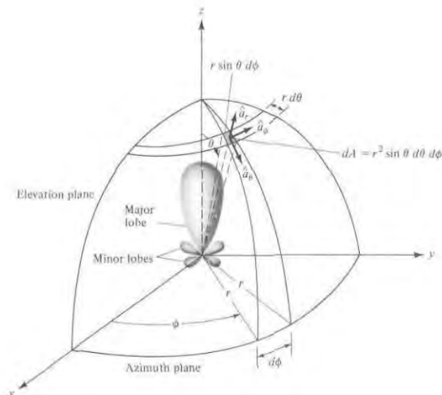
Figure 1.17 – Exemple de diagramme de rayonnement [9].
