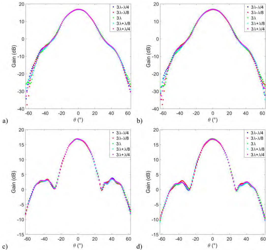
Figures 4.46 – Gain de l’antenne SGH705 à 6. 5 GHz mesuré avec a) la sonde corruguée et b) la sonde métallique dans le plan \phi = 0^\circ et mesuré c) la sonde corruguée et d) la sonde métallique dans le plan \phi = 90^\circ .
