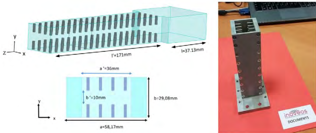
Figures 1.27 – OEWG avec métamatériau PIC [25].
