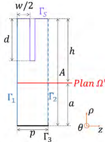
Figure 3.40 – Cellule élémentaire du transformateur d'impédance, avec A = 34.2 mm, a = 13.68 mm, d = 13.5 mm, h = 20.52 mm, p = 11.5 mm, et w = 8.5 mm.
