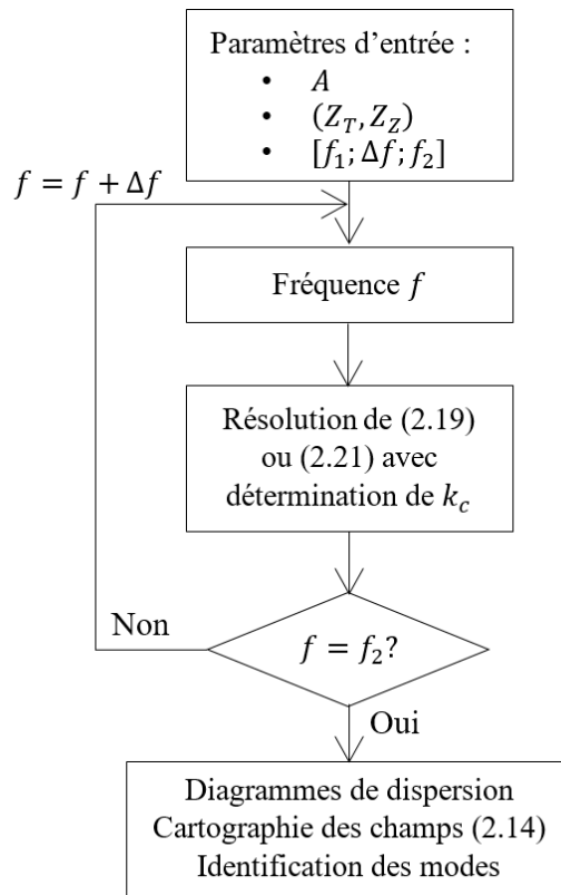
Figure 2.2 – Algorithme général de la TME.
