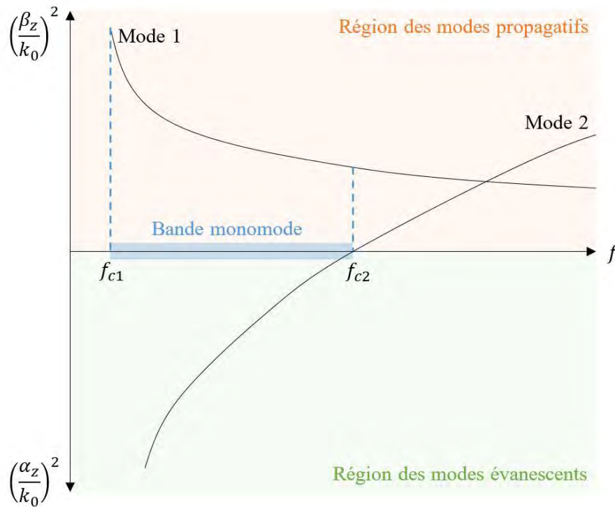
Figure 1.5 – Exemple de diagramme de dispersion.
