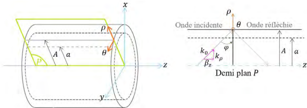
Figure 2.13 – Propagation d'une onde électromagnétique dans un guide cylindrique et définition de l'angle d'incidence \varphi .
