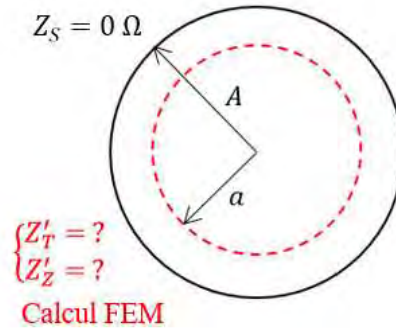
Figure 3.5 – Schématisation du guide d'onde métallique.
