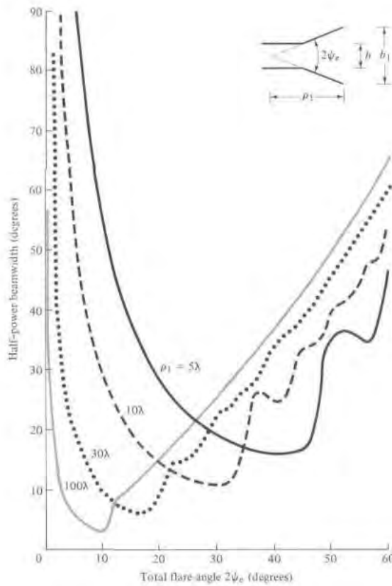
Figure 1.21 – Angle d’ouverture à -3 dB d’un cornet de type plan E en fonction de l’angle d’ouverture du cornet [9].
