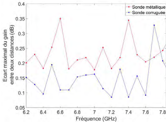
Figure 4.48 – Écart maximal du gain dans l'axe entre deux distances (pire cas) pour chaque sonde.
