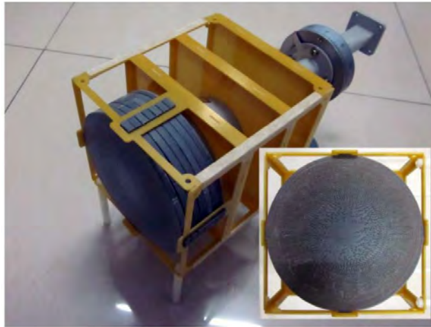
Figure 1.38 – Prototype réalisé dans [51].
