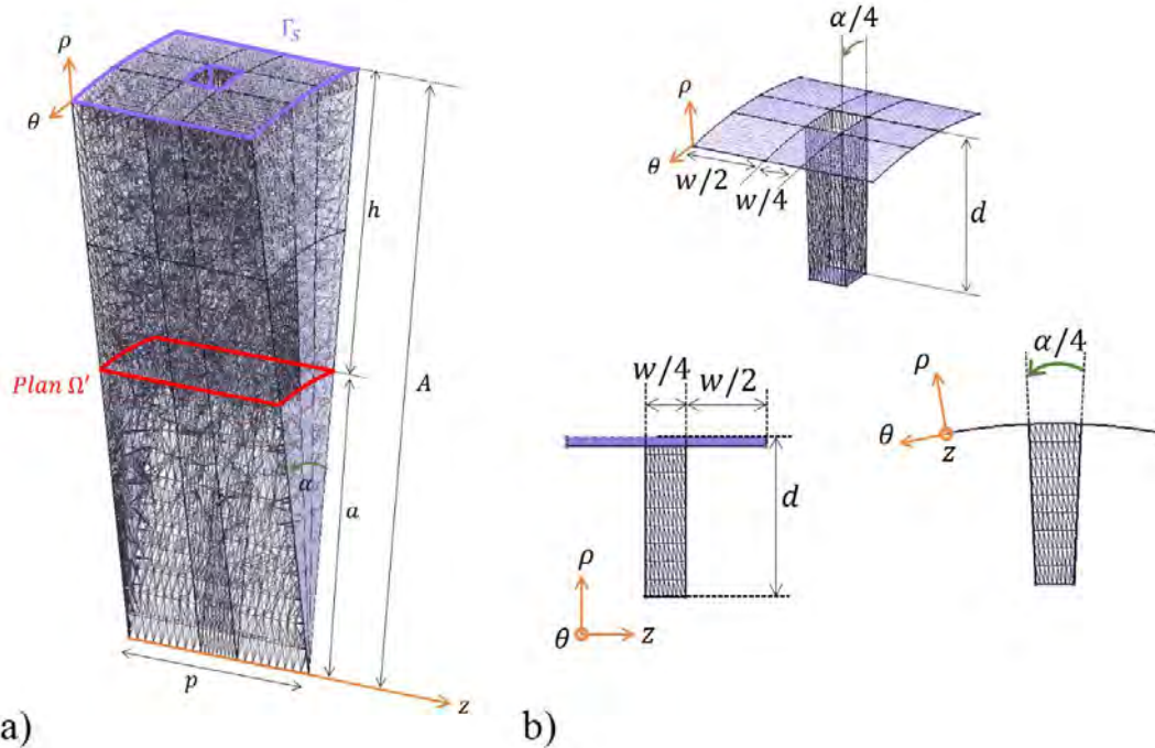
Figure 4.20 – a) Cellule élémentaire 3-D et son maillage avec A = 30 mm, a = 15 mm, \alpha = 20^\circ , d = 8 mm, h = 15 mm, p = 10 mm et w = 8 mm et b) différentes vues de la partie PEC.
