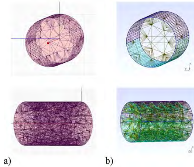
Figure 4.7 – Maillages utilisés dans a) HFSS et b) GetDP+GMSH.
