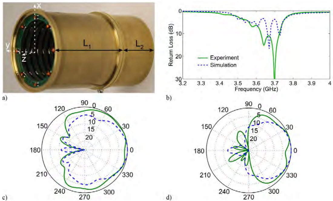
Figures 1.25 – a) OEWG, b) coefficient de réflexion ; c) coupe plan E et d) coupe plan H du diagramme de rayonnement à 3.70 GHz. Les mesures sont représentées en vert, et les simulations en pointillées bleus [35], [36].
