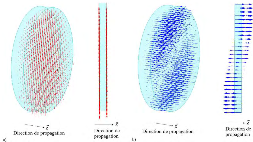
Figures 1.1 – Distributions du mode TE 11 dans un guide cylindrique métallique a) champ électrique et b) champ magnétique.
