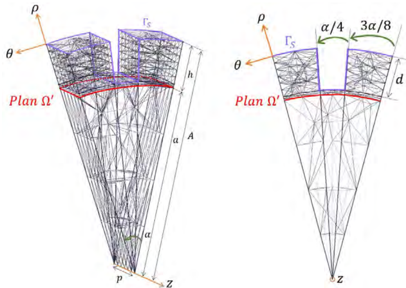
Figure 4.16 – Cellule élémentaire 3-D et son maillage avec A = 100 mm, a = 80 mm, \alpha = 30^\circ , d = 18.2 mm, h = 20 mm et p = 26.225 mm.
