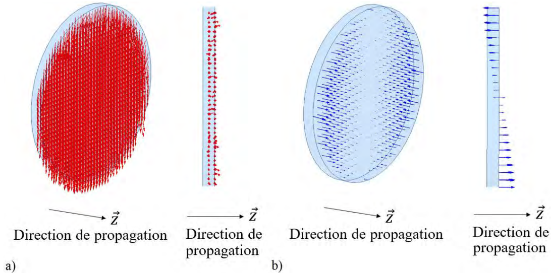
Figures 1.4 – Distributions du mode hybride EH_{11} dans un guide d'onde cylindrique à paroi isotrope Z_S = jZ_0/2 , a) champ électrique et b) champ magnétique.
