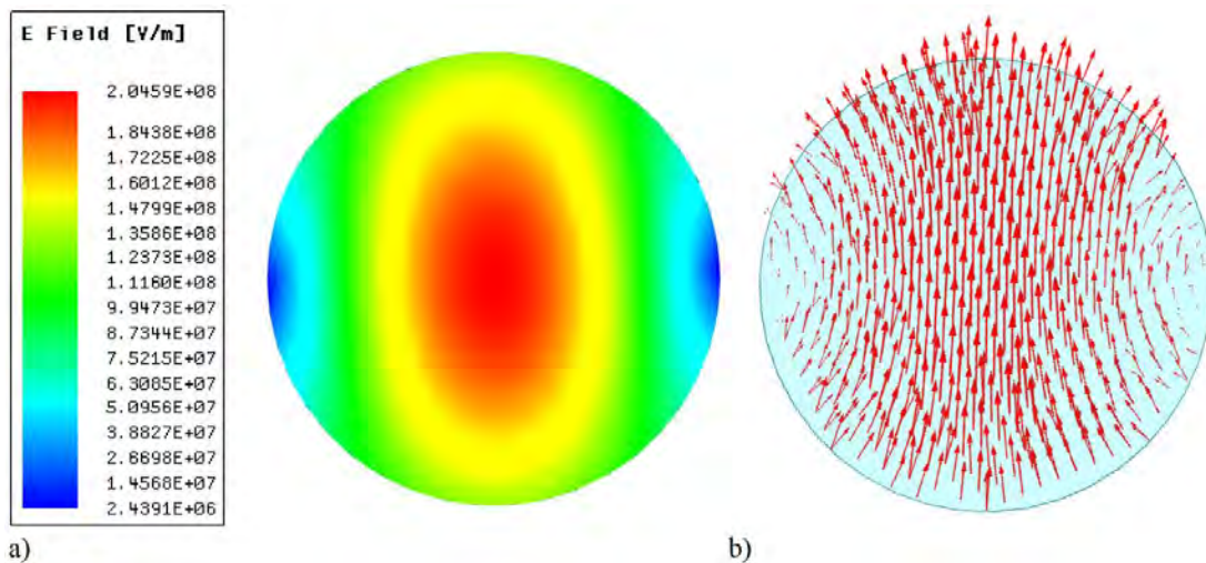
Figures 4.22 – Représentation a) en module et b) en vecteur du champ électrique du mode TE 11 dans un guide d'onde métallique.
