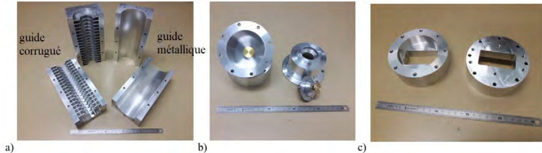
Figures 3.31 – Réalisations : a) guides corrugué et métallique par usinage, b) TGC du mode TM_{01} et c) TCR.
