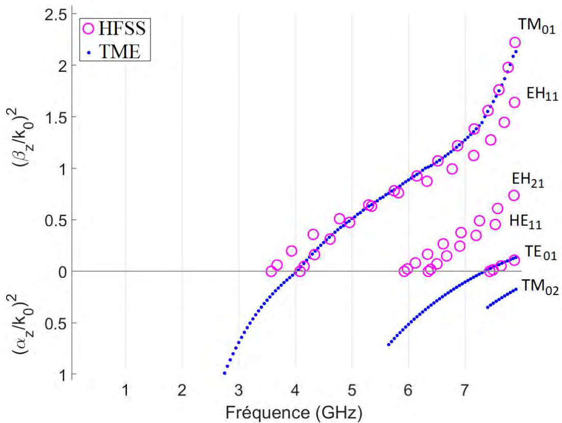
Figure 3.13 – Diagrammes de dispersion du guide de la figure 3.9 obtenus avec la TME (points bleus) et avec HFSS (cercles roses).
