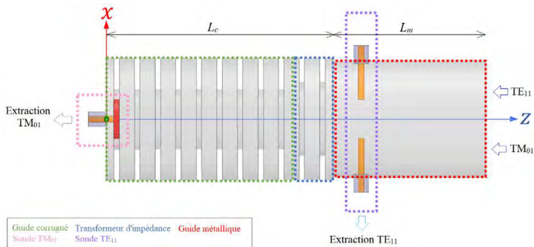
Figure 3.38 – Extracteur de modes.
