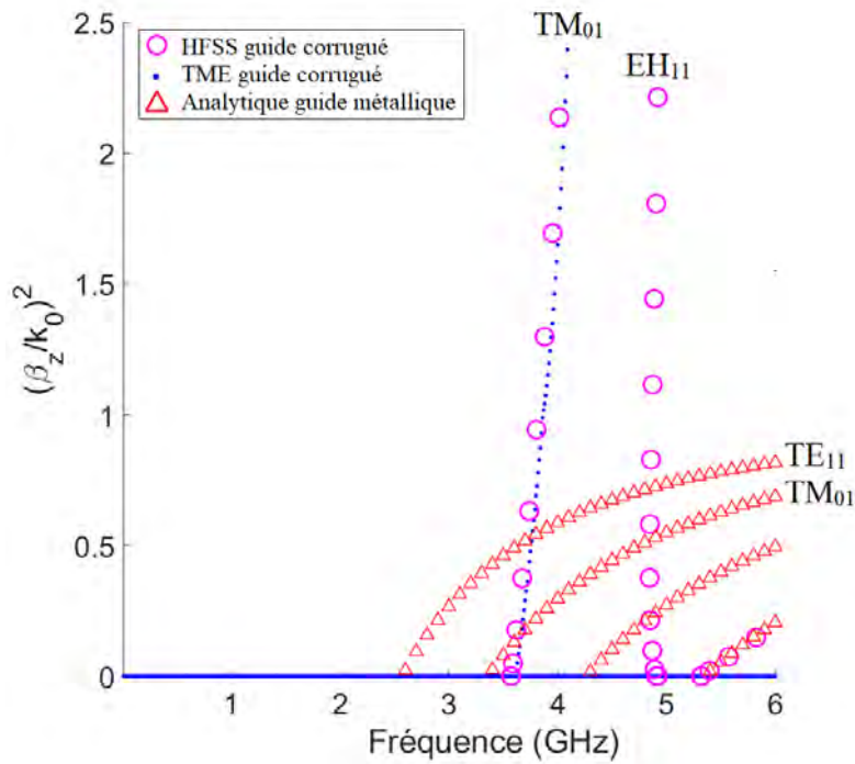
Figure 3.21 – Diagrammes de dispersion du guide métallique en rouge, et du guide corrugué (en bleu obtenu avec la TME et en rose avec HFSS).
