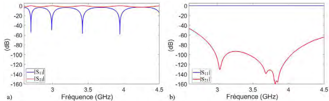
Figures 3.30 – Paramètres S des guides a) métallique et b) corrugué.
