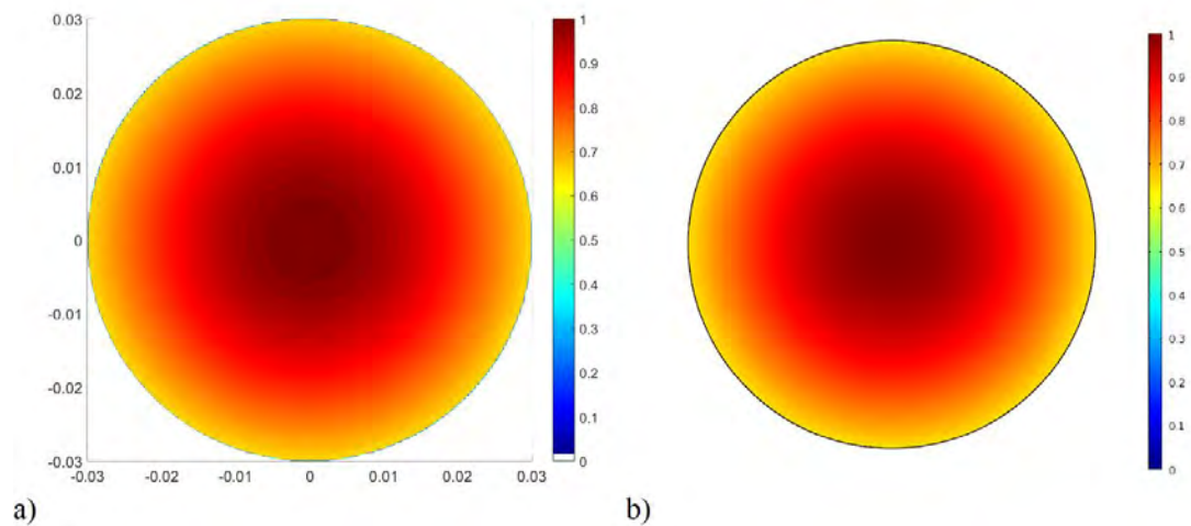
Figures 2.6 – Amplitude normalisée du champ électrique du mode TM 01 dans un guide à paroi anisotrope, à la fréquence f = 2.4 GHz avec a) TME et b) COMSOL.
