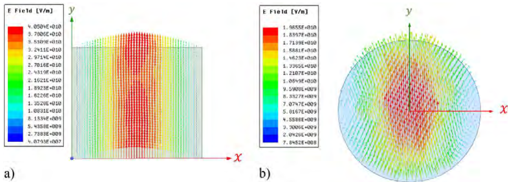
Figures 3.28 – Cartographies du champ électrique a) du mode TE_{01} dans un guide rectangulaire et b) du mode TE_{11} dans un guide cylindrique.
