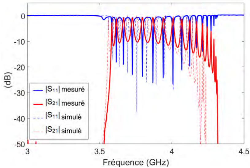
Figure 3.34 – Paramètres S du guide corrugué usiné après post traitement des mesures et comparaison avec les résultats de simulation.
