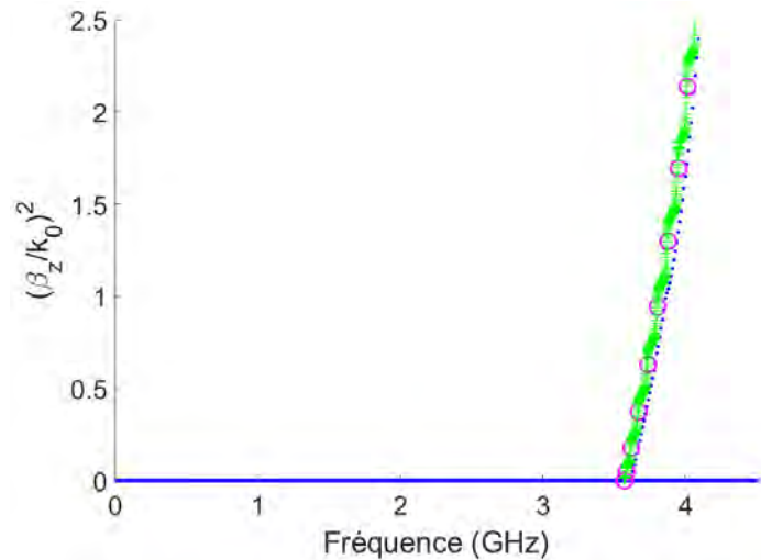
Figure 3.35 – Diagrammes de dispersion obtenu avec la TME (points bleus), avec HFSS en solver eigenmode (cercles roses) et après post traitement des mesures (croix vertes) du guide usiné.
