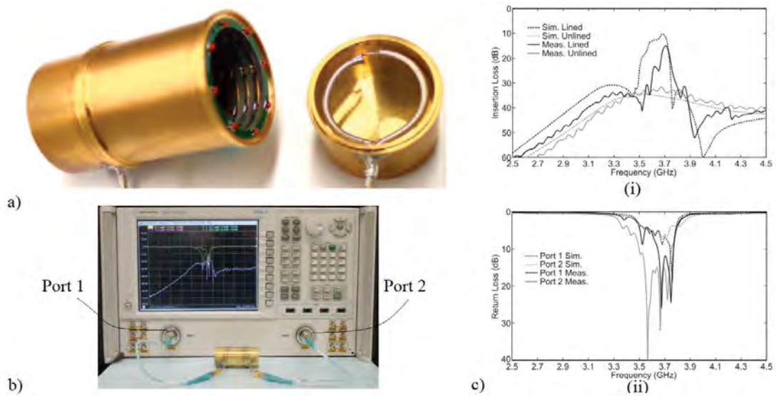
Figures 1.12 – a) Guide d’onde à métamatériau, b) dispositif de mesure et c) comparaison des paramètres de transmission (i) et réflexion (ii) mesurés et simulés [28].
