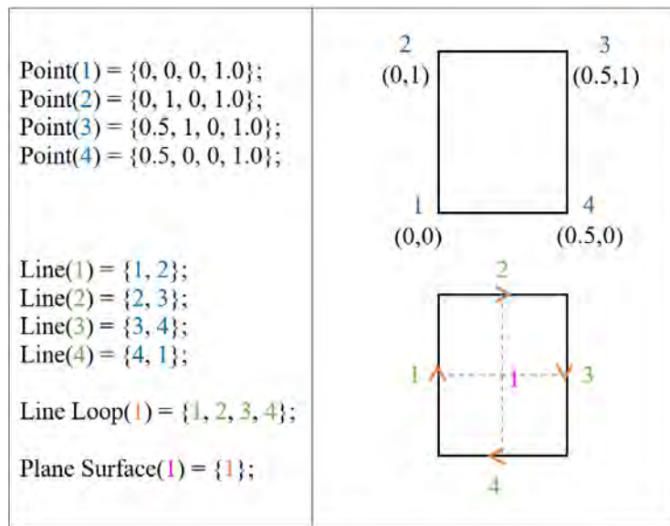
Figure G.4 – Fichier « .geo » correspondant à la figure G.3.
