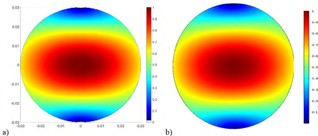
Figures 2.4 – Amplitude normalisée du champ électrique du mode TE_{11} dans un guide métallique, à la fréquence f = 3.5 GHz avec a) TME et b) COMSOL.
