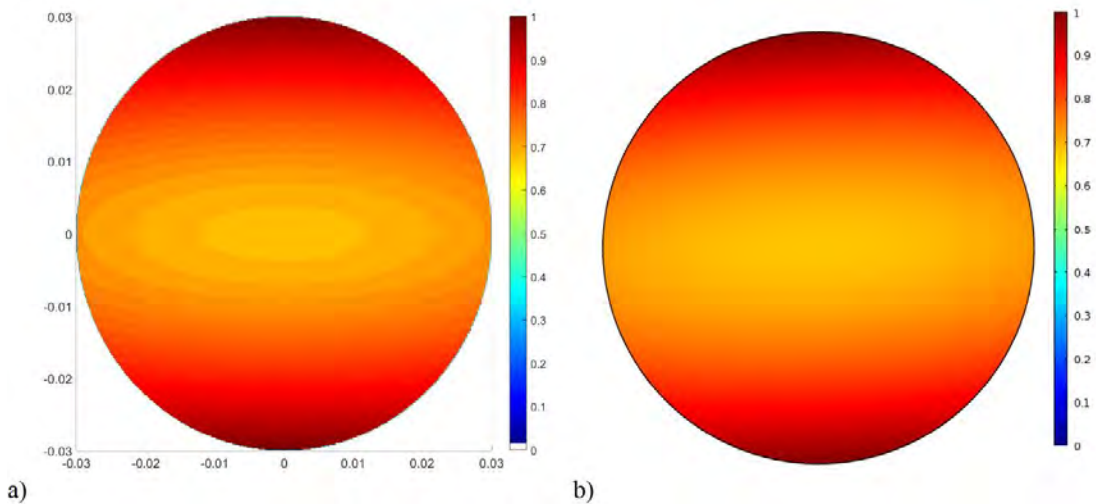
Figures 2.9 - Amplitude normalisée du champ magnétique du mode EH_{11} dans un guide à paroi anisotrope, à la fréquence f = 1 GHz avec a) TME et b) COMSOL.
