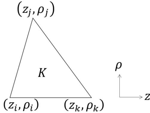
Figure E.1 – Élément du maillage : triangle K .
