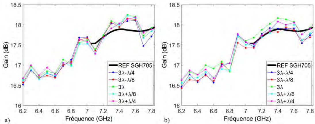
Figure 4.47 – Gain maximum de l'antenne SGH705 mesuré par les sondes a) corruguée et b) métallique pour les cinq distances.
