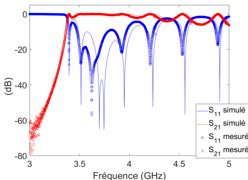
Figure I.4 – Paramètres S de l'ensemble « TGC-guide métallique-TGC » mesurés en cercle, et simulés en trait plein.
