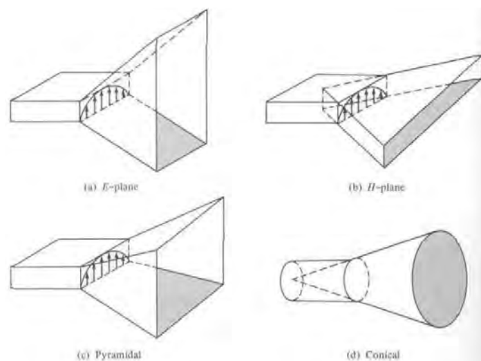
Figures 1.16 – Exemple d'antennes cornets de type a) plan E, b) plan H, c) pyramidale et d) conique [9].
