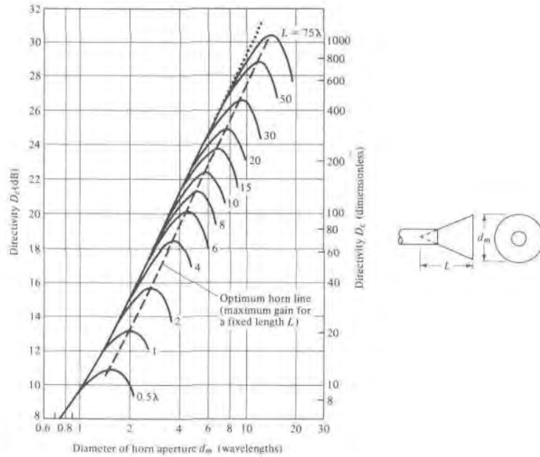
Figure 1.23 – Directivité d'un cornet E en fonction des dimensions [9].
