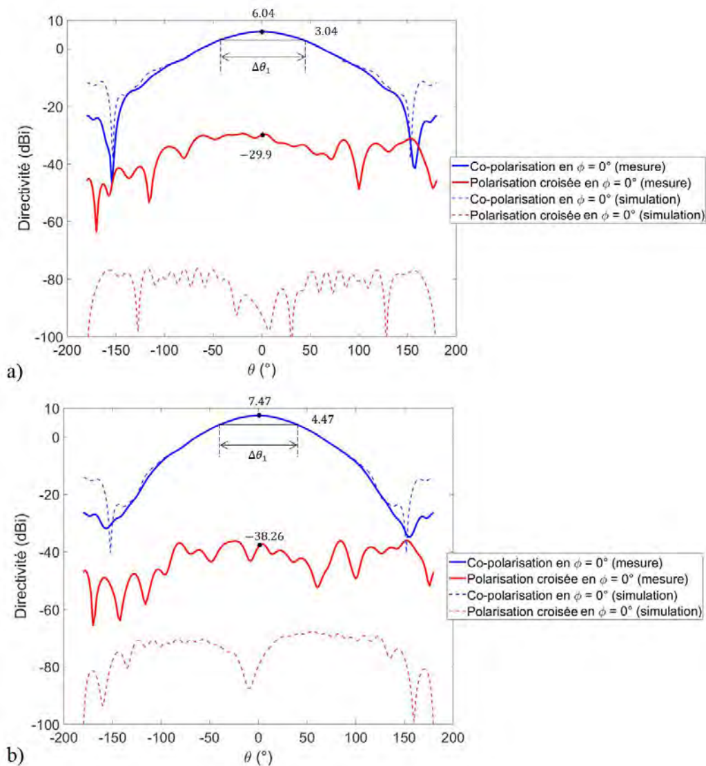
Figures 4.40 – Directivité (dBi) des sondes a) corruguée et b) métallique.
