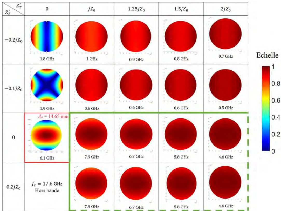
Figure 4.23 – Cartographie du champ électrique pour diverses combinaisons d'impédances.
