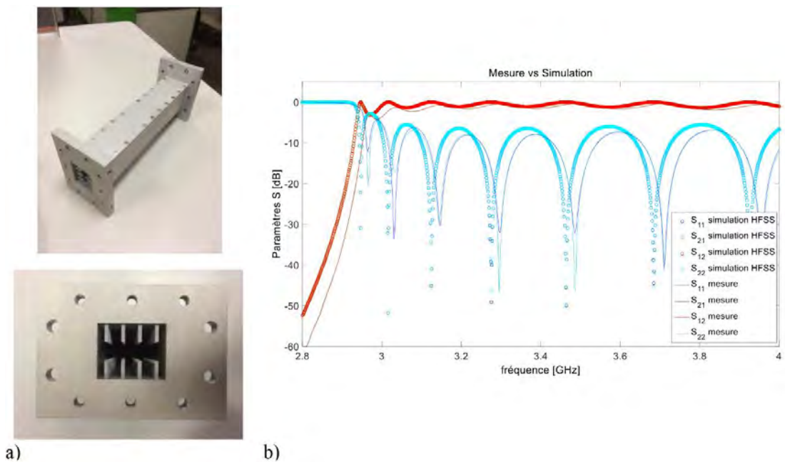
Figures 1.15 – a) Guide d'onde PIC et b) comparaison des paramètres S simulés et mesurés [25].
