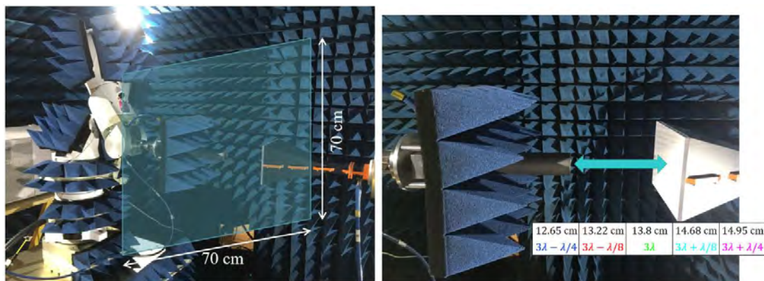
Figure 4.45 – Procédure de mesure du gain d'une antenne sous test avec les sondes.
