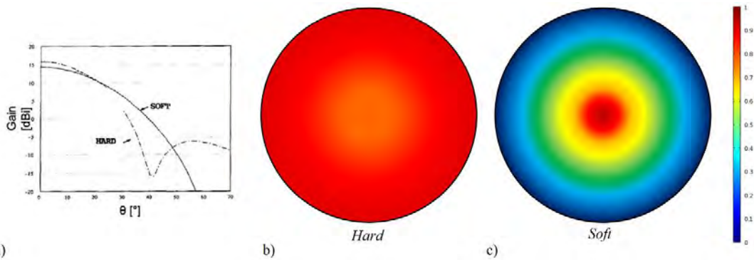
Figures 1.22 – a) Diagrammes de rayonnement de cornets soft et hard [34] et cartographies normalisées du champ électrique de cornets b) hard ou c) soft .
