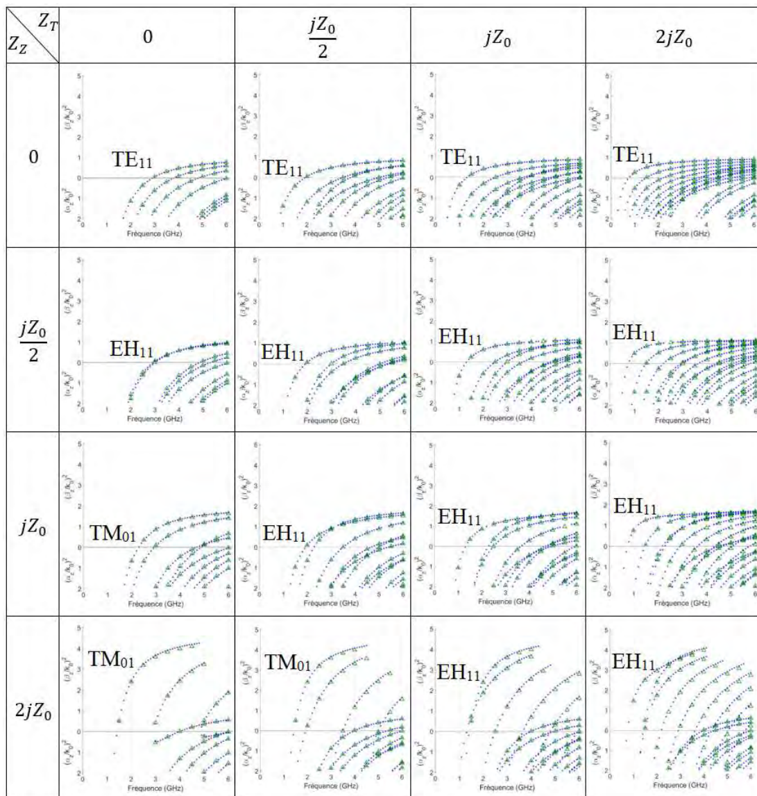
Figure 2.3 – Diagrammes de dispersion d'un guide cylindrique pour diverses combinaisons d'impédances de surface ( Z_T ; Z_Z ). Les courbes représentées avec des points bleus sont obtenues avec le code de TME et celles avec les triangles verts avec COMSOL.
