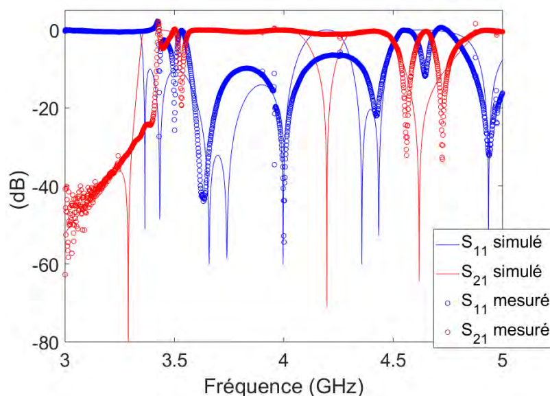
Figure I.5 – Paramètres S du guide métallique isolé après post-traitement, les mesures sont représentées par des cercles, et les simulations par des traits pleins.
