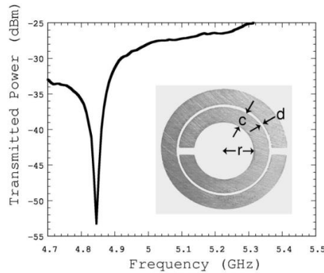
Figure 0.3 – Courbe de résonance du SRR [2].
