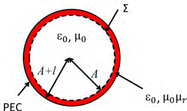
Figure C.1 – Guide d'onde utilisé sous COMSOL.
