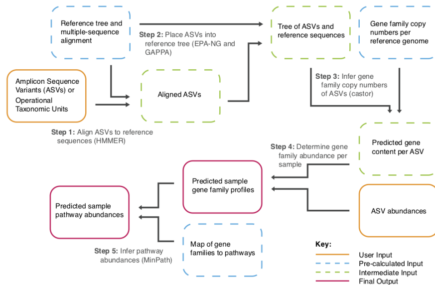
FIGURE A.XVIII – Chaîne de traitement de PICRUSt2.
