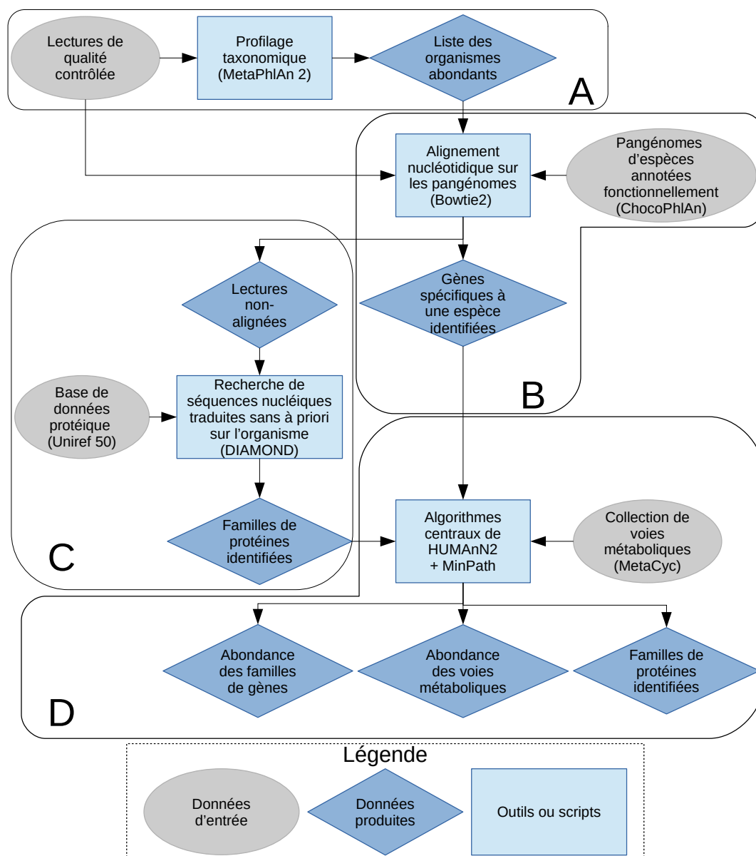
FIGURE B.XIII – HUMAnN2 pipeline. Composé de quatre modules : A : analyse phylogénétique des lectures issues de séquençage métagénomique par MetaPhlAn v2.0 ; B : alignement sur une base de données de pangénomes ; C : recherche par des séquences nucléiques traduites contre une base de données protéiques ; D : reconstruction des voies métaboliques.
