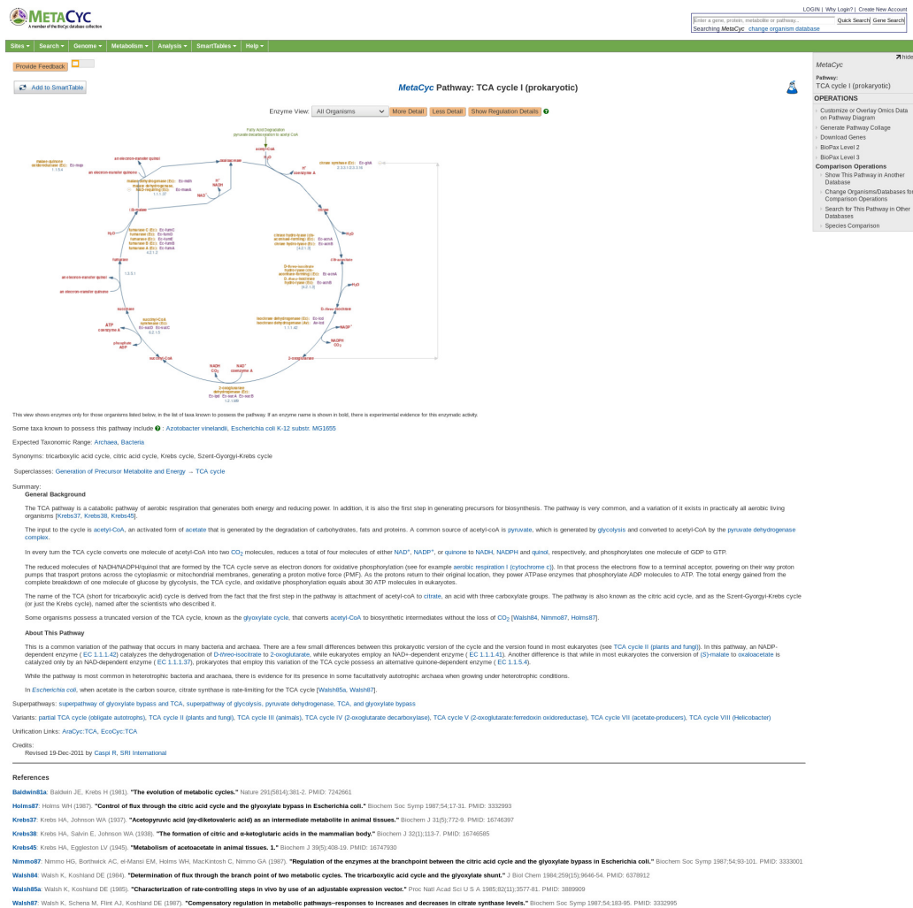
FIGURE A.XV – Fiche du cycle de Krebs ( TCA cycle en anglais) procaryote dans MetaCyc.
