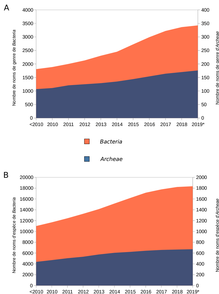
FIGURE A.VII – Évolution du nombre de noms de genres (A) et d'espèces (B) dans le NCBI Taxonomy. * : Le nombre pour 2019 a été arrêté au 30/08/2019.
