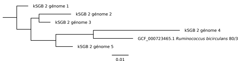
FIGURE B.III – Zoom sur la zone de l'arbre phylogénétique contenant les génomes reconstruits du groupe kSGB 2.
