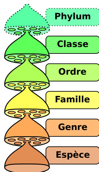
FIGURE A.VI – Rangs taxonomiques majeurs régus par le code de nomenclature des procaryotes. Les phyla sont indiqués en pointillés, car non régus à l'heure actuelle par le code, bien qu'une proposition ait été effectuée (OREN et al. 2015).
