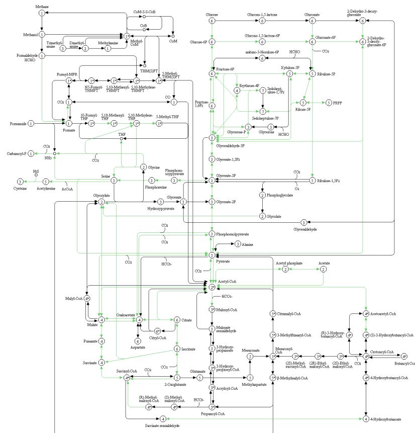
FIGURE A.XVI – Ensemble des voies du métabolisme du carbone présentes chez Escherichia coli K-12 MG1655. Les flèches vertes indiquent que le gène codant l'enzyme catalysant la réaction a été identifié et que sa séquence ainsi que la séquence d'acides aminés de l'enzyme est disponible.
