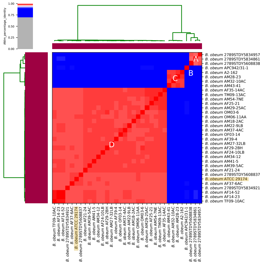
FIGURE B.VIII – Ensemble des génomes assemblés appartenant à l'espèce Blautia obeum présent dans RefSeq (n = 33) et GenBank (n = 1). Blautia obeum ATCC 29174 surlignée correspond à la souche type de l'espèce.
