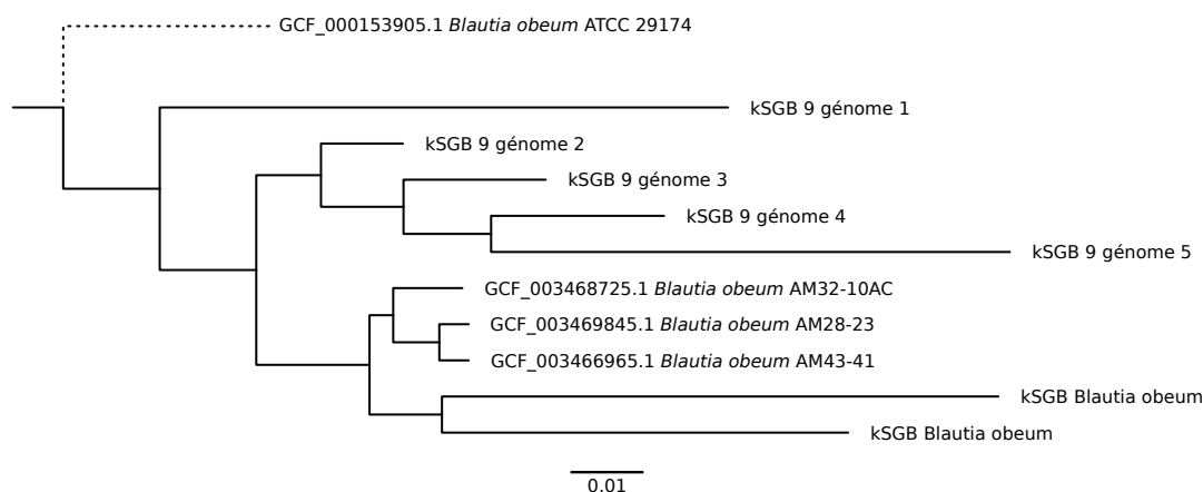
FIGURE B.IV – Zoom sur la zone du groupe kSGB 9. Les génomes notés « kSGB Blautia obeum » font partie d'une autre kSGB affiliée à Blautia obeum . Blautia obeum ATCC 29174 est le génome de la souche type de l'espèce Blautia obeum . Le point de divergence avec le génome de la souche type est indiqué en pointillés.
