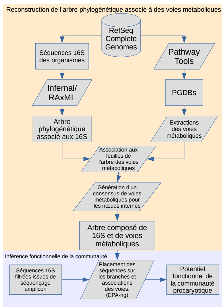
FIGURE A.XX – Chaîne de traitement de PAPRICA.
