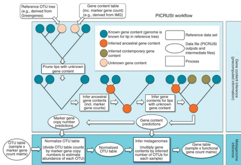
FIGURE A.XVII – Chaîne de traitement de PICRUSt.
