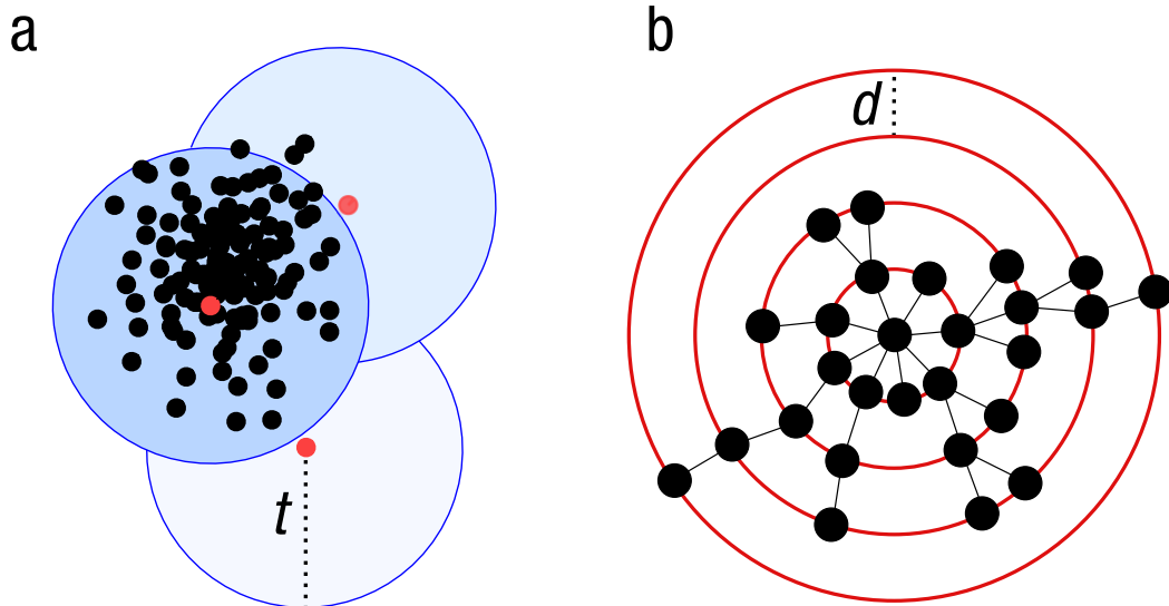
FIGURE A.X – Schéma de deux méthodes de groupement de séquences. A : par identité de séquence. Les ronds rouges sont les séquences centrales choisies au hasard pour former un groupe à t % de similarité. Bien que les différentes séquences soient proches, elles appartiennent à différents groupes. B : par essaim. Une séquence est choisie au hasard et toutes les séquences avec d nucléotides de différence sont ajoutées aux groupes. Une fois cette opération réalisée, elle est répétée pour les séquences ajoutées. Toutes les séquences appartiennent ici à la même OTU.
