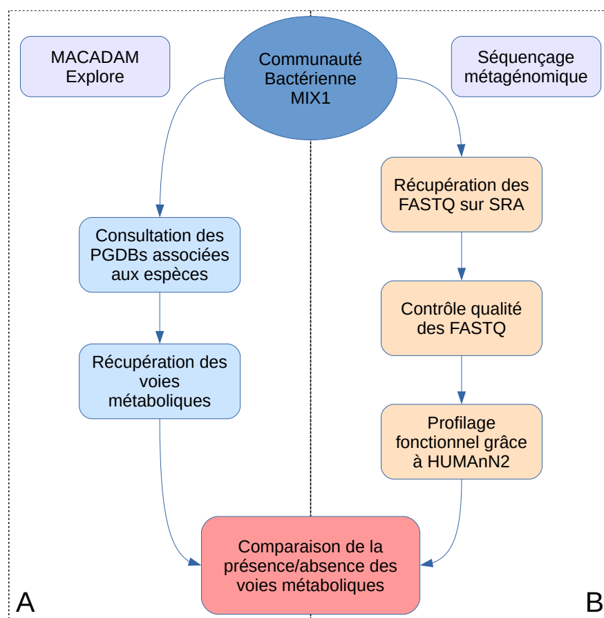
FIGURE B.XII – Schéma des deux chaînes de traitement d'analyse permettant la comparaison des voies métaboliques présentes : A : MACADAM Explore ; B : Séquençage métagénomique en utilisant HUMANN2.
