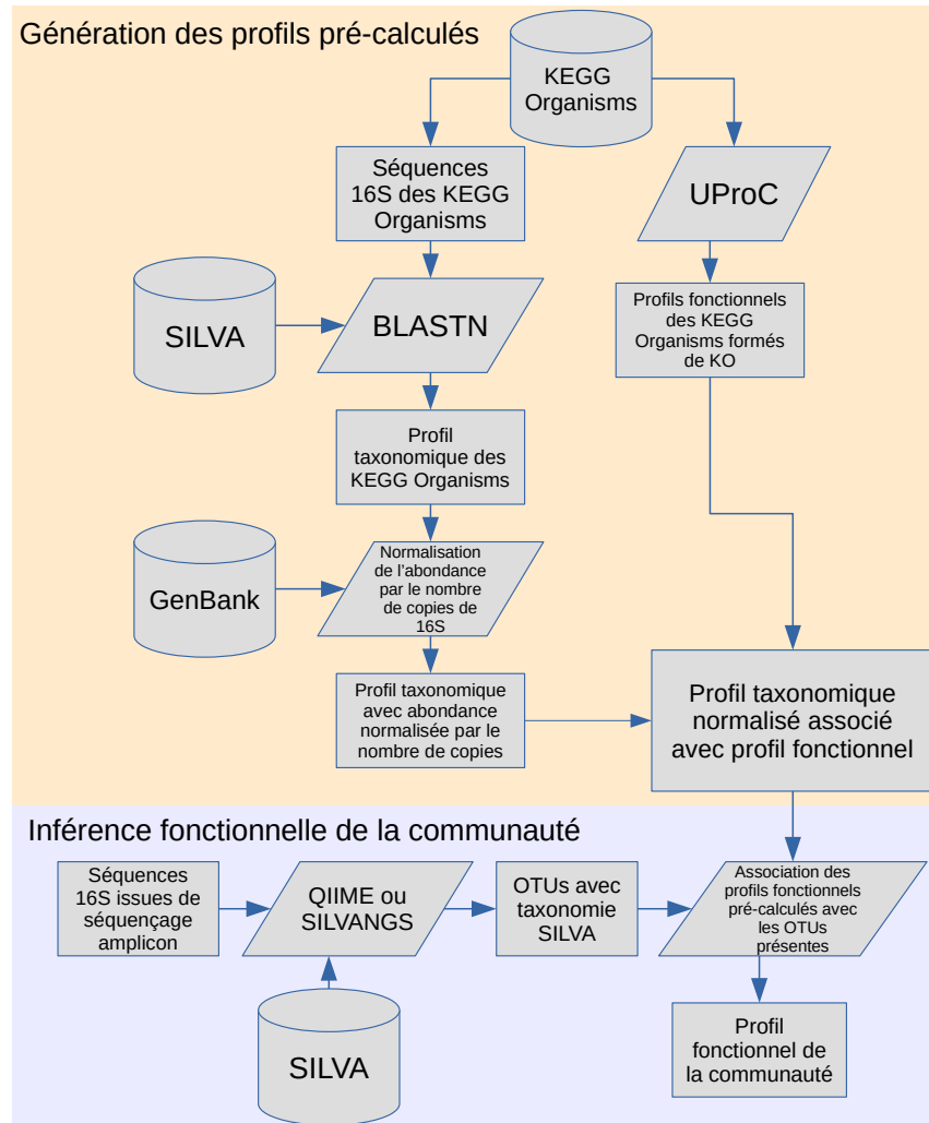
FIGURE A.XIX – Chaîne de traitement de Tax4Fun.
