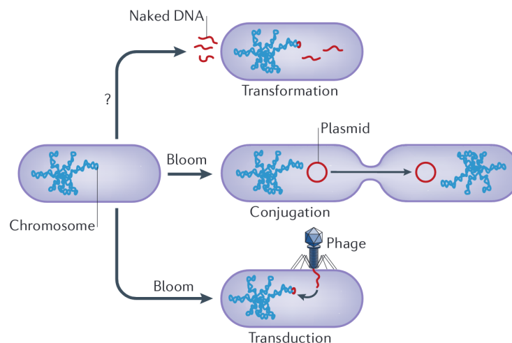
FIGURE A.II – Mécanismes de transferts horizontaux de gènes chez les bactéries.
