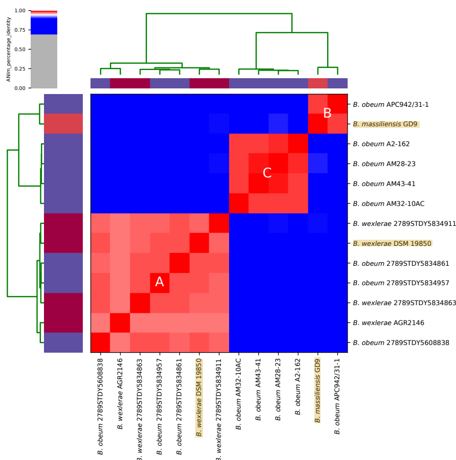
FIGURE B.IX – Ensemble des génomes assemblés appartenant aux espèces Blautia obeum , Blautia wexlerae ( n = 4 ) et Blautia massiliensis ( n = 1 ) présents dans RefSeq. Les génomes de B. obeum proviennent des trois groupes A, B et C de la figure B.VIII.
