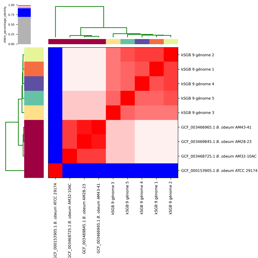
FIGURE B.VII – Représentation de l’ANIm calculé entre les 5 génomes choisis aléatoirement du groupe kSGB 9 et une sélection de génomes assemblés affiliés à Blautia obeum présent dans RefSeq. Blautia obeum ATCC 29174 est la souche type de l’espèce.
