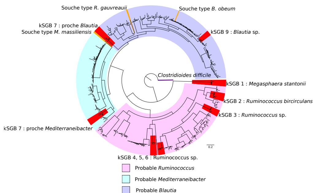
FIGURE C.I – Arbre phylogénétique résumant les résultats mis en évidence dans la partie B.1, page 79.
