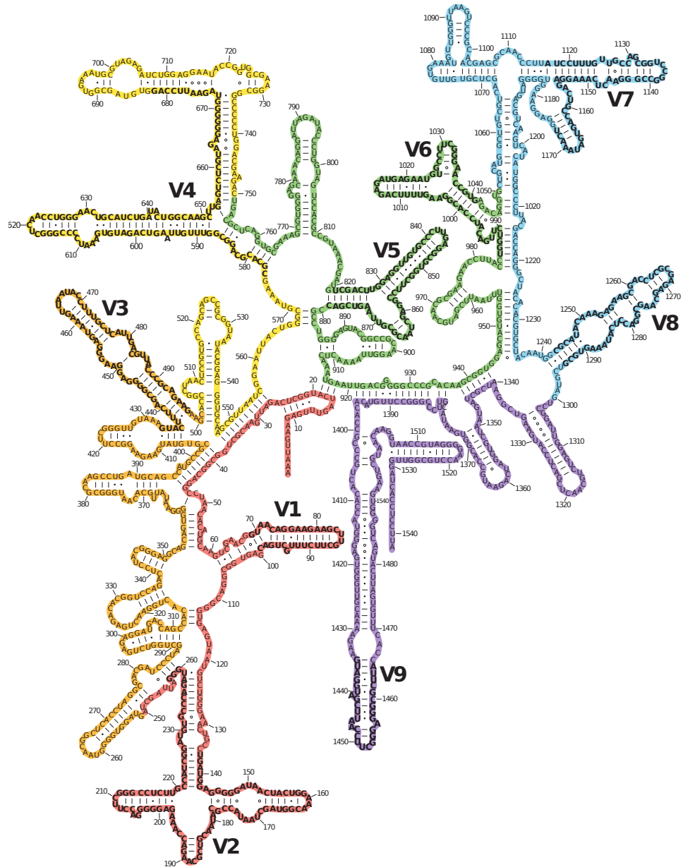
FIGURE A.III – Structure secondaire de l'ARNr 16S chez Escherichia coli composée de 1541 nucléotides (BROSIOUS et al. 1978). Les régions variables sont indiquées par leur nom (V1 par exemple), et les nucléotides les composant sont indiqués en gras.
