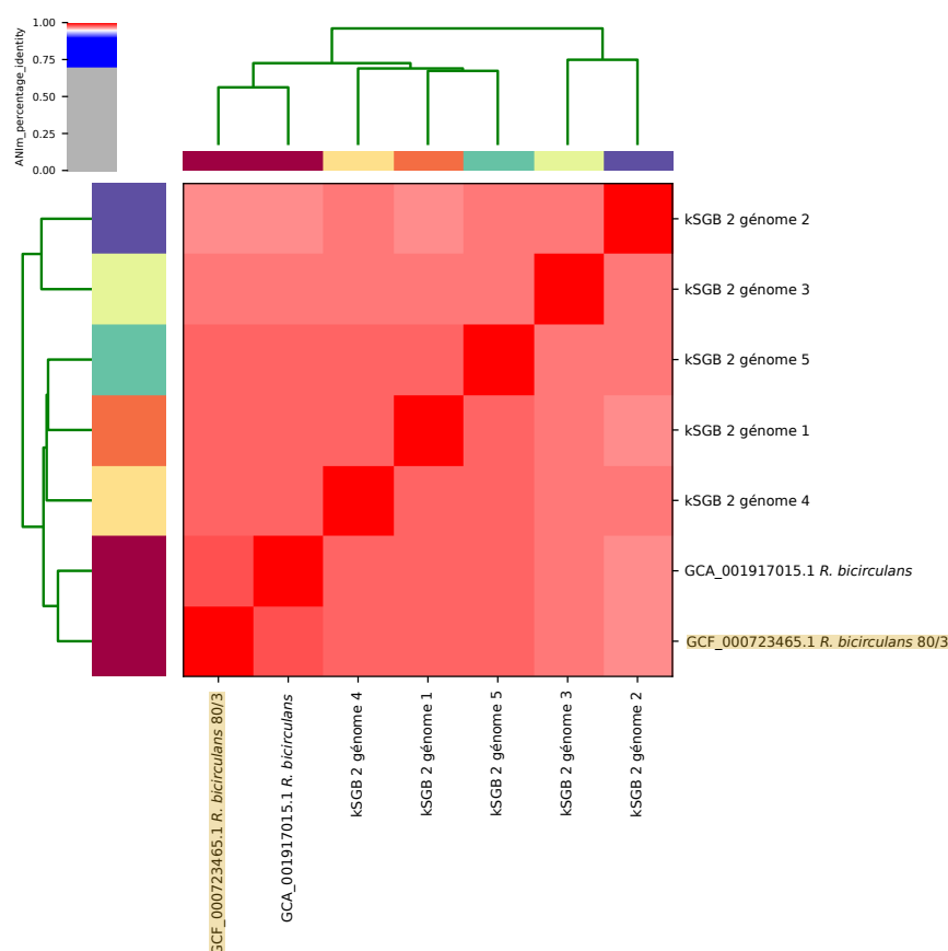
FIGURE B.VI – Représentation de l'ANIm calculé entre les 5 génomes choisis aléatoirement dans le groupe kSGB 2, les 2 génomes RefSeq et les 2 génomes GenBank de Ruminococcus bicirculans . Ruminococcus bicirculans 80/3 est la souche type de l'espèce.
