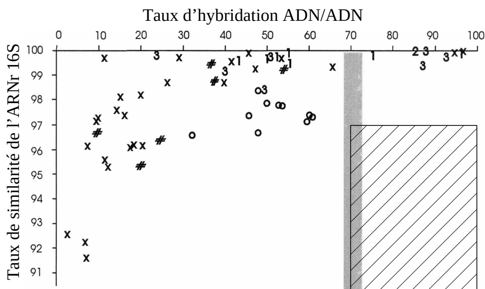
FIGURE A.IV – Comparaison du taux de similarité de l'ARNr 16S et du taux d'hybridation ADN/ADN dans une sélection d'organismes provenant de différents jeux de données. Chaque symbole indique un jeu de données différent où l'hybridation ADN/ADN à été effectué via différentes méthodes : x, méthode par filtration membranaire ; #, 1, 2, 3 et 4, méthode par taux de renaturation ; o , méthode de la nucléase S1. La zone hachurée (moins de 97% de similarité entre les ARNr 16S et plus de 70% d'hybridation ADN/ADN) ne contient aucun couple d'organismes.
