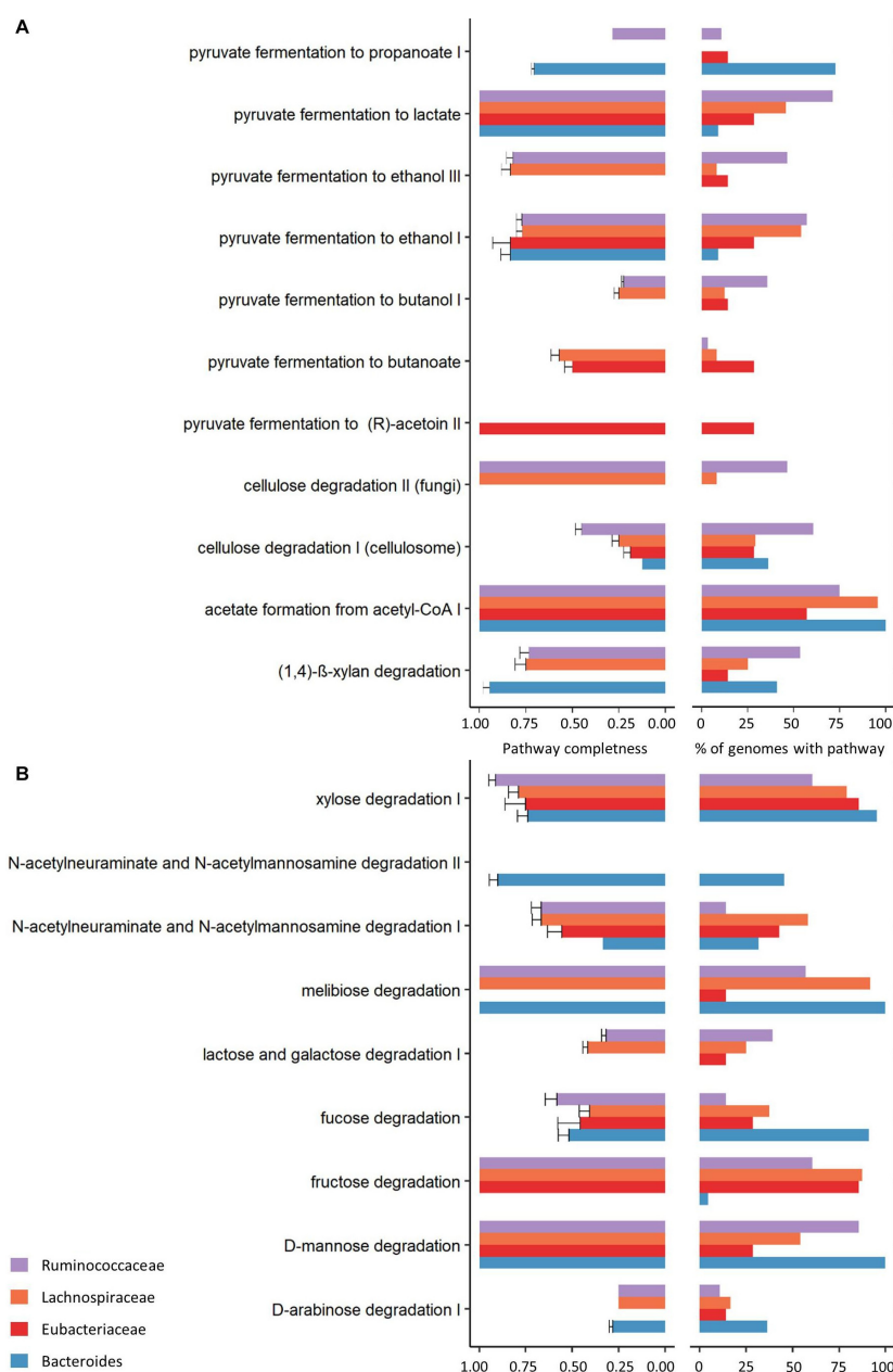
FIGURE B.X – Complétude et pourcentage d'organismes où les voies métaboliques de dégradation ou fermentation de polymères ( A ) ou de dégradation des glucides ( B ) sont présentes, chez les Lachnospiraceae , Ruminococcaceae , Eubacteriaceae et Bacteroides . Un score de 1 indique que l'ensemble des réactions composant la voie métabolique est présent dans l'organisme. Un score de zéro indique qu'aucune réaction n'est présente.
