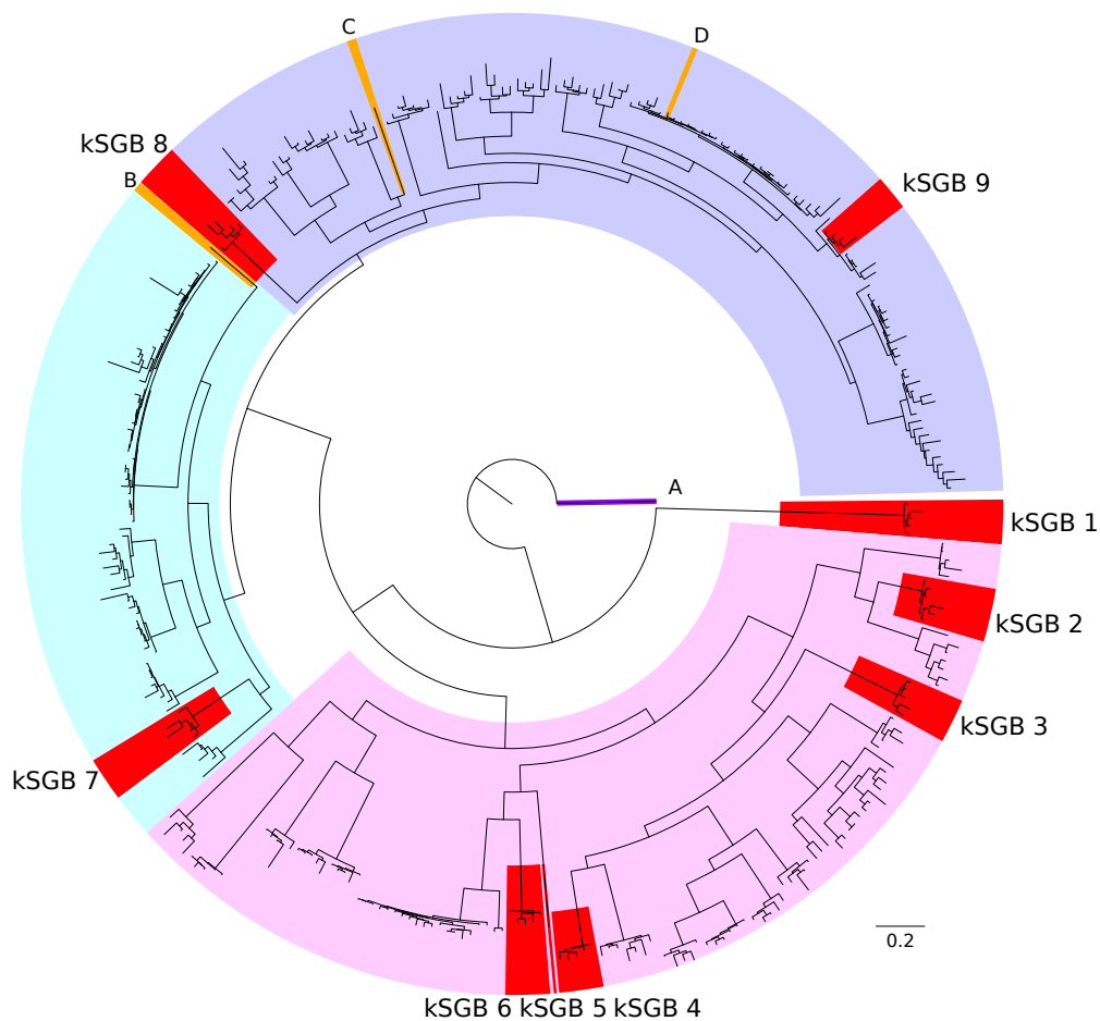
FIGURE B.II – Arbre phylogénétique se basant sur les cinq génomes reconstruits sélectionnés aléatoirement de chacun des 43 kSGBs identifiés comme appartenant au genre Blautia et Ruminococcus ainsi que les 50 et 89 génomes RefSeq pour les genres Blautia et Ruminococcus , respectivement.
