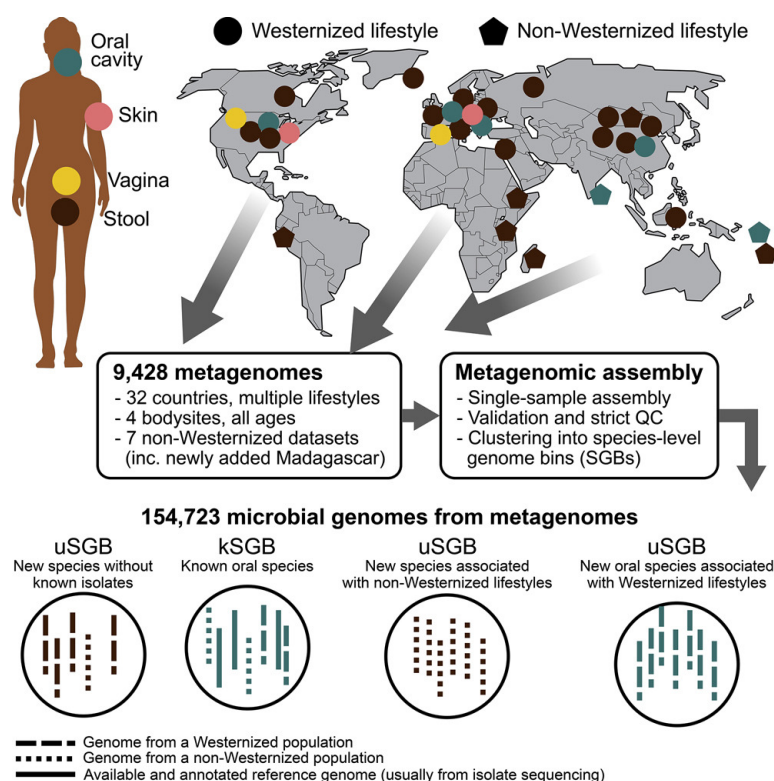
FIGURE B.I – Résumé graphique de l'étude PASOLLI et al. (2019). Ce schéma indique la nature des prélèvements et leurs origines géographiques.
