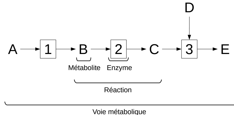
FIGURE A.XI – Les acteurs du métabolisme. Les lettres représentent des métabolites tandis que les chiffres représentent des enzymes. L'ensemble métabolite(s) d'entrée (substrat(s), B ), enzyme ( 2 ) et métabolite(s) de sortie (produit(s), C ) est appelé réaction. Une suite de réactions forme une voie métabolique.
