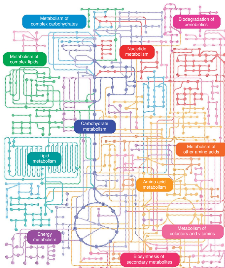
FIGURE A.XIV – Schéma du réseau métabolique de Escherichia coli .
