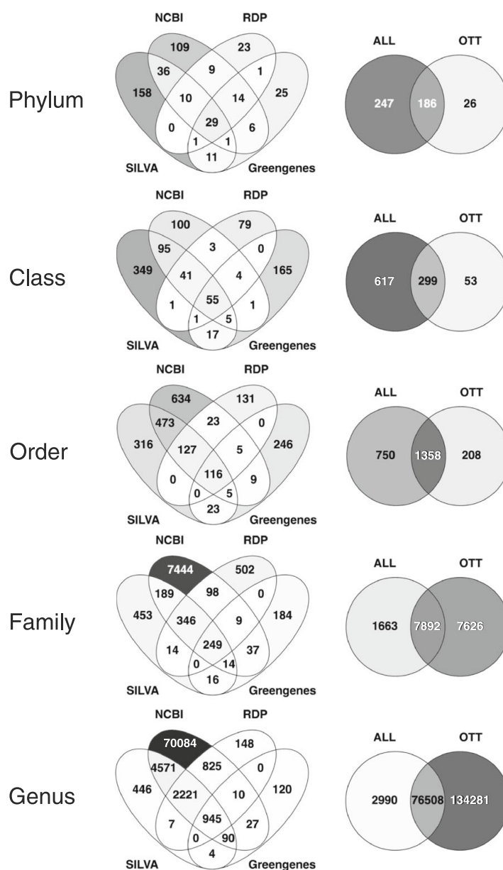
FIGURE A.VIII – Diagrammes de Venn de l'intégralité des noms de taxons (formels et informels) présents dans une ou plusieurs bases de données taxonomiques. Les diagrammes de gauche présentent, pour chaque rang taxonomique, les noms présents dans NCBI Taxonomy, Greengenes, SILVA et RDP. Le diagramme de droite présente l'union des taxonomies précédentes contre OTT. Les nuances de gris indiquent le pourcentage de noms taxonomiques contenus dans l'intersection.
