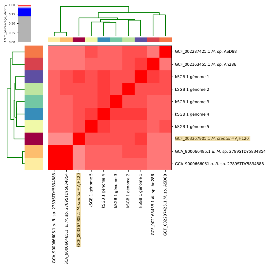
FIGURE B.V – Représentation de l'ANIm calculé entre les 5 génomes choisis aléatoirement dans le groupe kSGB 1 et les 4 génomes RefSeq et GenBank associés au groupe kSGB 1 ainsi que le génome de la souche type de l'espèce Megasphaera stantonii : Megasphaera stantonii AJH120.
