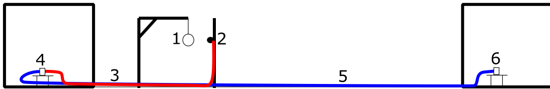
Figure 3-3: Disposition des différents éléments nécessaires pour une mesure de surpression aérienne à symétrie sphérique et en champ libre avec le standard IEPE.
