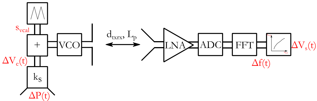
Figure 4-21: Architecture de l'émetteur RF avec calibration pour la mesure de pression sans fil.
