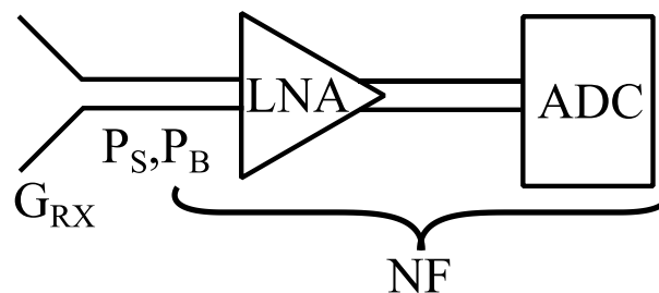
Figure 4-5: Architecture du récepteur
