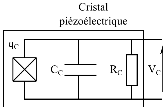
Figure 3-1: Schéma électrique d'un cristal piézoélectrique
