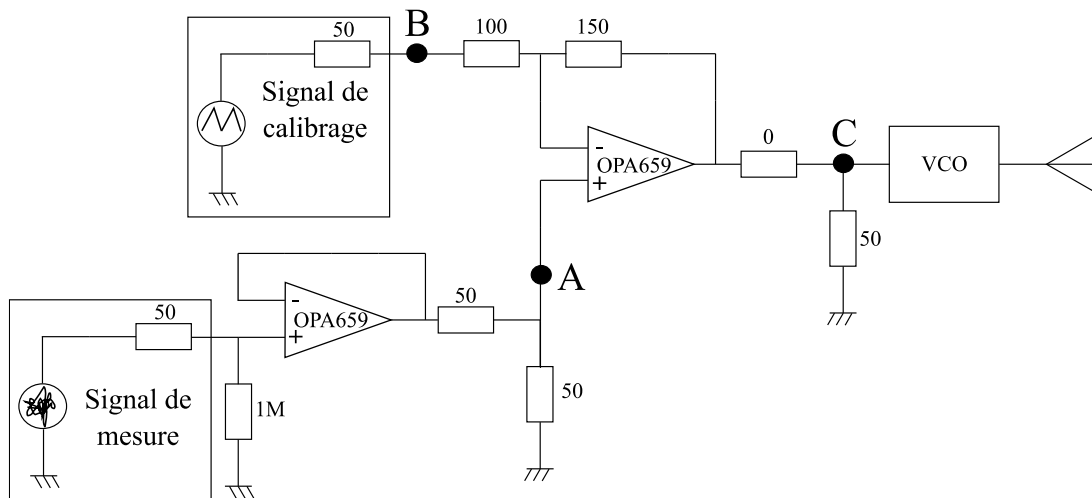
Figure 5-2: Circuit de l'émetteur du système sans fil. Montage n°2.
