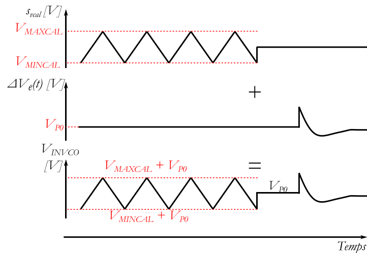
Figure 4-20: Somme des signaux de calibrage et de mesure à l'entrée du VCO.
