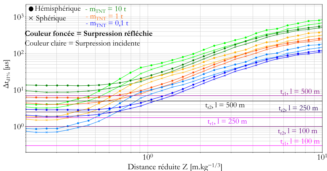
Figure 3-23: Comparaison \Delta t_{d1\%} avec t_{r1} et t_{r2} , lorsque m_{TNT} > 100 \text{ kg} .
