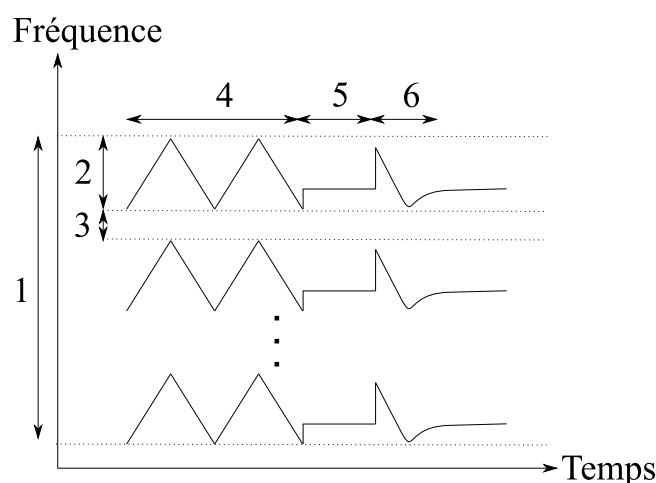
Figure 4-25: Schéma de principe du multi-capteurs avec la technique FDMA.
