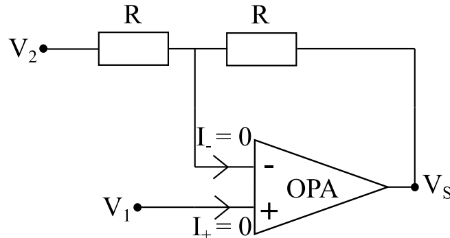
Figure 4-22: Montage classique à amplificateur opérationnel type soustracteur.
