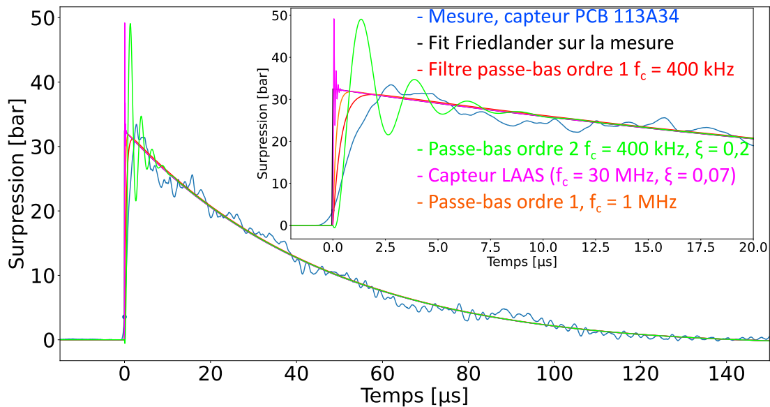
Figure 2-2: Comparaison de signaux de Friedlander théoriques avec une mesure de pression d'onde de souffle.
