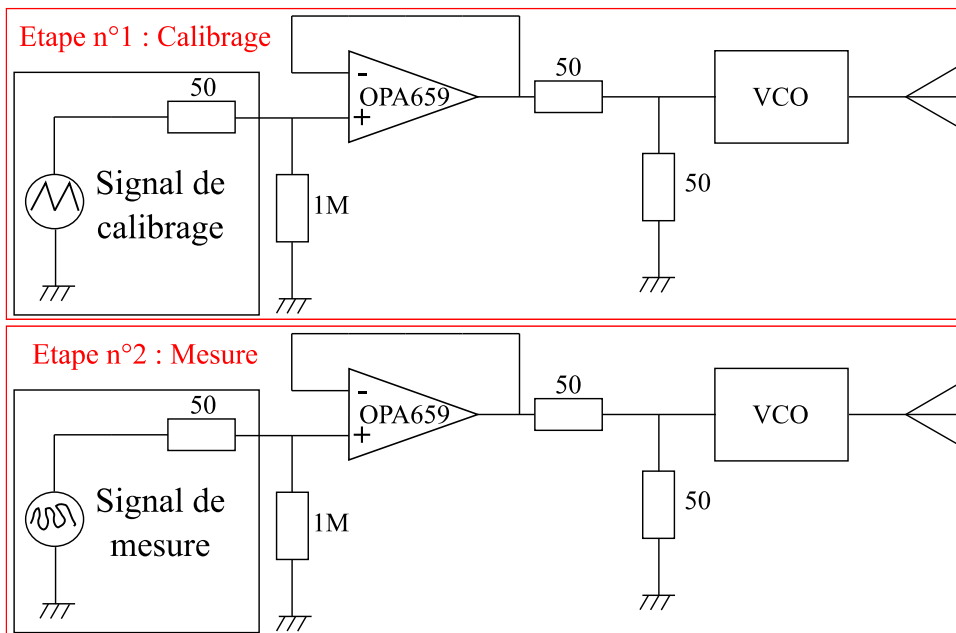
Figure 5-1: Circuit de l'émetteur du système sans fil. Montage n°1.
