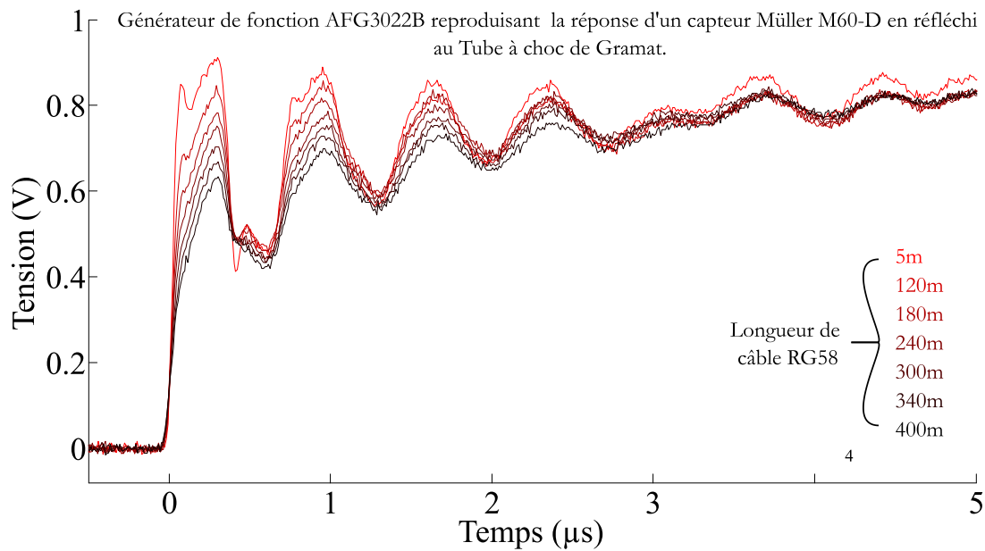
Figure 3-19: Acheminement avec plusieurs longueurs de câbles RG58 d'un signal de pression rapide reproduit avec un générateur de fonction.
