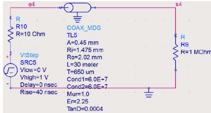
Figure 3-20: Circuit utilisé pour la simulation de la Figure 32.
