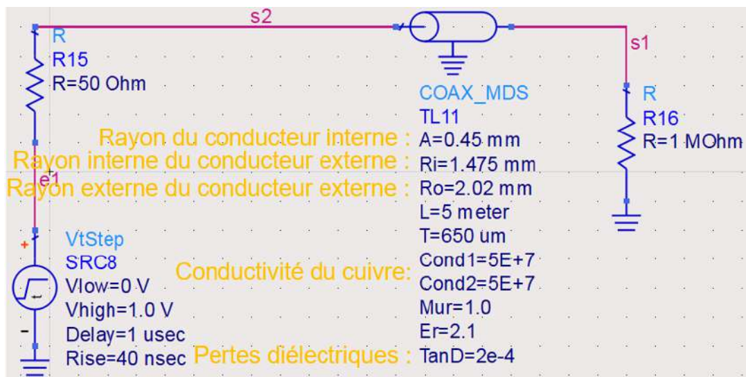
Figure 3-13: Schéma du circuit simulé avec ADS. Les caractéristiques du câble sont explicitées sur la Figure 3-14.
