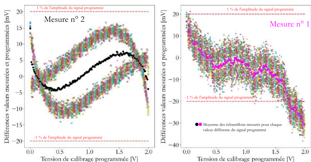
Figure 5-6: Différences entre la valeur programmée et la valeur mesurée, en fonction de la valeur programmée.
