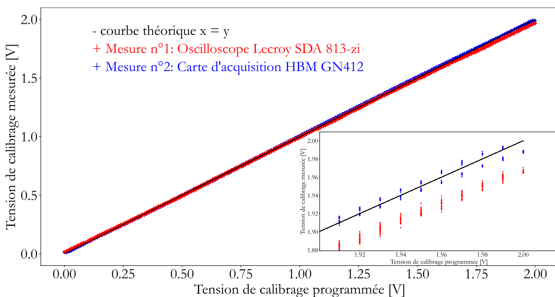
Figure 5-5: Tracé du signal triangulaire mesuré à l'oscilloscope en fonction du signal programmé dans le générateur. Montage électrique en Figure 5-4.
