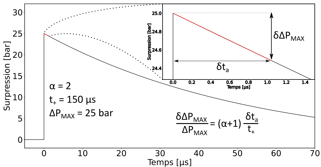
Figure 1-9: Erreur effectuée sur la surpression crête en fonction de l'erreur sur le temps d'arrivée.
