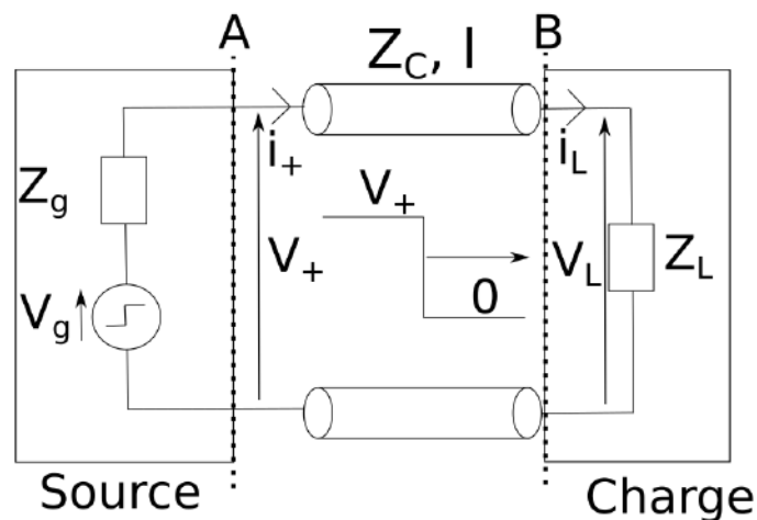
Figure B-3 : Propagation de l'onde incidente aux premiers instants après l'application du signal à l'entrée de la ligne.
