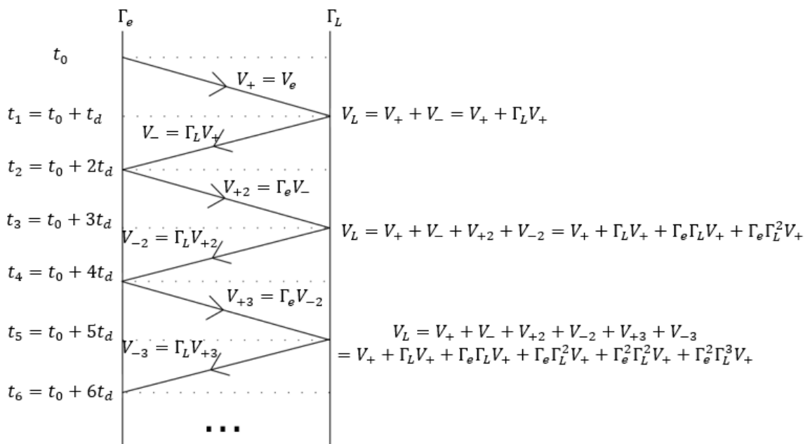
Figure B-4: Diagramme de Bounce d'une ligne de transmission désadaptée en entrée et en sortie.
