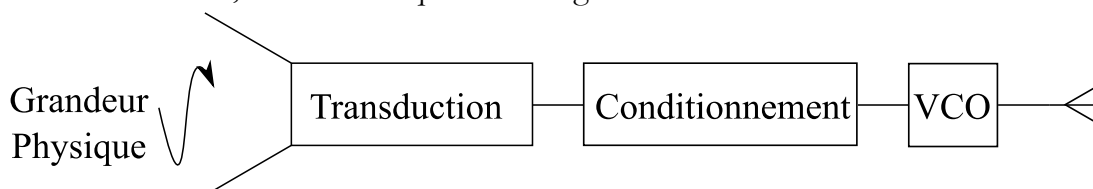
Figure 4-2: Architecture la plus simple possible d'un émetteur RF destiné à la transmission sans fil d'un signal de mesure analogique.
