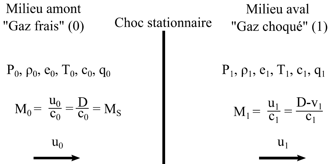
Figure 1-2: Onde de souffle après changement de référentiel pour se retrouver dans un cas similaire à la Figure 1-1
