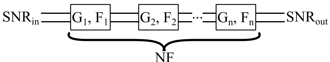
Figure 4-6: Plusieurs composants de gain G_i et de figure de bruit F_i . Figure de bruit de l'ensemble NF .
