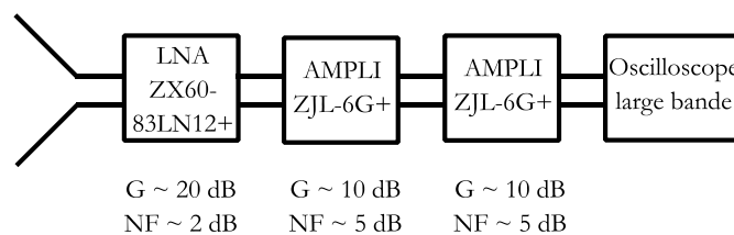
Figure 5-3: Montage électrique du récepteur du système sans fil.
