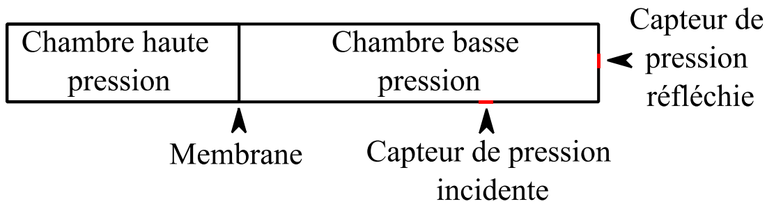
Figure 3-16: Schéma de principe d'un tube à choc à membrane.
