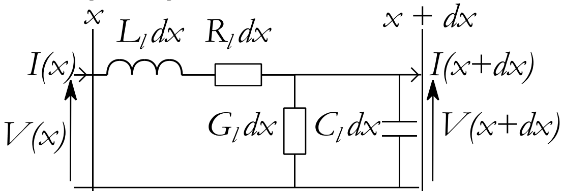
Figure 3-5: Modèle électrique à éléments distribués d'une portion infinitésimale dx de la ligne.
