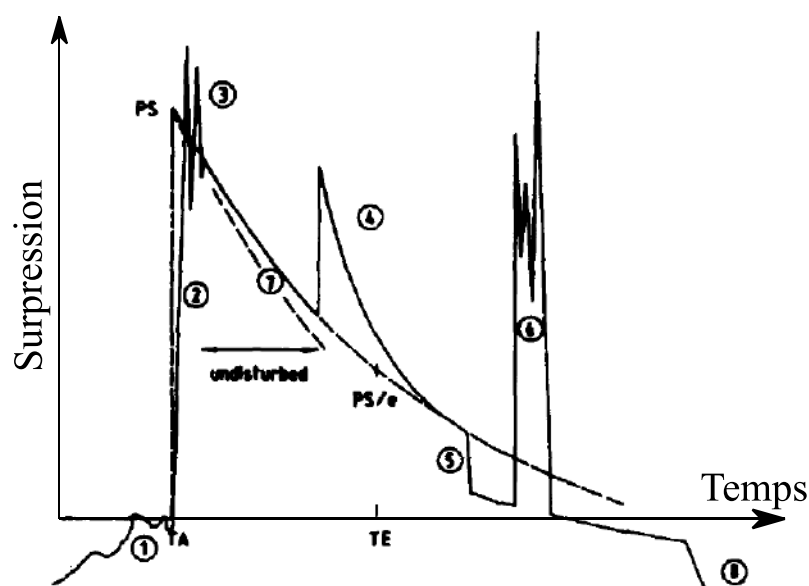
Figure 1-7: Ensemble des perturbations possibles sur une acquisition de mesure de surpression d'une onde de souffle [65].
