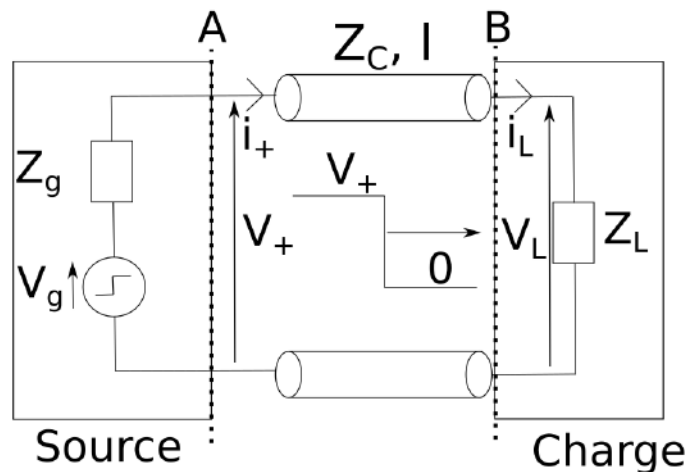
Figure B-3 : Propagation de l'onde incidente aux premiers instants après l'application du signal à l'entrée de la ligne.
