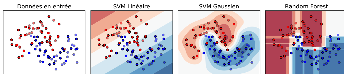
FIGURE 1.17 – Exemple de la séparation de deux classes selon les algorithmes SVM et RF. Inspiré du code de Gaël Varoquaux et Andreas Müller.
