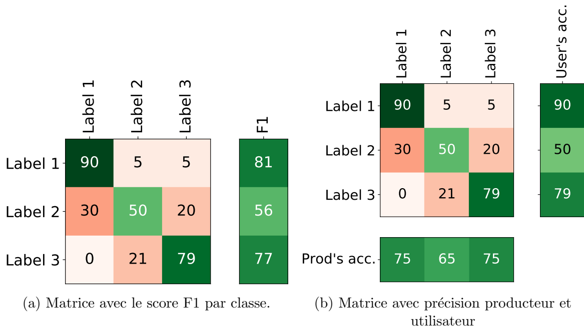
FIGURE 5.6 – Les différents types de matrices de confusion améliorées réalisées avec la classe PlotConfusionMatrix de Museo ToolBox. Ces figures ont été écrites en utilisant le Code 5.7
