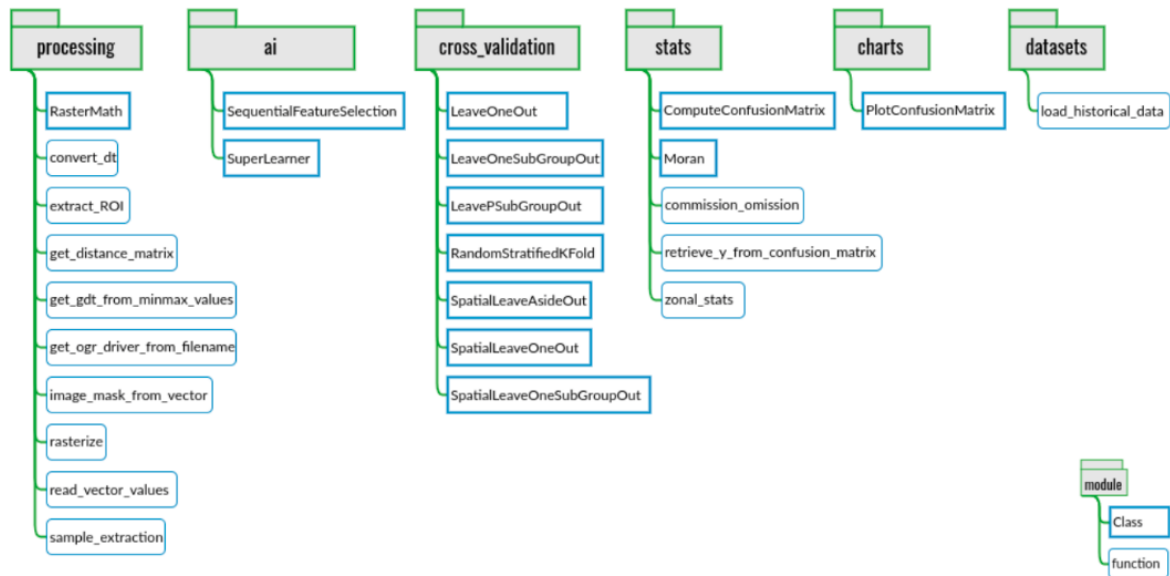
FIGURE 5.3 – Organisation générale de la bibliothèque Museo ToolBox. Plusieurs modules centralisent des traitements par thématique.
