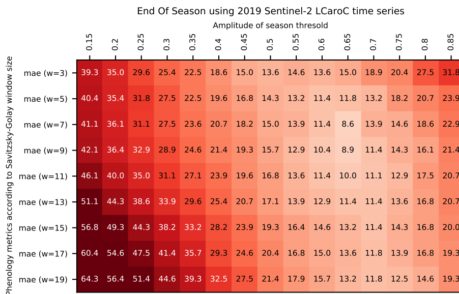
FIGURE C.18 – Erreur moyenne absolue (MAE) pour la fin de saison (BBCH=91) en fonction de la taille du filtre de Savitzky-Golay et du pourcentage de l’amplitude du LCaroC.
