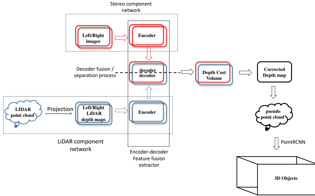
FIGURE B.4: Structure globale du réseau de neurones SLS-Fusion.
