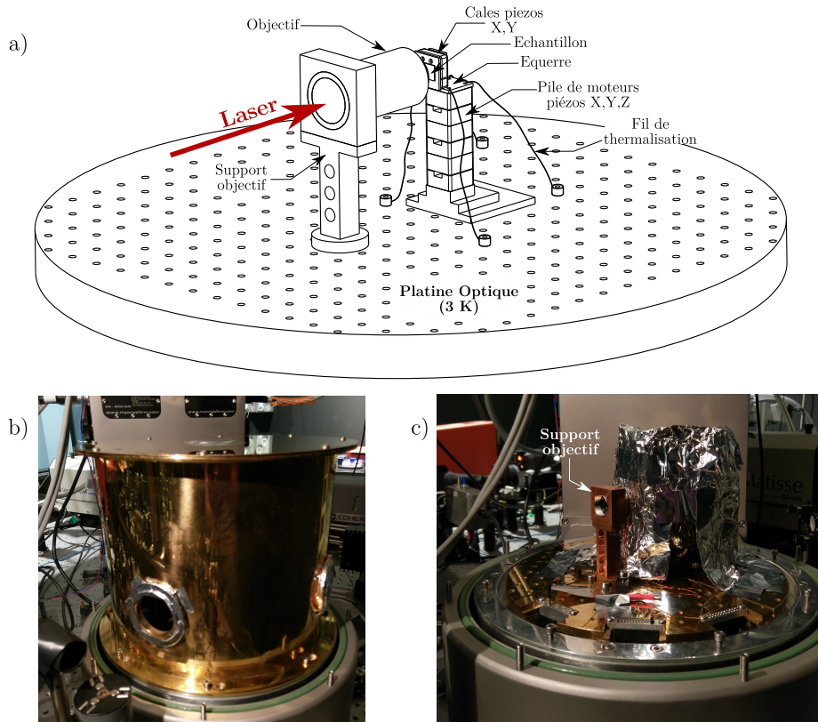
FIGURE 2.17 – Montage cryogénique. a) Schéma du montage de l'échantillon et de l'objectif sur la platine optique du cryostat ; b) Photographie de la platine optique avec l'écran thermique principal ; c) Avec l'écran thermique additionnel.
