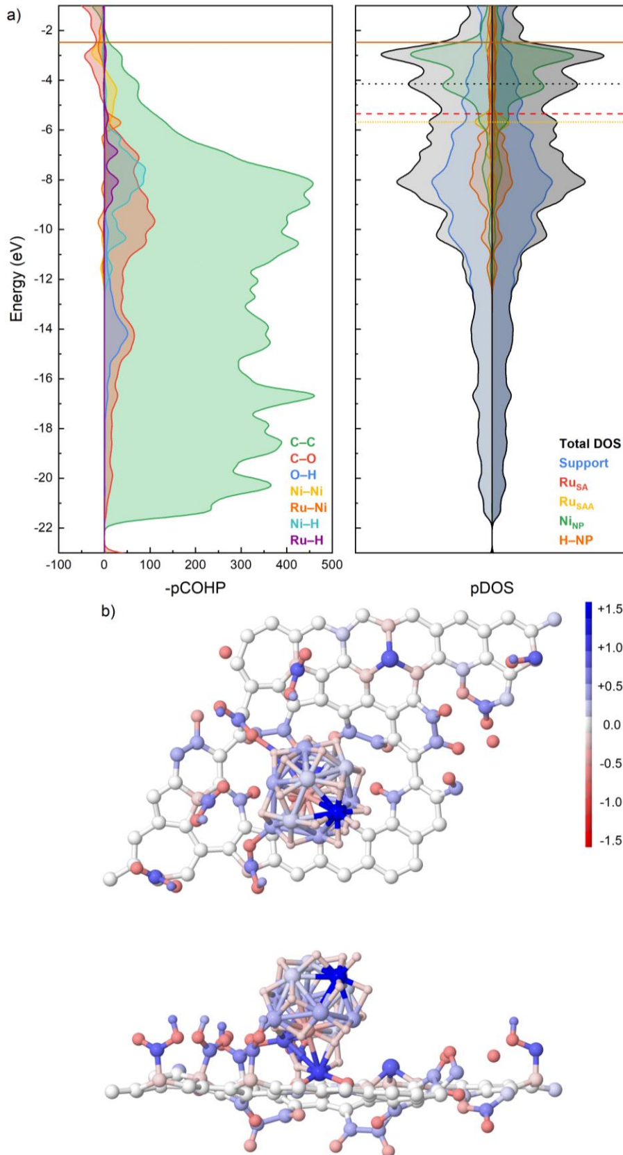
Figure 35 : Caractérisation du modèle de catalyseur SAA Ru_{SA}Ni_{NP} "Ni146" le plus stable (voir Figure 33). (a) Profils DOS et COHP projetés pour les interactions entre les plus proches voisins. (b) Vues de dessus et latérale des charges atomiques projetées de l'AMP.
