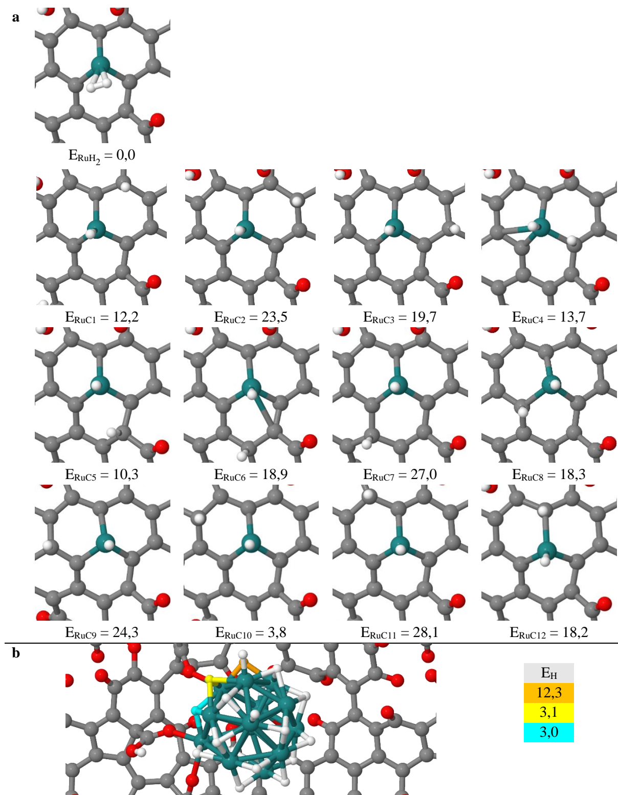
Figure 8 : Energies de réaction calculées (en \text{kcal.mol}^{-1} ) pour le système Ru_{SA+NP} . (a) Activation de H_2 et dissociation hétérolytique de H_2 sur le Ru_{SA} . L'énergie est référencée par rapport à l'état non dissocié. (b) Processus de transfert de H de la Ru_{NP} au Ru_{SA} . Schéma de couleurs atomiques : Ru (vert céladon) ; O (rouge) ; C (gris) ; H (blanc).
