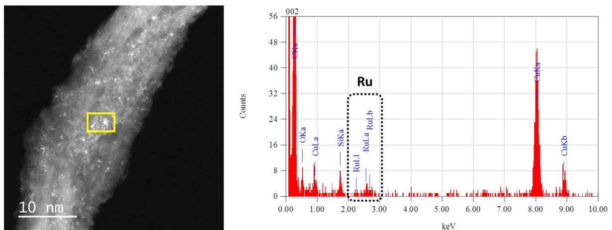
Figure 3 : Analyse STEM-EDX du catalyseur Ru_{SA}/CNT .
