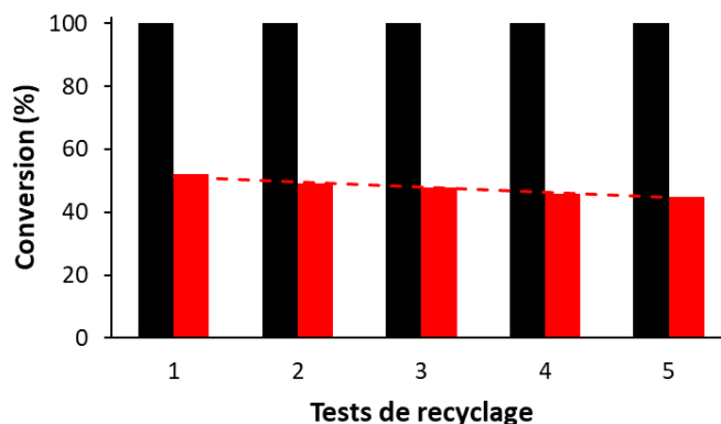
Figure 19 : Expériences de recyclage à 100 % (barres noires) et 50 % (barres rouges) de conversion réalisée sur le catalyseur Pd/N-CNT pour la réduction du 4-NP sous H_2 .
