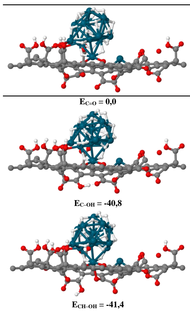
Figure 13 : Energies de réaction calculées (en kcal.mol -1 ) pour le processus d'hydrogénation du C=O en CH-OH. Les énergies sont référencées par rapport au système Pd NP+SA . Schéma de couleurs atomiques : Pd (bleu marine) ; O (rouge) ; C (gris) ; H (blanc).
