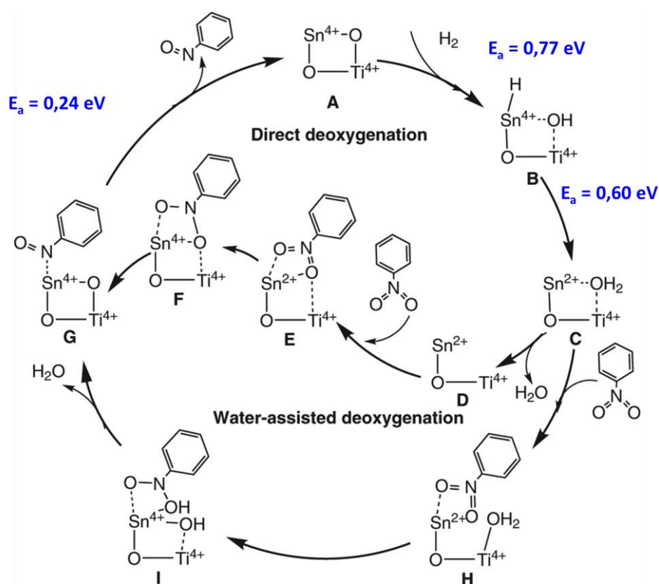
Schéma 3 : Mécanisme proposé de désoxygénation catalytique du nitrobenzène sur \text{Sn}_{\text{SA}}/\text{TiO}_2 . Issu de la référence [19].
