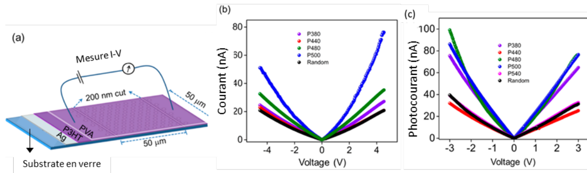
Figure 7.2. (a) Représentation schématique utilisée pour les mesures de conductivité sous ESC (b) Courbes I-V de rr-P3HT en fonction de la périodicité des réseaux de trous, (c) Courbes I-V de rr-P3HT en fonction de la périodicité des réseaux de trous sous illumination visible. Reproduit de la réf [197].
