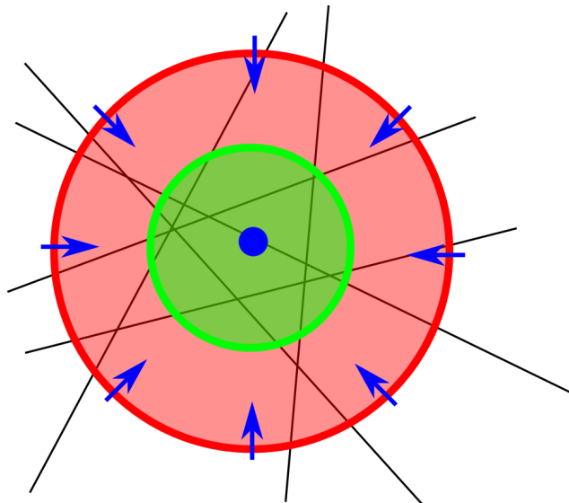
FIGURE 5: Illustration de la résolution pour la tomographie Backus–Gilbert. Le problème est d’estimer un paramètre physique au point bleu à partir des données obtenues pour les trajets illustrés par les lignes noires. La résolution signifie que la valeur estimée au point bleu sera une moyenne spatiale de la vraie Terre, par exemple la région en rouge : la fonction de résolution . L’inversion Backus–Gilbert cherche à minimiser la taille de cette région. L’inversion SOLA cherche à minimiser l’écart entre la fonction de résolution et une fonction de résolution cible , par exemple la région en vert.
