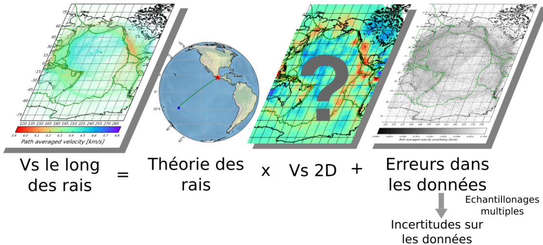
FIGURE 6: Illustration du problème direct pour la régionalisation (deuxième étape de l'inversion en deux étapes) dans le cadre de la théorie des rais. À gauche sont représentés les trajets source-récepteur, colorés en fonction des vitesses moyennes des ondes S le long des rais issues de la première étape à 75 km de profondeur. La théorie des rais permet de relier ces données à la vitesse des ondes S à 75 km de profondeur. À droite est représentée l'incertitude pour chaque rai obtenue en comparant les trajets proches.
