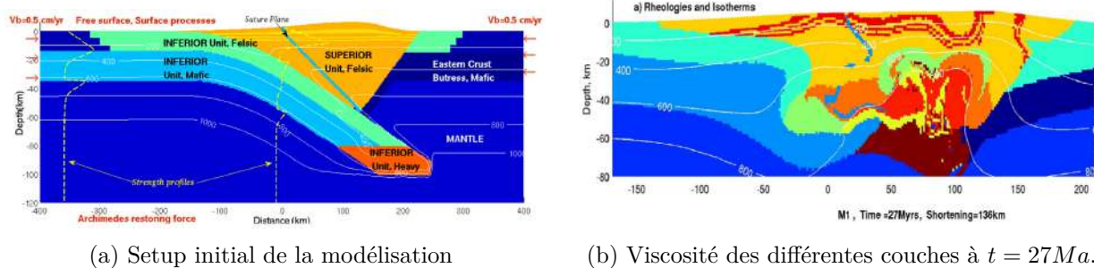
FIGURE 1.25 – Modélisation réalisée par GERBAULT et al. [2018] avec le code Parovoz basé sur une méthode explicite dite de relaxation dynamique sur grille "mobile" lagrangienne, appliquée à l'orogène Varisque dans un contexte de compression. Des dômes se forment par diapirisme après 27 Ma de convergence (en vert et jaune sur le snapshot b).
