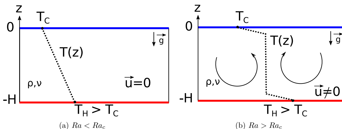
FIGURE 1.14 – Schéma illustrant l'instabilité de Rayleigh-Bénard sur un système fluide chauffé par le bas et refroidi par le haut : (a) Lorsque le nombre de Rayleigh Ra est inférieur à une valeur critique Ra_c , le système ne convecte pas et la distribution verticale de température est linéaire. (b) Lorsque Ra > Ra_c , le système convecte et la température est relativement homogène sauf près des parois supérieure et inférieure.
