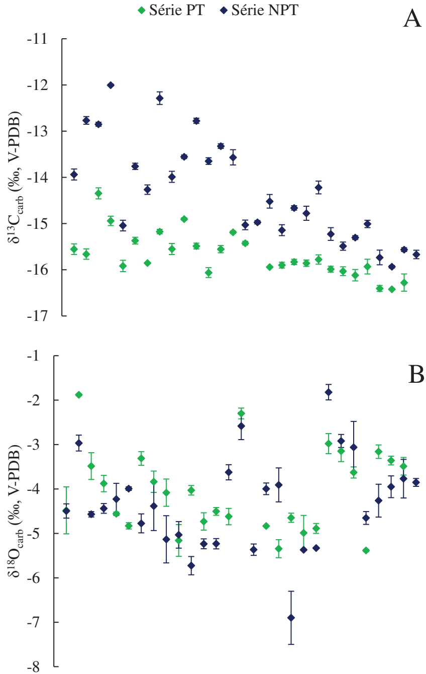
Figure 64 : Comparaison des compositions isotopiques du carbone (A, \delta^{13}\text{C}_{\text{carb}} , ‰ V-PDB) et de l'oxygène (B, \delta^{18}\text{O}_{\text{carb}} , ‰ V-PDB) mesurées sur les groupements carbonates de l'apatite des échantillons du squelette d'humain moderne entre une série prétraitée (PT) et une série non prétraitée (NPT). Les échantillons sont classés par ordre croissant de gauche (SA-1) à droite (SA-29).
