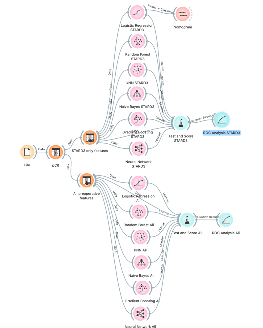
Figure 22. Workflow du développement des modèles prédictifs
