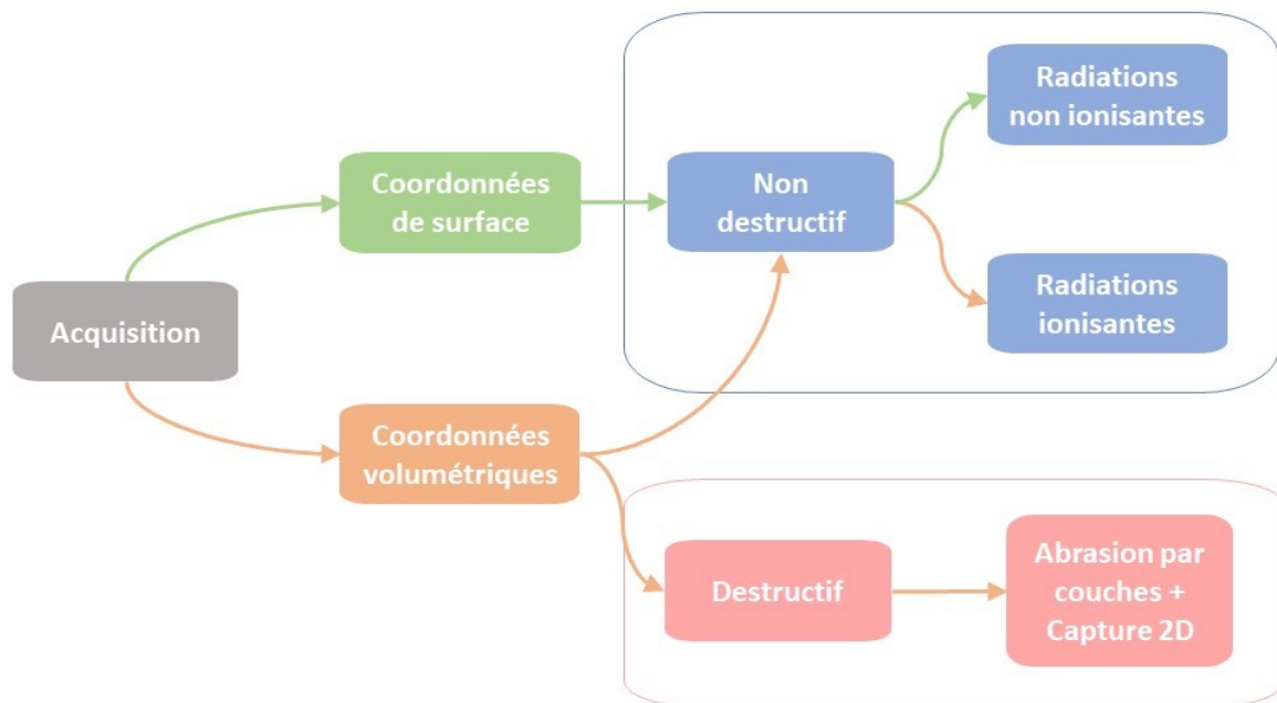
Figure II.1 : Familles de numérisations sans contact
