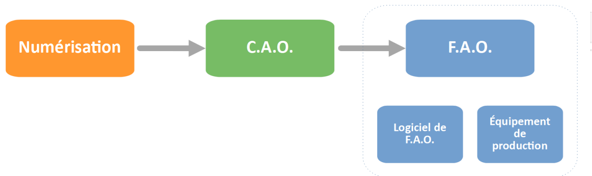
Figure I.1 : Les maillons de la chaîne CFAO
