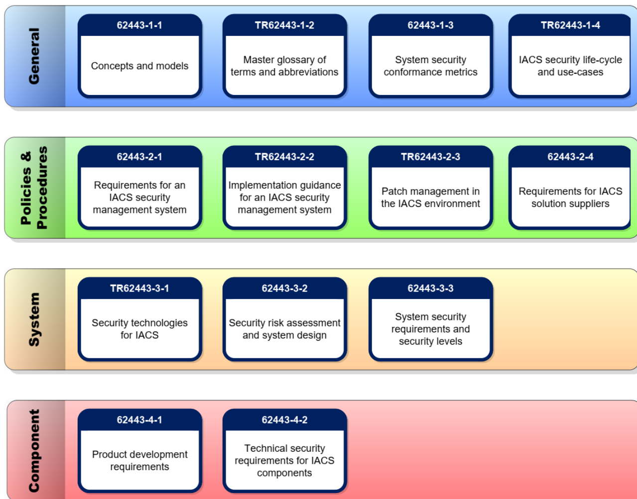
FIGURE 5.2 – Composantes de ISA/IEC 62443 (Niemann, 2017).
