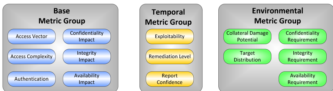
FIGURE 3.1 – Groupes de métriques CVSS (Mell et al., 2007).
