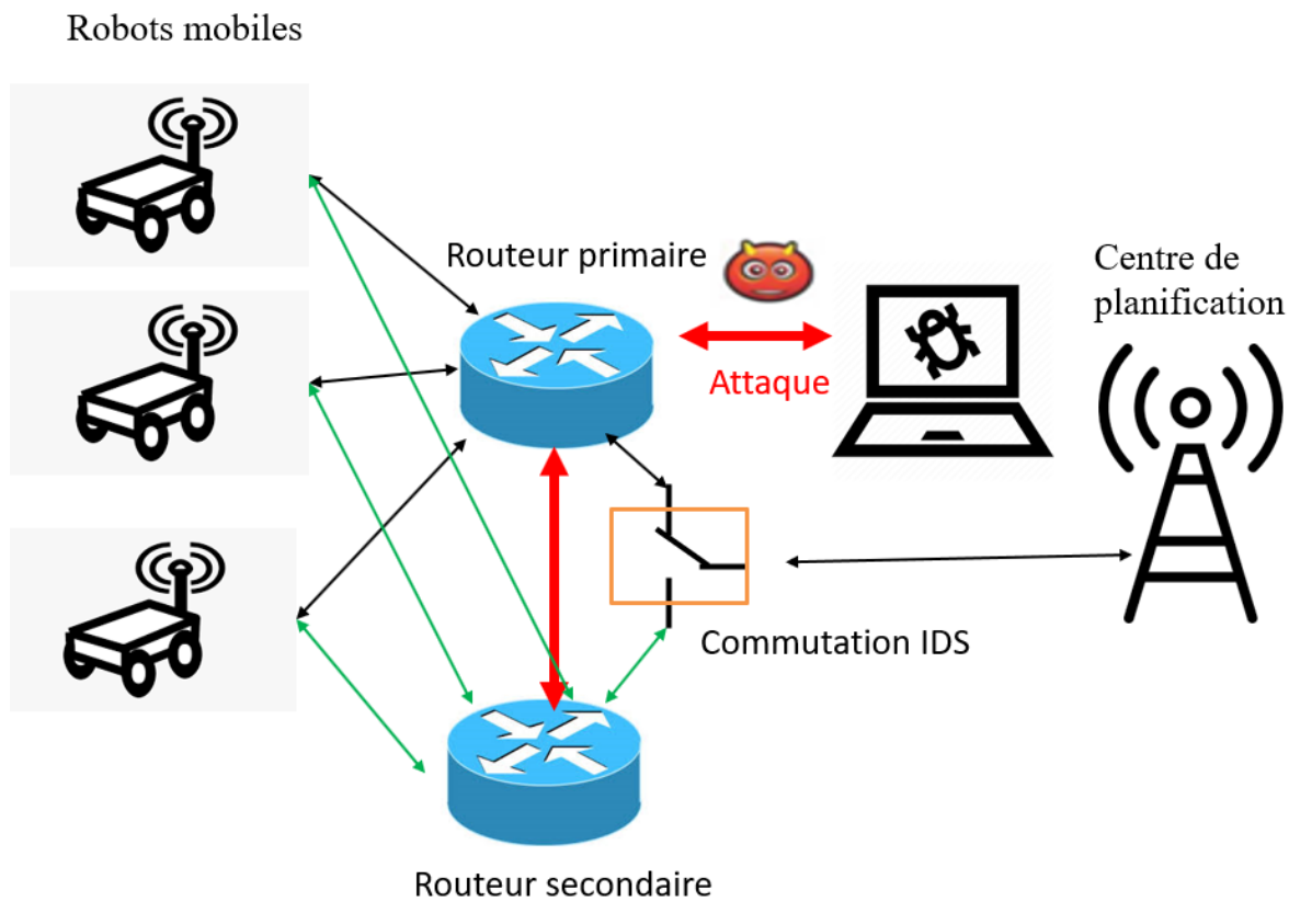
FIGURE 5.21 – Architecture duplex (redondance) pour renforcer la disponibilité
