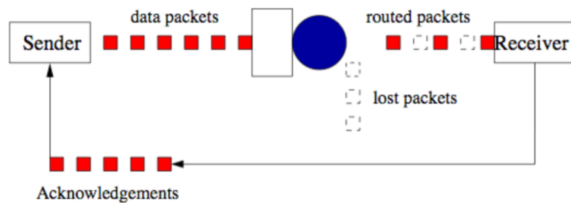
FIGURE 5.15 – Pertes des paquets au niveau du routeur (Hollot et al., 2002)
