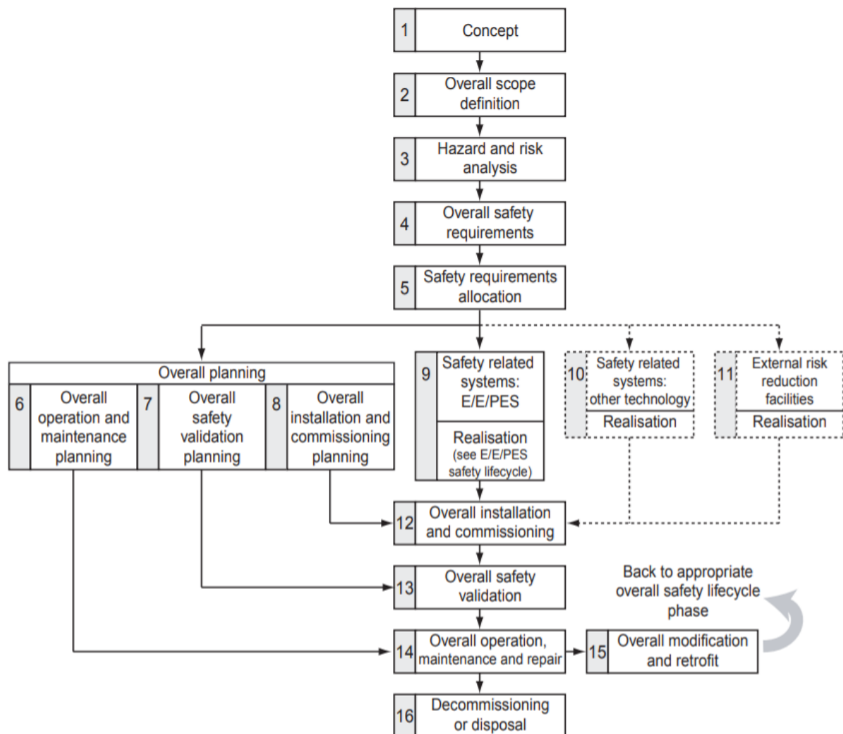
FIGURE 5.1 – Cycle de vie global de la sécurité-innocuité de la CEI 61508 (Brun et al., 2013) (Lundteigen, 2009).
