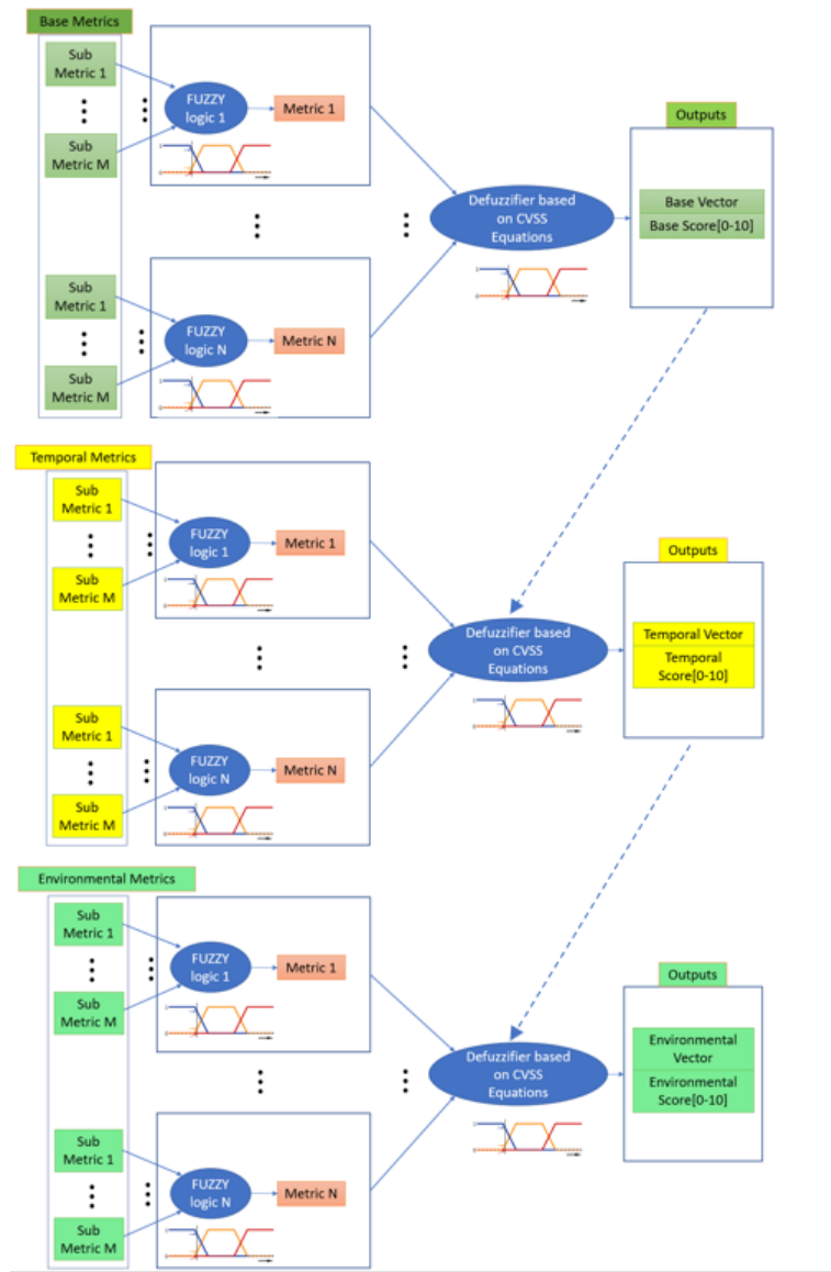
FIGURE 4.7 – Méthodologie floue ICVSS
