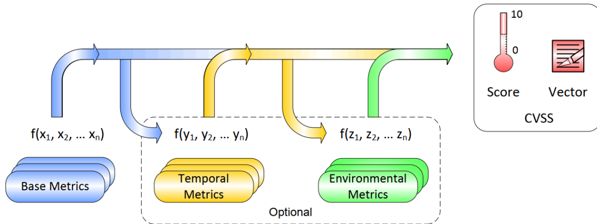
FIGURE 3.2 – Métriques et équations du CVSS (Mell et al., 2007).
