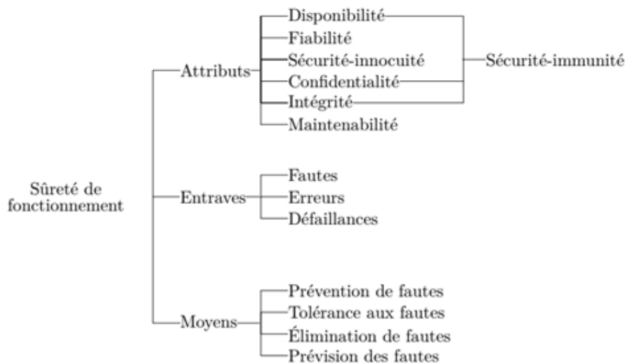
FIGURE 1.3 – Arbre de la sûreté de fonctionnement (Avizienis et al., 2004).
