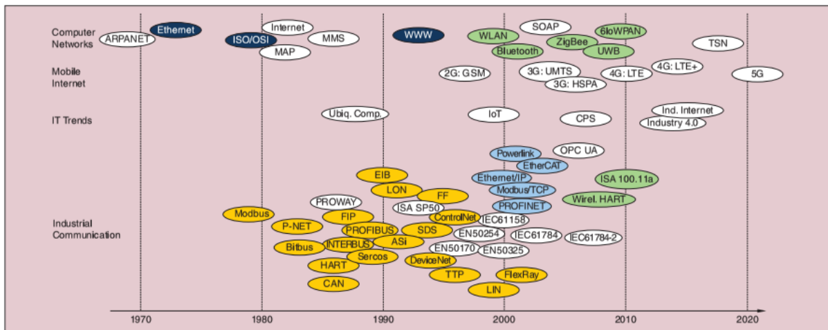
FIGURE 4.1 – Protocoles de communication dans les ICS et les secteurs technologiques associés (Wollschlaeger et al., 2017).
