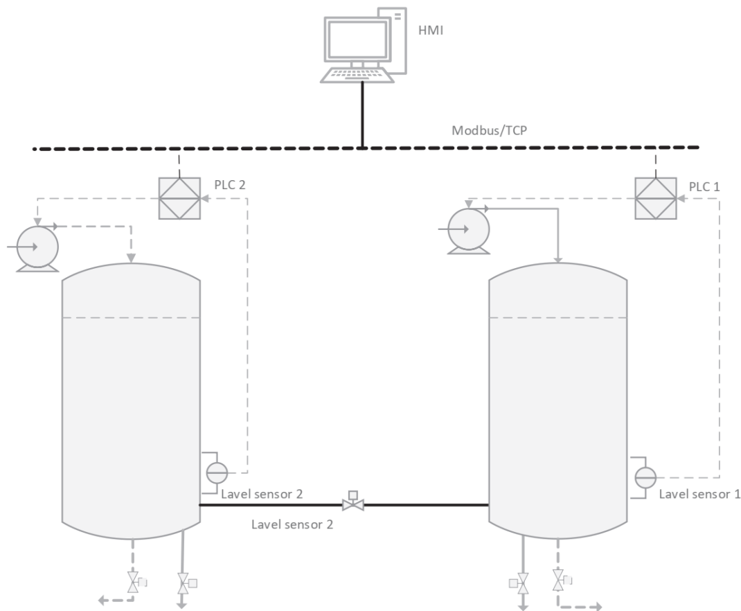
FIGURE 3.6 – Système à deux réservoirs sans système de SAF.
