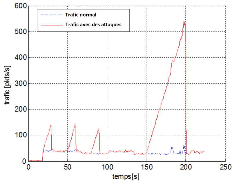
FIGURE 5.17 – Trafic normal vs trafic avec une attaque DoS de type rampe (CHEMALI et al., 2017)
