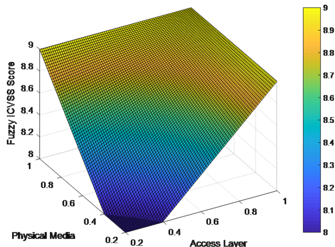
FIGURE 4.10 – Variation du score ICVSS flou par rapport à la couche d’accès (AM) et au moyen physique (PM)
