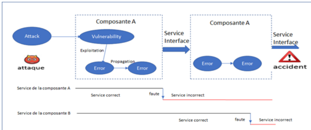
FIGURE 1.5 – Exploitation de la vulnérabilité par une attaque.
