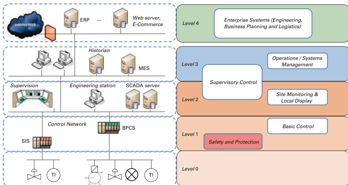
FIGURE 1.1 – Modèle de Purdue de l'architecture d'un ICS (Flaus, 2018).
