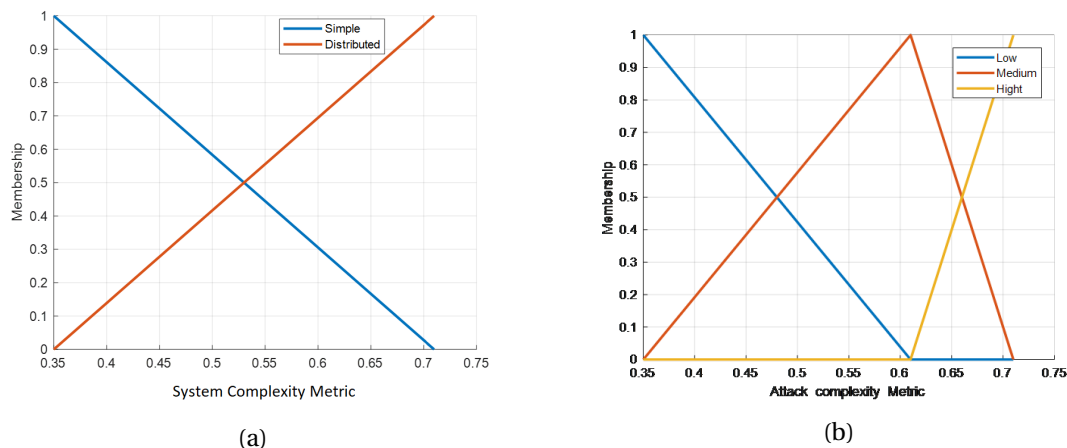
FIGURE 4.9 – Fonctions d’appartenance de : (a) complexité du système (SC), (b) complexité attaque (AC)
