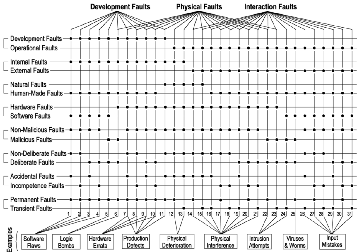
FIGURE 1.6 – Classes de défauts combinés (Avizienis et al., 2004).
