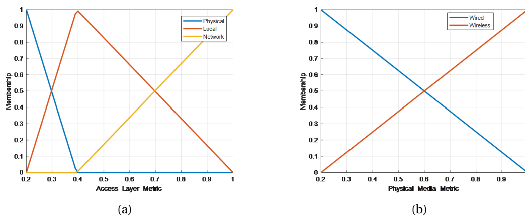
FIGURE 4.8 – Fonctions d'appartenance de : (a) couche d'accès (AL) , (b) moyen physique (PM)
