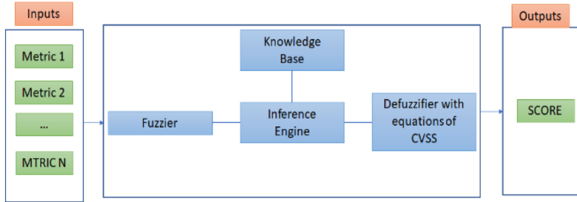
FIGURE 4.5 – Concepts de la logique floue.
