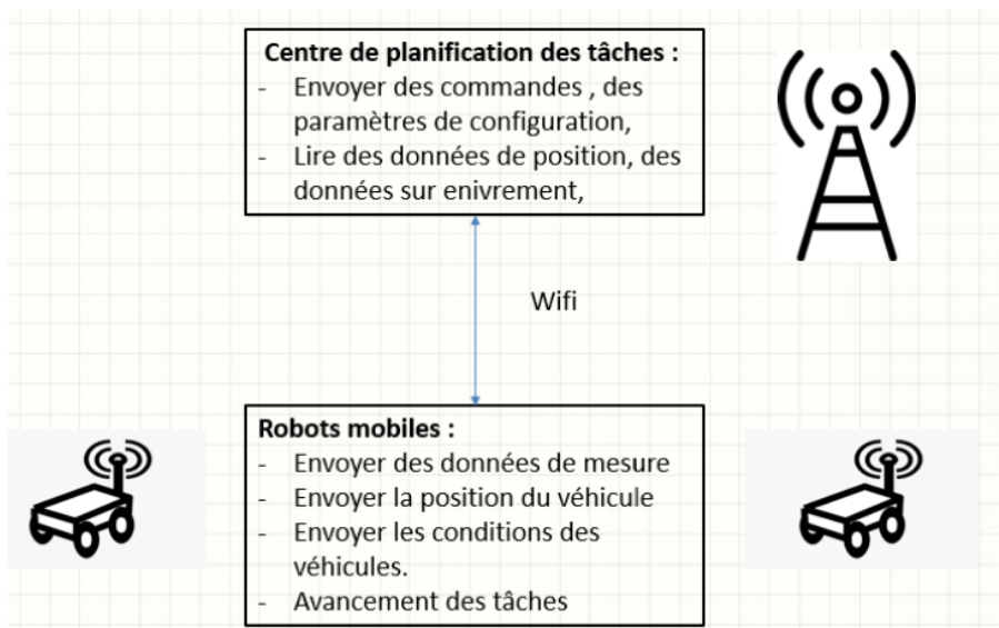
FIGURE 5.14 – Communication bidirectionnelle entre les robots et la station
