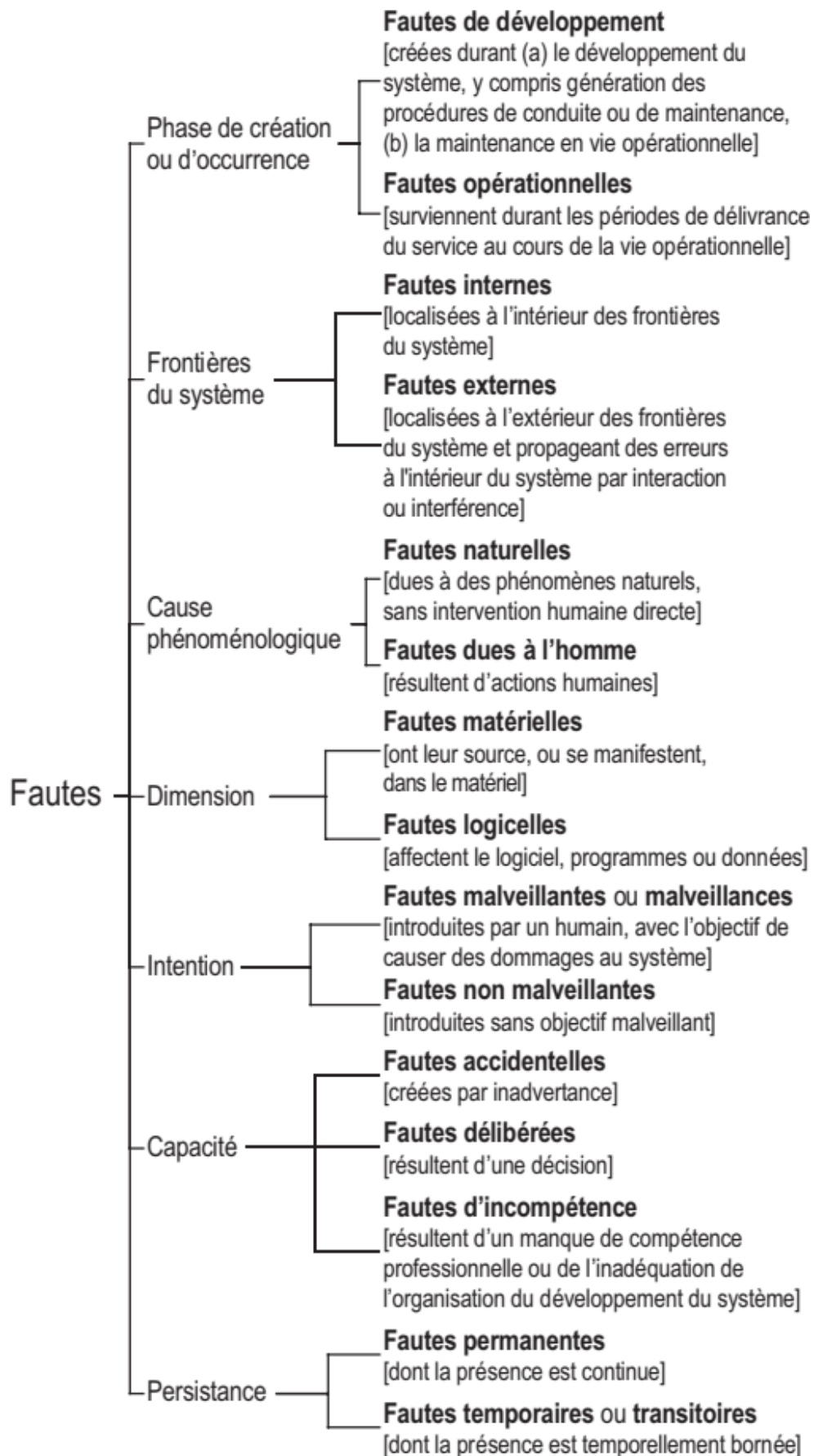
FIGURE 1.4 – Classes de fautes élémentaires (Arlat et al., 2006).
