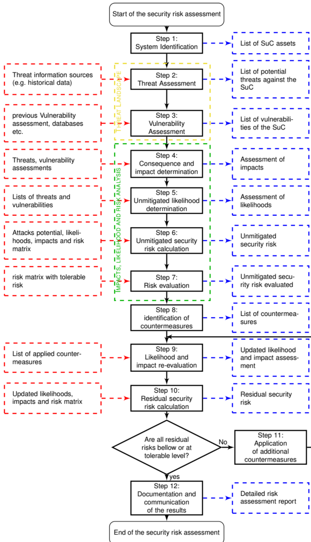
FIGURE 5.3 – Méthode d'évaluation des risques de sécurité ISA/IEC-62443 (Rekik et al., 2018).
