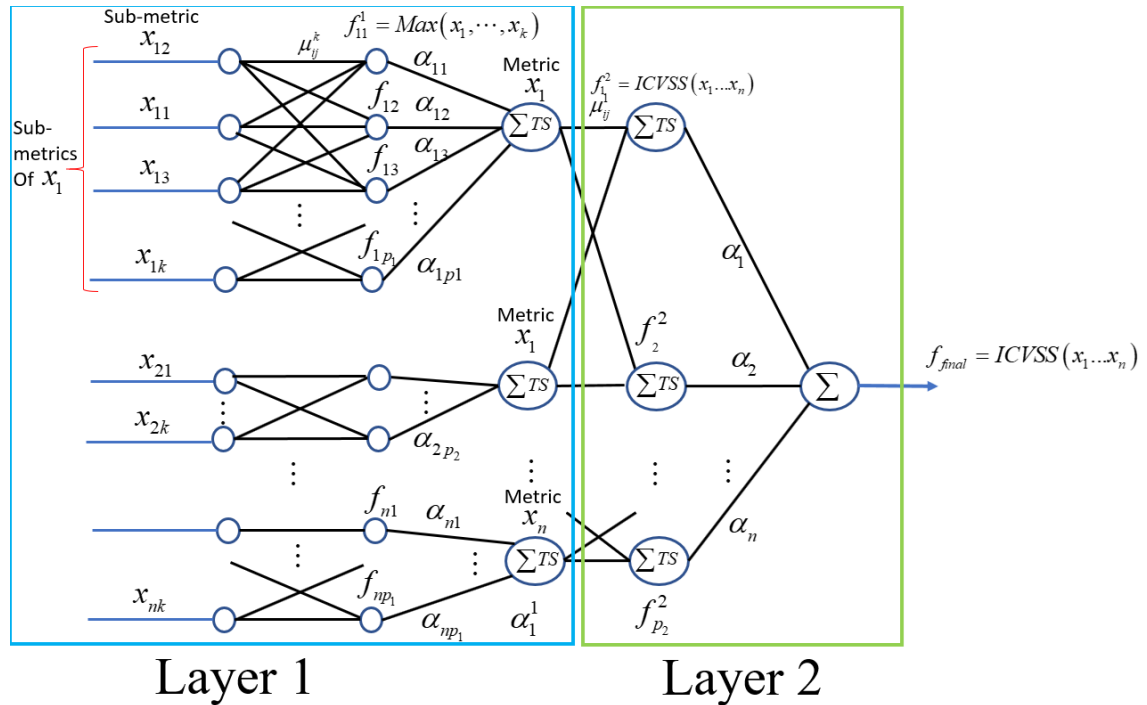
FIGURE 4.6 – ICVSS basé sur l'algorithme de Takagi-Sugeno
