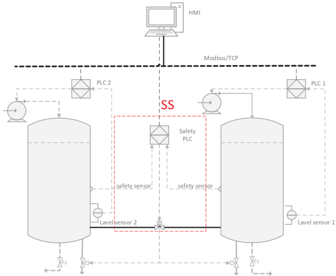
FIGURE 3.10 – Système à deux réservoirs avec un système de SAF (SS).
