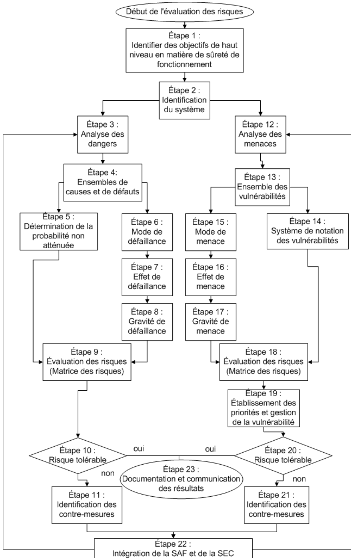
FIGURE 5.9 – Méthodologie d'évaluation des risques basée sur les normes ISA/IEC-62443 et IEC-60812 (AMDVEC & ER)
