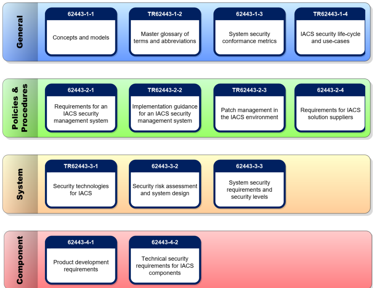
FIGURE 5.2 – Composantes de ISA/IEC 62443 (Niemann, 2017).
