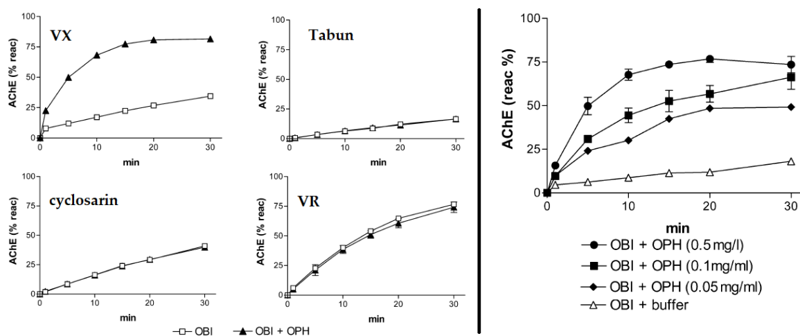
Figure 56. Effet de l'OPH (0.2 mg/mL à gauche – concentration variable à droite) sur les cinétique de réactivation des OP-hAChE par l'obidoxime (OBI dans le diagramme, 20 µM) 330
