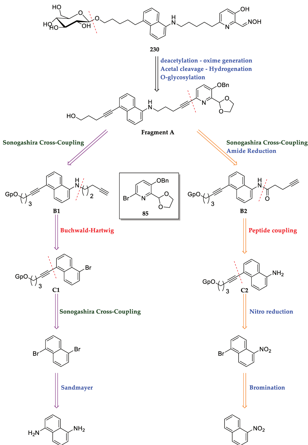
Figure 218. Retrosynthèses envisagées
