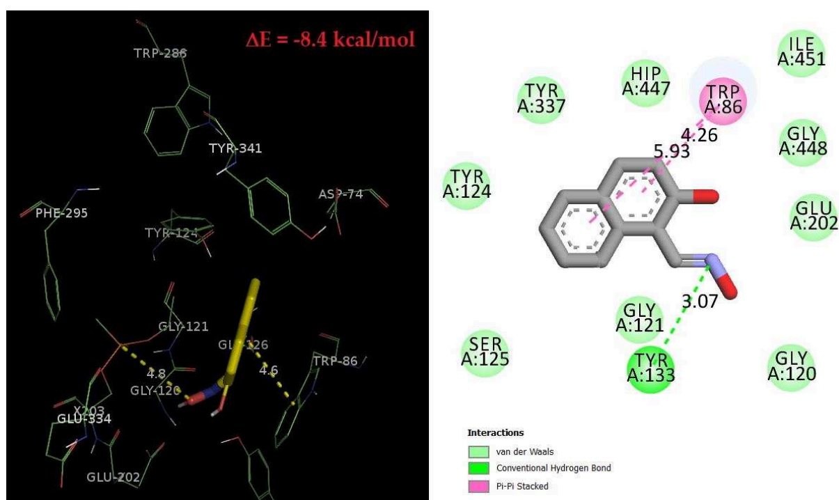
Figure 245. Conformation prédominante obtenue dans la mACHé inhibée par le VX (Docking flexible à gauche visualisation sur Pymol et docking statique à droite visualisé sur Discovery Studio)
