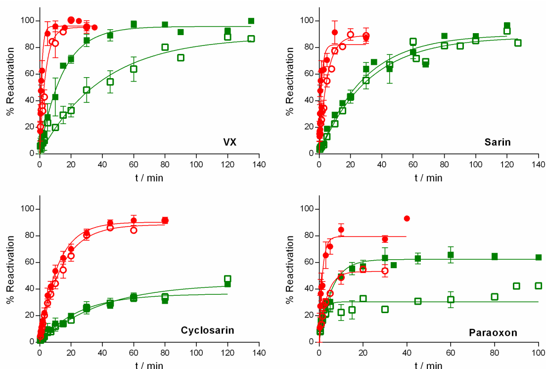
Figure 136. Récupération de l'activité cholinergique dans le sang humain empoisonné au NOPs (symbole plein, 0.7 µM ; symbole vide : 3.4 µM) et traité par le JR595 (1 mM, en rouge) et le GM415 (1mM, en vert)
