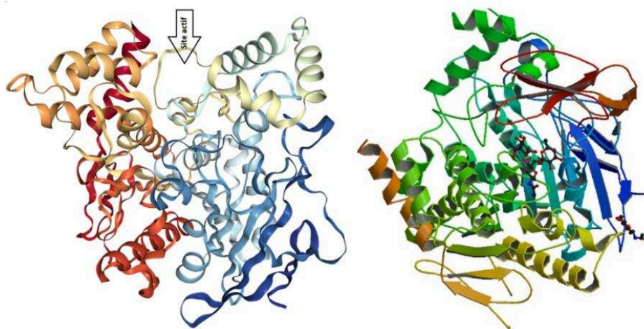
Figure 26. Structure tridimensionnelle de la TcAChE native (à gauche – code PDB 1EA5) et de la hAChE-FAS (à droite -code PDB 1B41)
