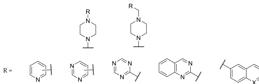
Figure 202. Amines à envisager comme ligands du site périphérique
