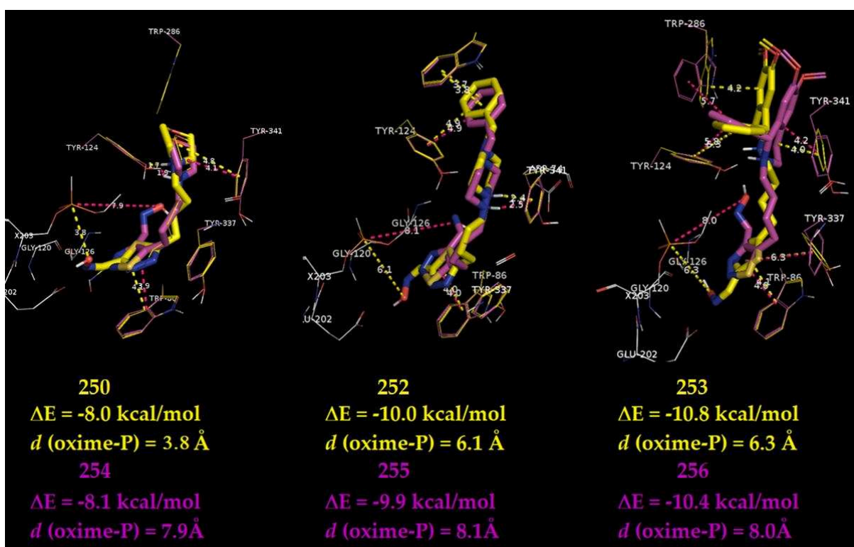
Figure 233. Superposition des conformations proposées des réactivateurs 250, 252 à 256 (Docking flexible - visualisé sur Pymol version 2.0.7) dans la mAChE inhibée par le VX.
