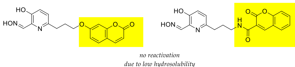
Figure 228. Réactivateurs fluorescents étudiés par le Dr Julien Renou
