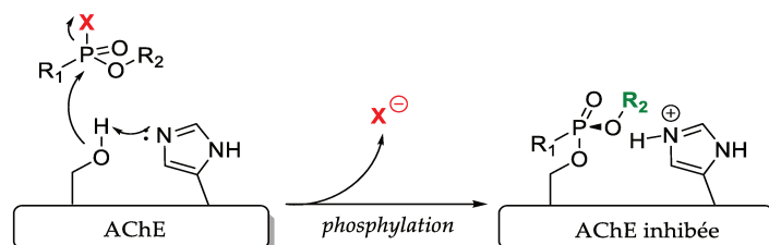
Figure 33. Phosphorylation de l'AChE
