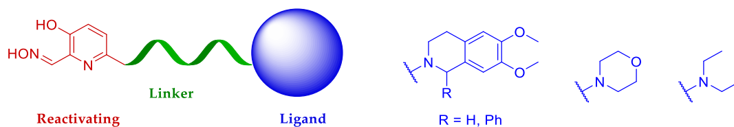
Figure 10. Structure générale des réactivateurs non-chargés resynthétisés
