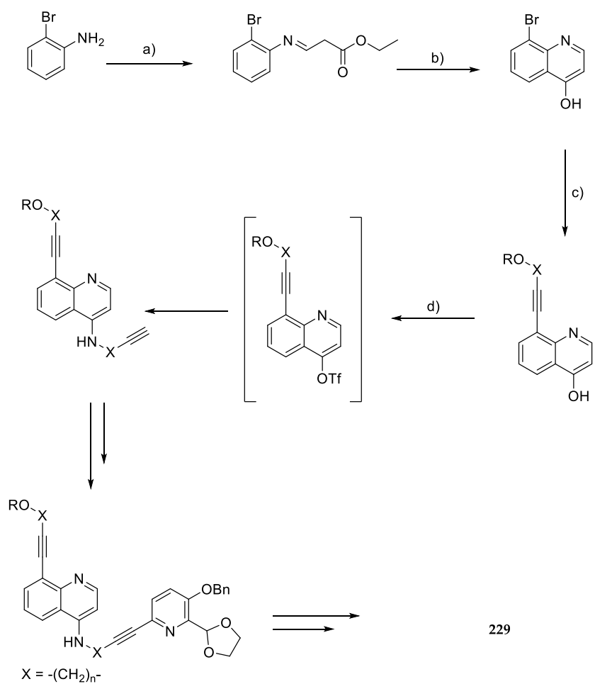
Figure 224. Voie de synthèse possible de la molécule 229
