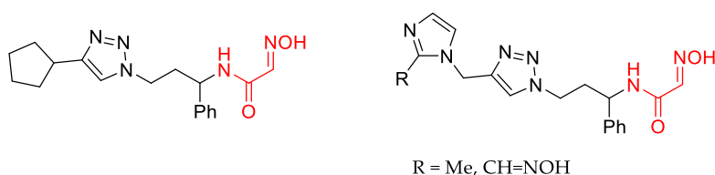
Figure 96. Réactivateurs de Maraković et coll.
