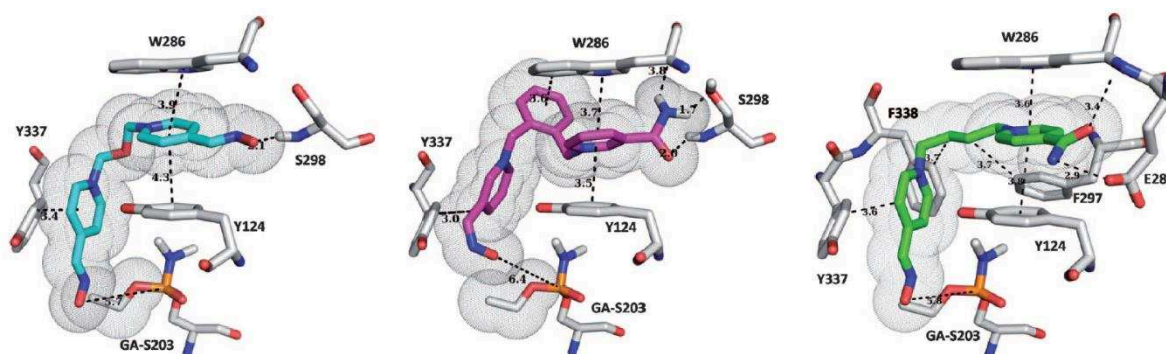
Figure 76. Etude d'amarrage moléculaire de l'obidoxime (en bleu – à gauche) du K646 (en magenta – au centre) et du K203 (vert – à droite) sur la mAChE inhibée par le tabun (pdb : 2JEZ) 427
