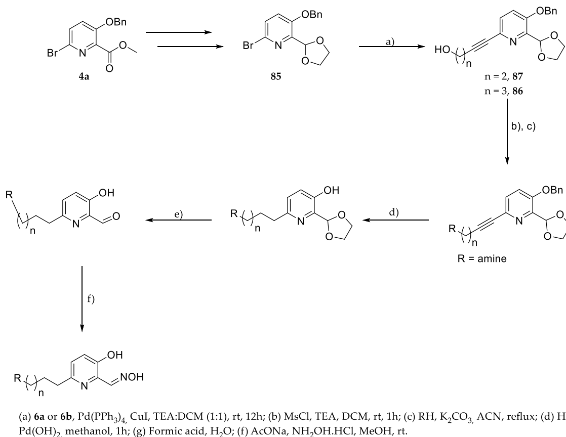
Figure 203. Voie alternative d'accès aux réactifs possible
