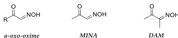
Figure 91. Structure générale des α-oxo-oximes (R = alkyle ou aryle) ainsi que les deux premiers exemples décrits
