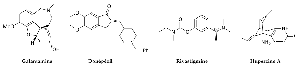
Figure 39. Structures des médicaments anti-Alzheimer testés comme neuroprotecteur des OPs
