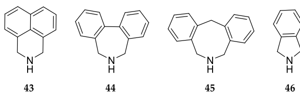
Figure 153. Amines libres désirées
