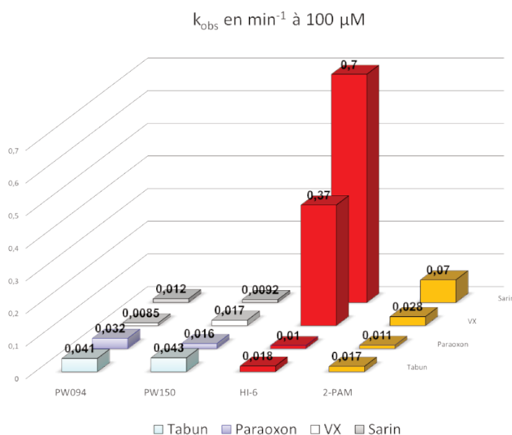
Figure 215. détermination des constantes k_{\text{obs}} de réactivation de la hAChE inhibée par 4 OPs. .
