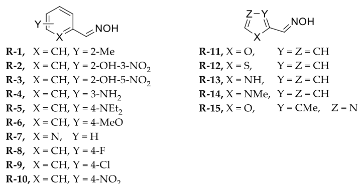
Figure 103. Fonctions réactivatrices synthétisées par Ribeiro et coll. 472,473
