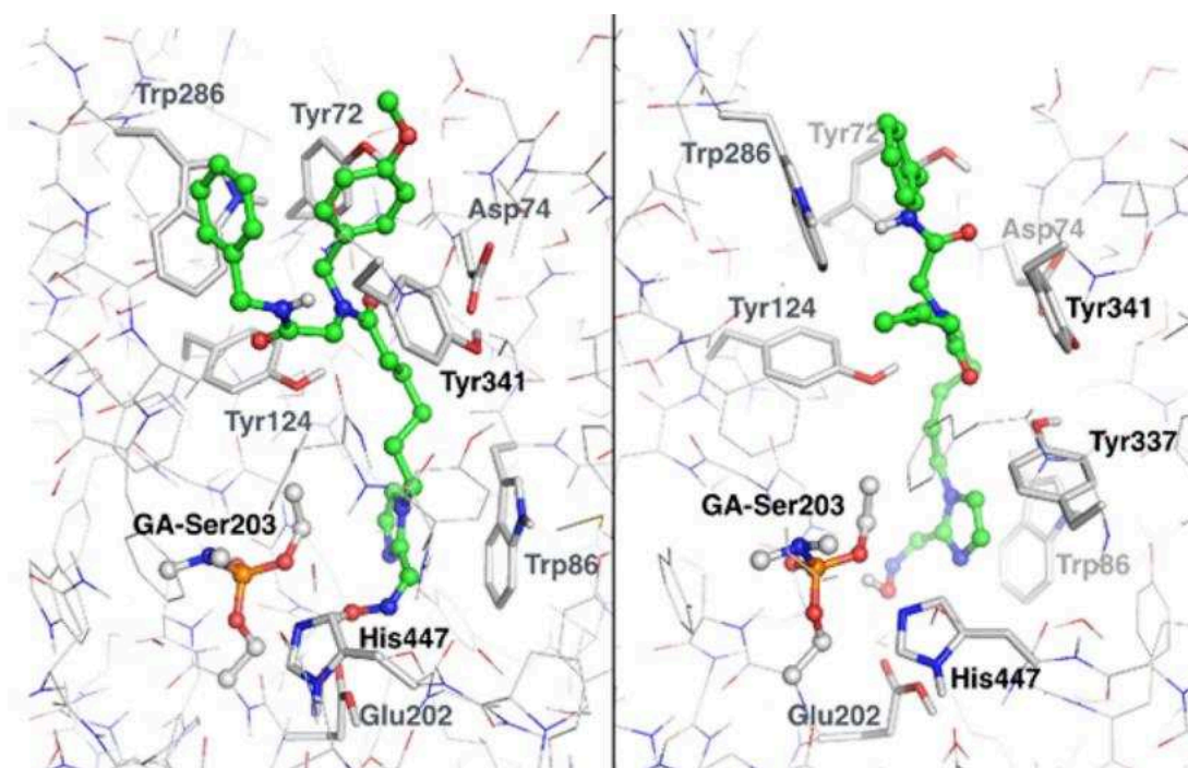
Figure 101. Étude d'amarrage moléculaire des molécules Ugi-12c (à gauche) et Ugi-12d (à droite) sur la hAChE inhibée par le tabun (pdb : 4EY4 et 3DL4).
