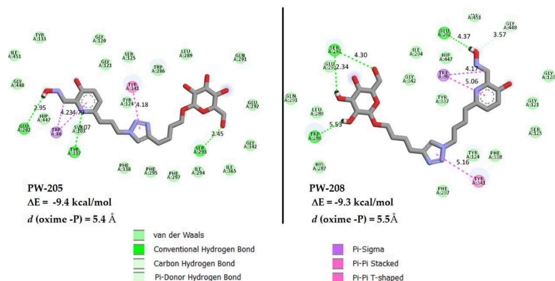
Figure 207. Interactions du PW205 (gauche) et PW208 (droite) avec la hAChE inhibée par le VX en docking statique (visualisées sur Discovery)
