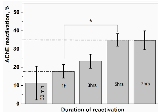
Figure 142. Réactivation des AChEs centrales du rat exposé au paraoxon et traité par les SLNs contenant la 2-PAM et le GM415
