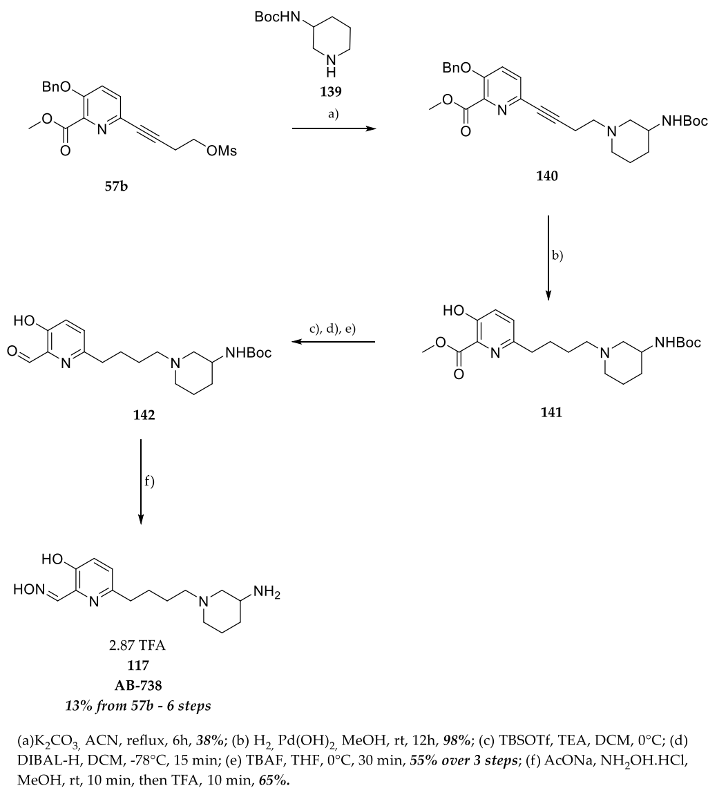
Figure 177. Synthèse du réactif 117
