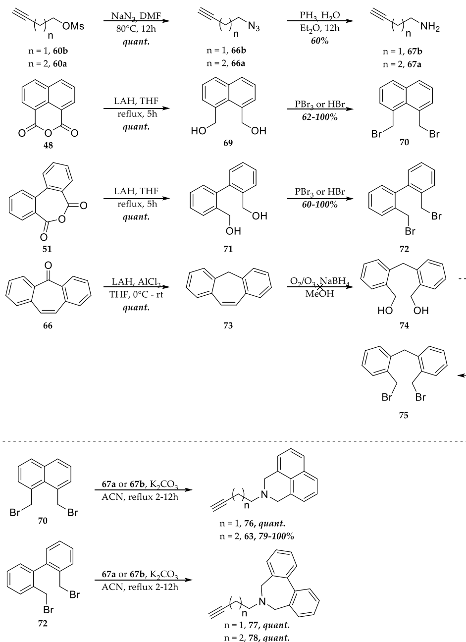
Figure 156. Génération des amines portant un bras espaceur
