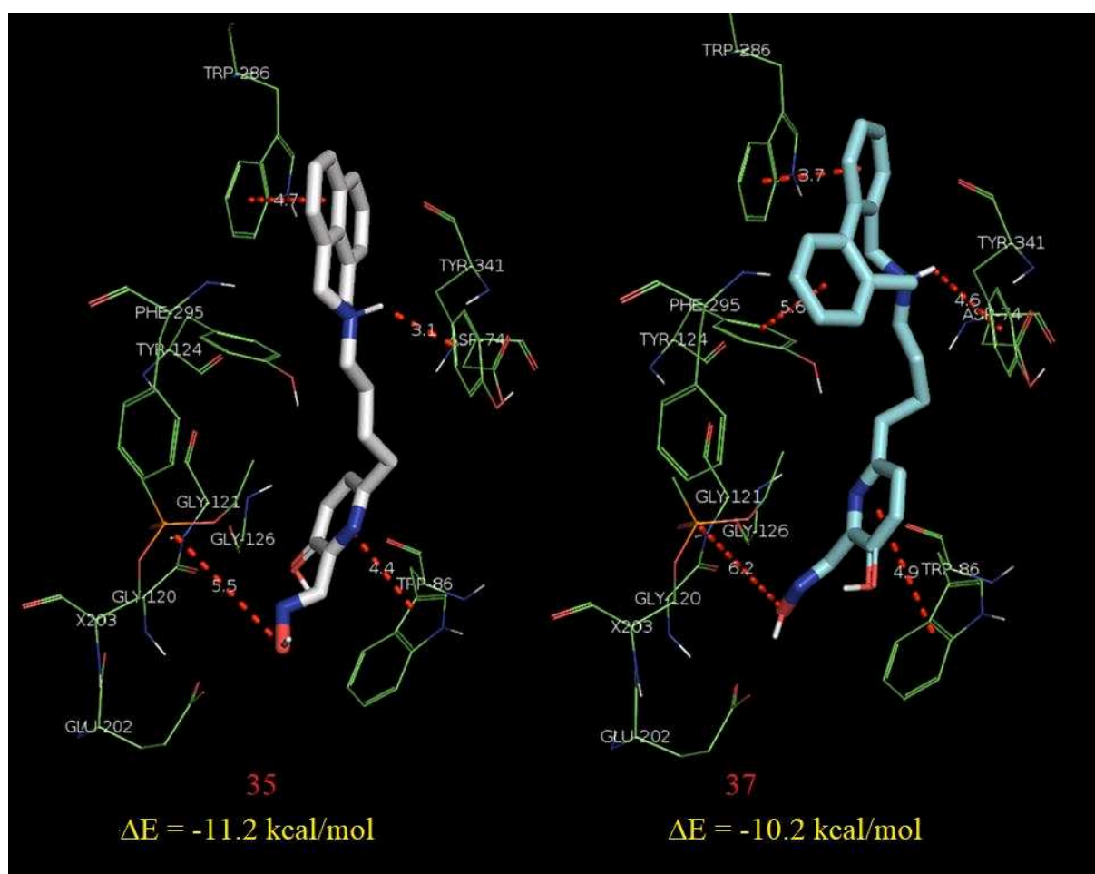
Figure 148. Conformations proposées des réactifs 35 (gauche) et 37 (droite) ; conformation prédominante – Docking statique - visualisé sur Pymol (version 2.0.7) dans la mAChE inhibée par le VX.
