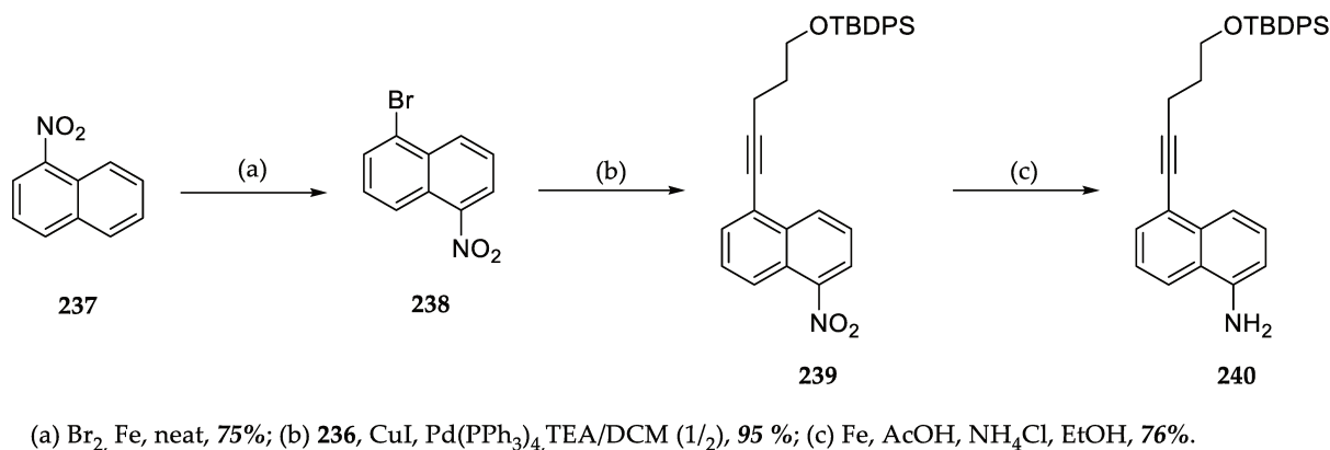
Figure 221. Synthèse de l'intermédiaire 240 .
