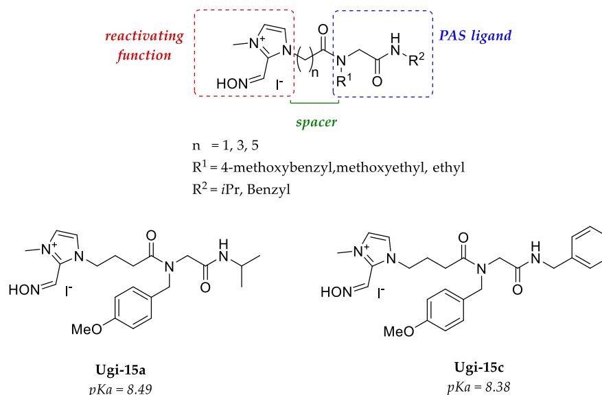
Figure 68. Imidazoliums oximes développées par De Koning
