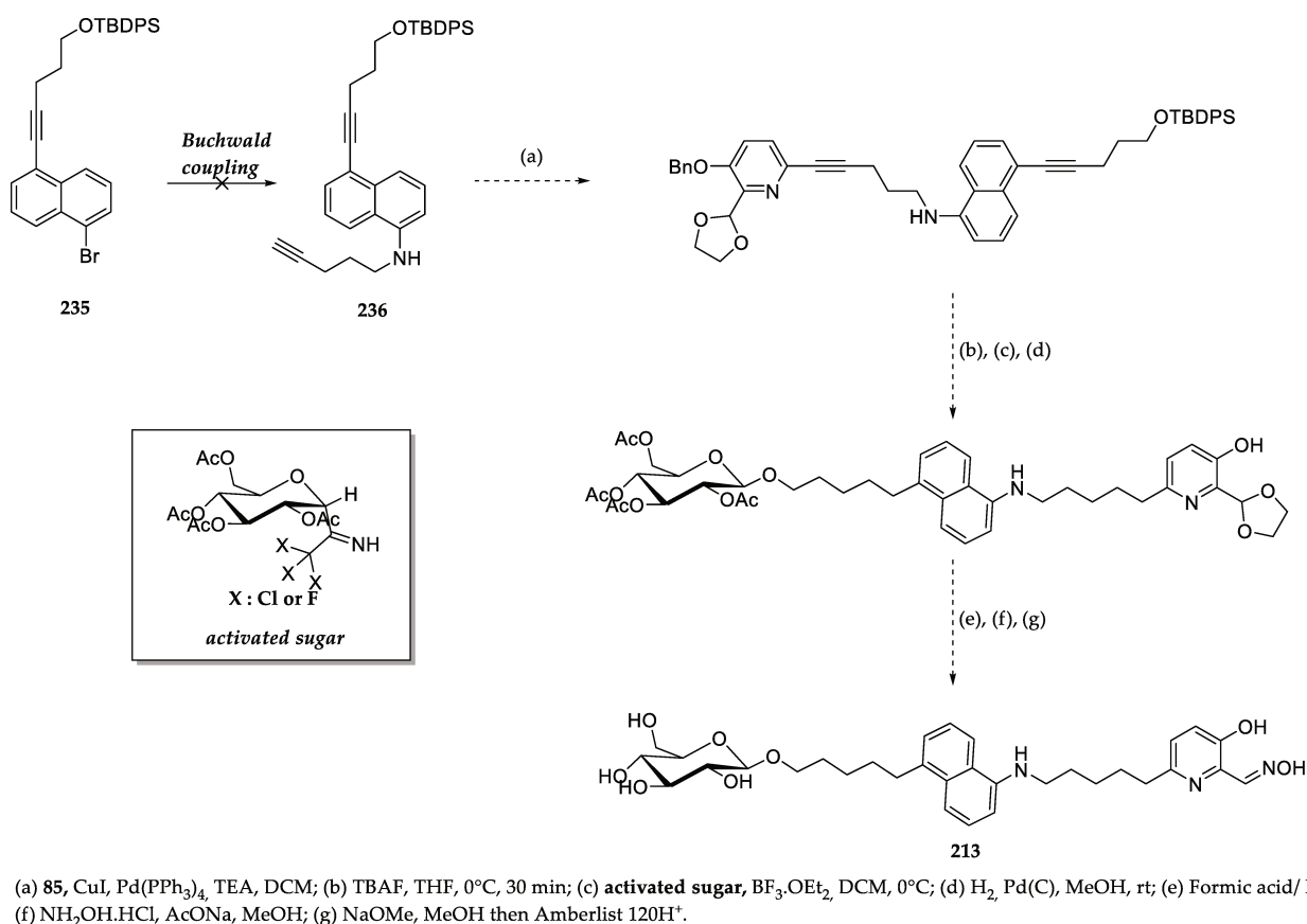
Figure 220. Fin de synthèse initialement envisagée
