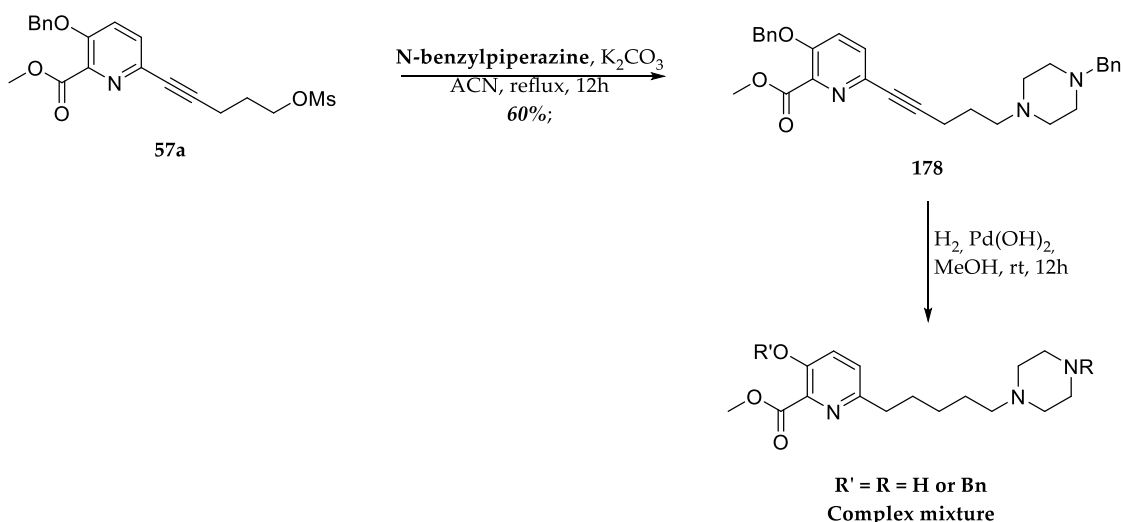
Figure 188. Voie de synthèse initialement envisagée pour le réactivateur 153
