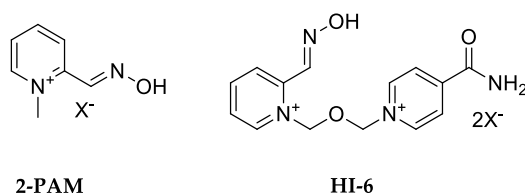
Figure 7. Structure du 2-PAM et du HI-6
