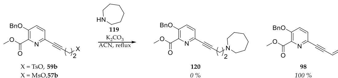
Figure 171. Tentative d'obtention de l'intermédiaire 120 par substitution nucléophile
