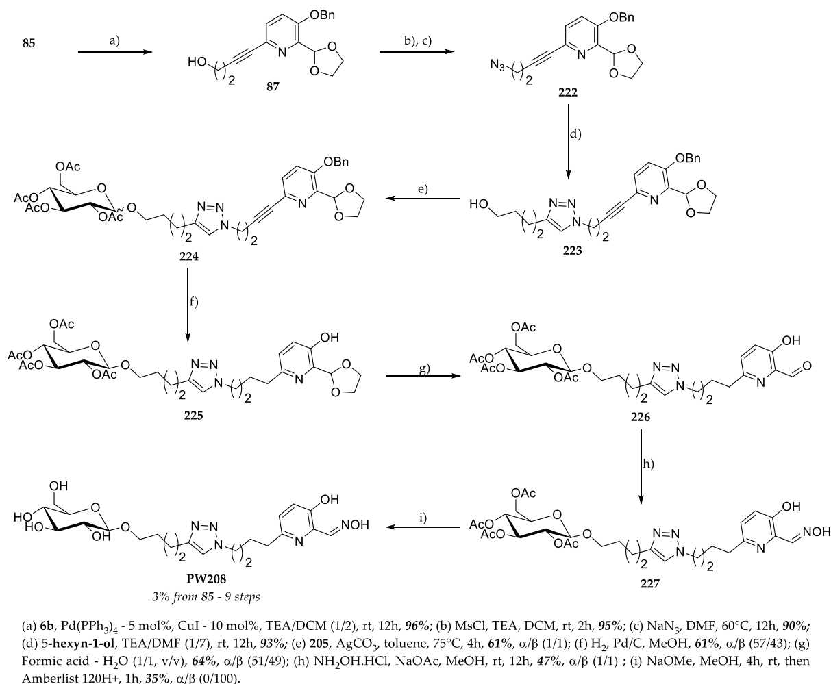
Figure 213. Synthèse optimisée du PW208
