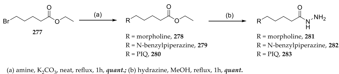
Figure 239. Synthèse des intermédiaires acylhydrazone 281 à 283
