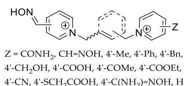
Figure 75. Bis-pyridiniums aldoximes rigides synthétisées 323,422-430
