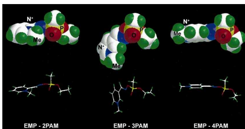
Figure 55. Structure 3D des phosphyloximes dérivés des PAMs 329
