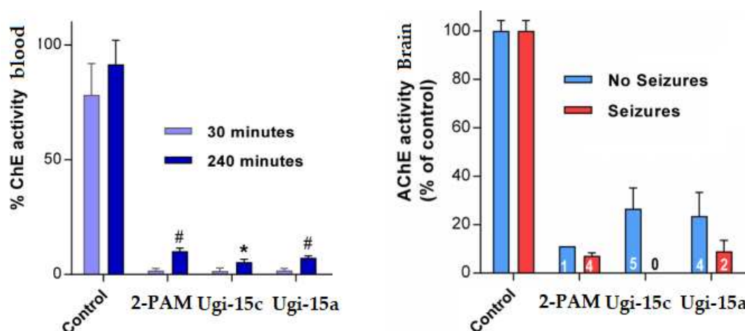
Figure 69. Activité cholinergique dans le sang des rats exposés au sarin (130 \mu\text{g/kg} SC) traités par les oximes (16 \mu\text{mol/kg} IV + 3mg/kg en IM d'atropine + 1 min) 30 min et 4h après exposition (à gauche) – Activité cholinergique dans le cerveau des rats 4h après exposition au sarin (à droite)
