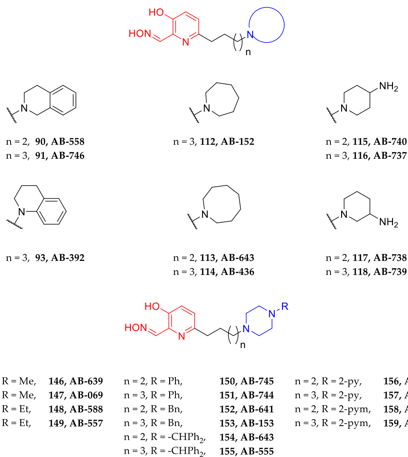
Figure 201. Structures des réactivateurs synthétisés dans ce chapitre
