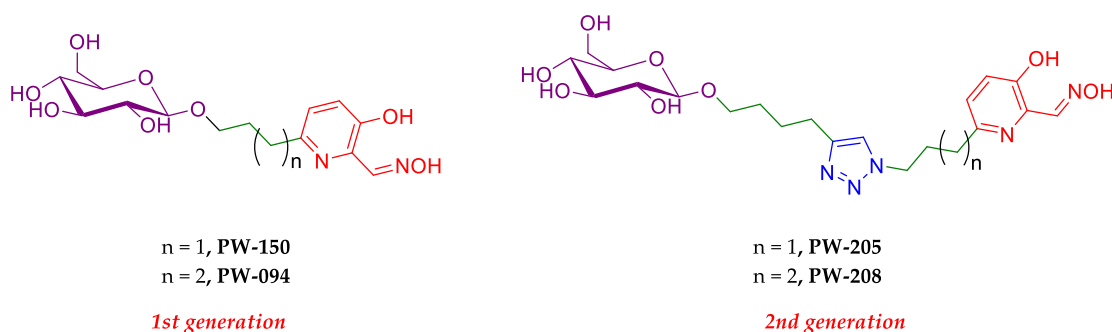
Figure 254. Réactivateurs présentés dans le chapitre 4 – 1 ère et 2 ème générations
