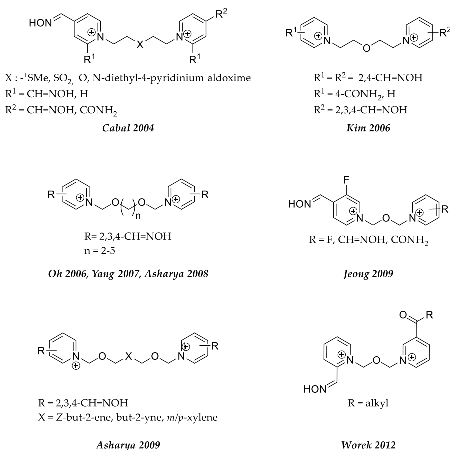
Figure 74. Structure des bis-pyridiniums aldoximes dont l'espaceur comprend un hétéroatome
