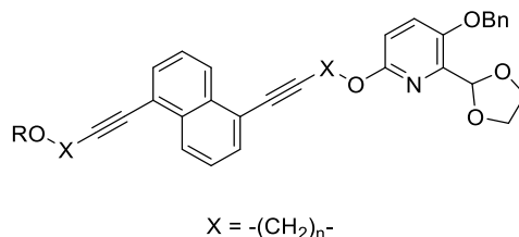
Figure 223. Intermédiaire incorporant le naphthalène
