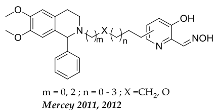
Figure 114. Structures des réactivateurs dérivés de la PIQ
