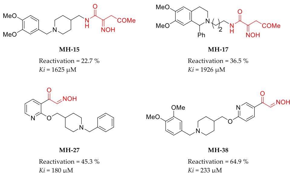
Figure 95. Structures et capacité in vitro de réactivation des leads de McHardy (20 \mu\text{M} ) sur la réactivation de l'AChE inhibée par le cyclosarin. 464
