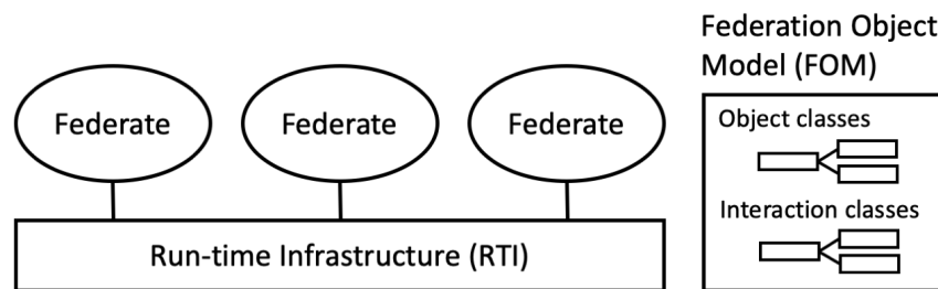
Figure 3.7: Architecture simplifiée de HLA
