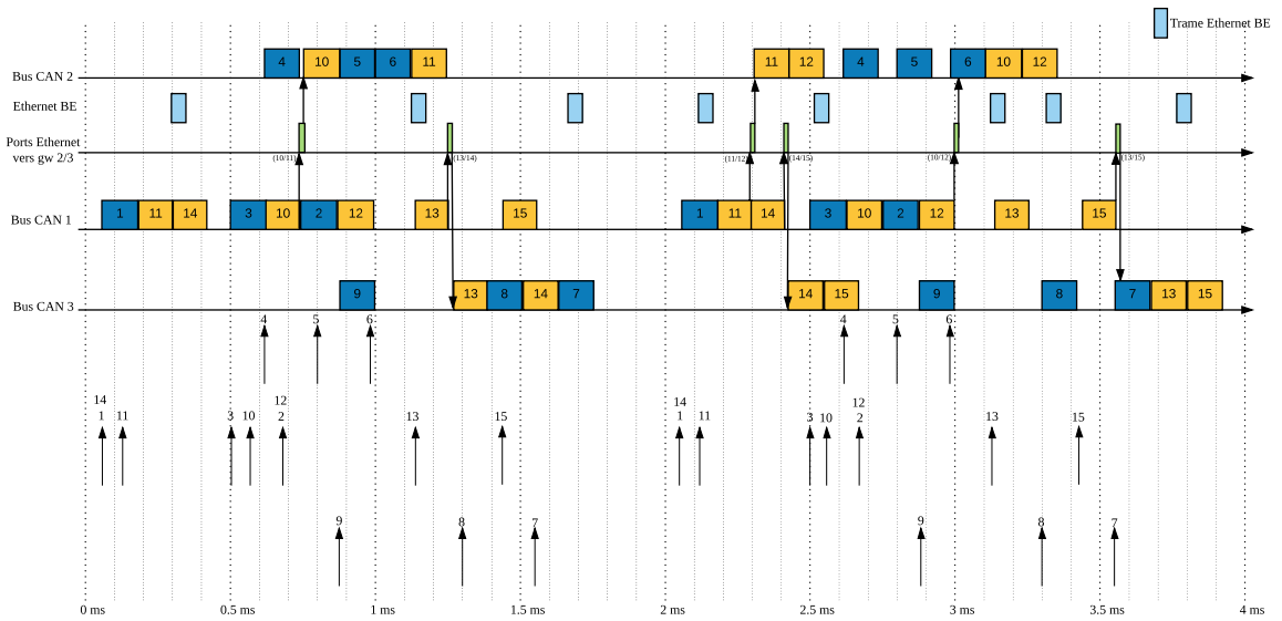
FIGURE 5.4 – Scénario avec deux trames CAN pour une trame Ethernet
