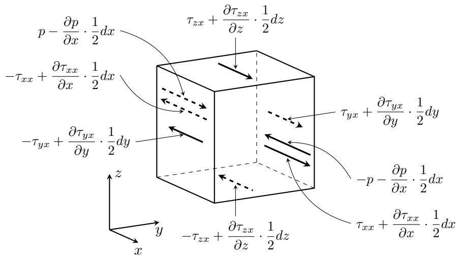
FIGURE 2.4 – Composantes des contraintes dans la direction x
