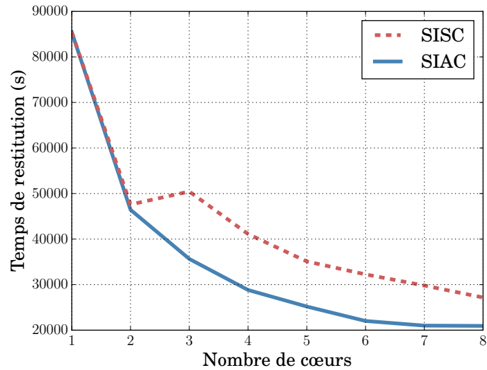
FIGURE 5.6 – Mur - Temps de restitution (s) sur le cluster local
