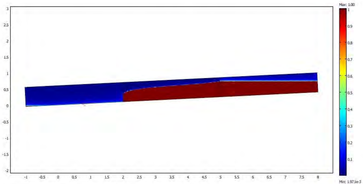
Figure 1.4.27 : Comparaison de la ligne d'eau expérimentale et modélisée par COMSOL pour le débit Q=10 l/s en cas du milieu poreux constitué des cailloux de diamètre moyen d=1 cm
