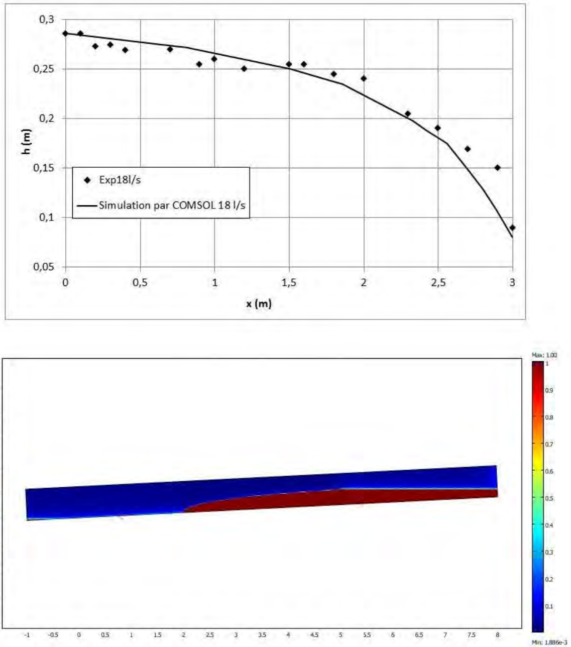
Figure I.4.36 : Comparaison ligne d'eau expérimentale et modélisée par COMSOL pour le débit Q= 18 l/s en cas du milieu poreux constitué des cailloux de diamètre moyen d=15 cm
