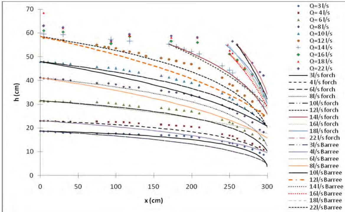
Figure I.4.21 : simulation de la ligne d'eau par la relation de Forchheimer (1901) et Barree et Conway (2004) pour une mèche de cailloux de diamètre moyen d=1\text{ cm} et pour les différents débits traités
