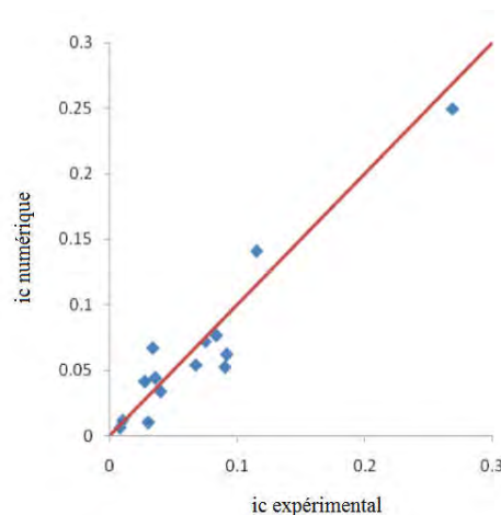
Figure II.1.1 : graphique comparant les résultats expérimentaux et numériques de gradient hydraulique critique (Jafar Chapokpour et Ebrahim Amiri Tokaldany (2012))
