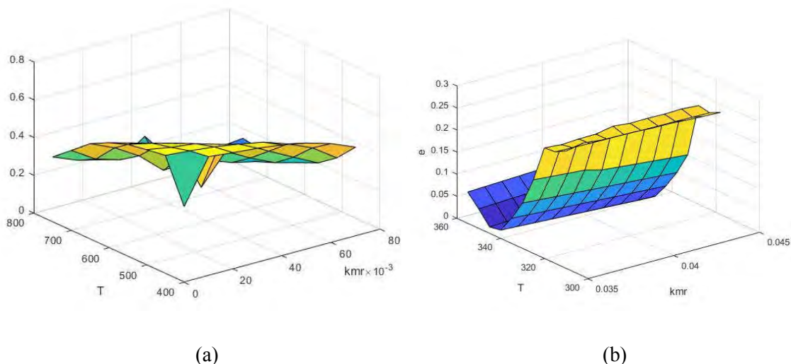
Figure I.4.4 : surface de l'erreur en fonction du couple de k_{mr} et T du modèle de Barree et Conway (2004) pour l'expérience avec des cailloux de diamètre moyen d=7\text{cm} ; (a)= 20l/s et (b)= 30 l/s
