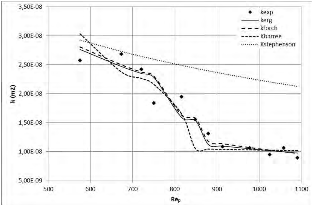
Figure I.4.18 : simulation des expériences en cas d'écoulement turbulent
