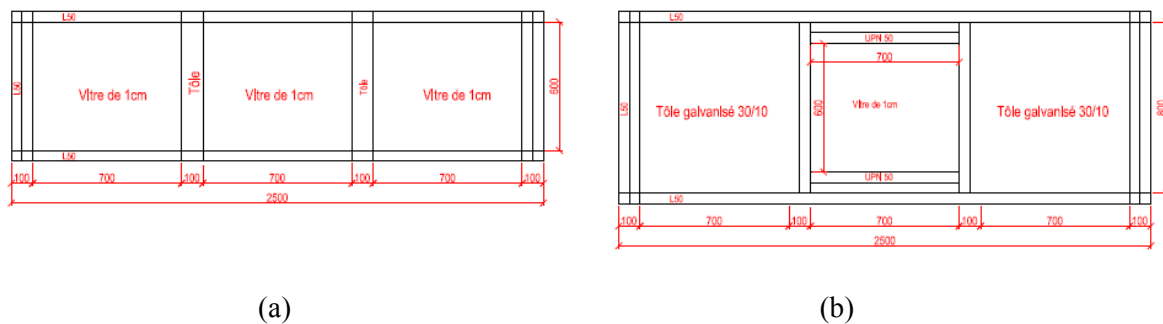
Figure I.2.3 : Schéma des vitres (a) et des couvercles du canal (b)
