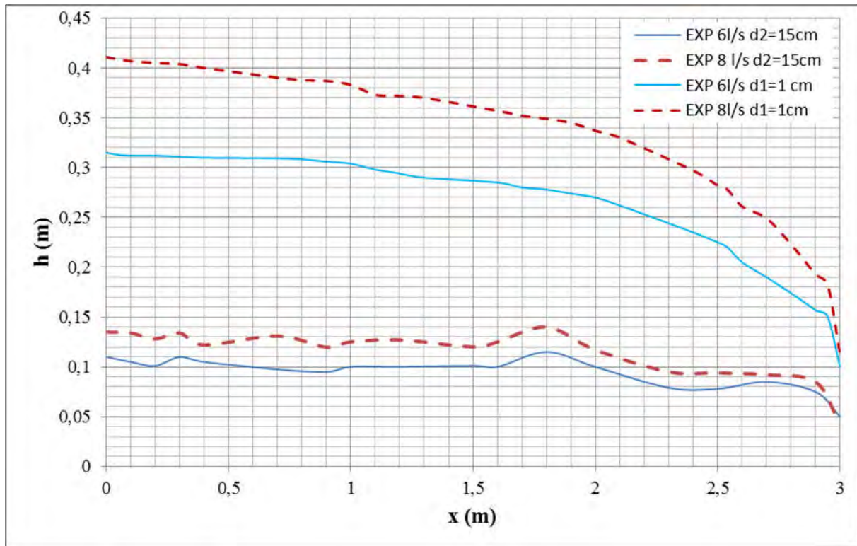
Figure I.3.16 : Ligne d'eau expérimentale pour les deux milieux étudiés ( d_1=1 cm et d_2=15 cm avec les deux débits 6 et 8 l/s
