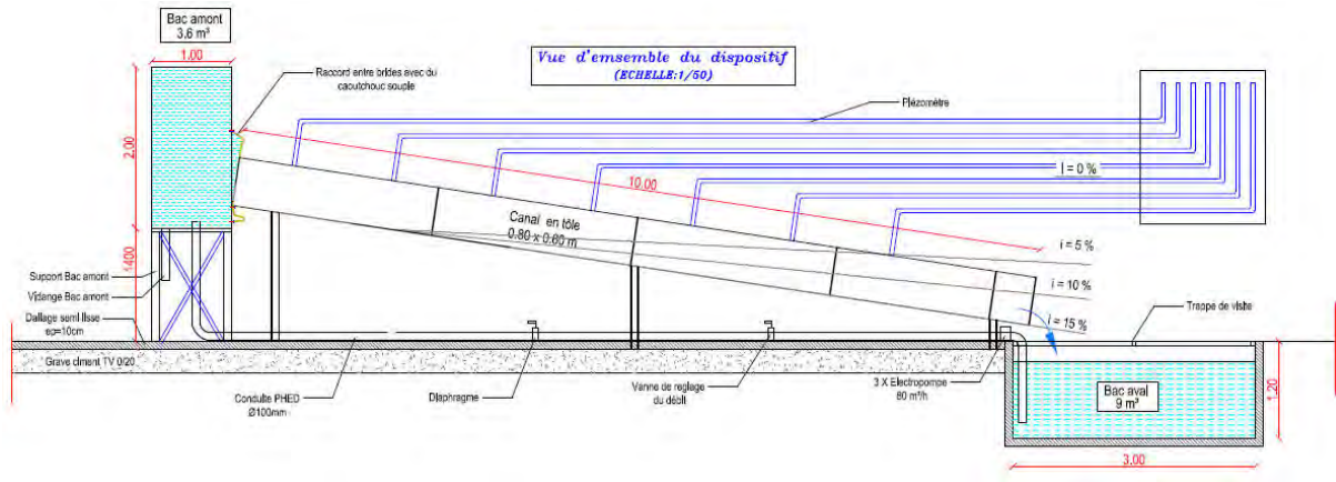
Figure I.2.4: Schéma du dispositif expérimental (vue de profil) – Grand canal de l'INAT
