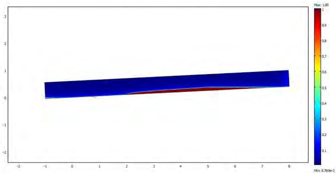
Figure I.4.31 : Comparaison ligne d'eau expérimentale et modélisée par COMSOL pour le débit Q=6 l/s en cas du milieu poreux constitué des cailloux de diamètre moyen d=15 cm
