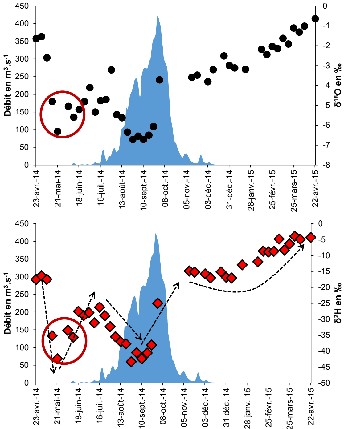
Figure 81 : Evolution de \delta^{18}\text{O} et de \delta^2\text{H} (‰) en fonction du débit ( \text{m}^3.\text{s}^{-1} ) à Kankan durant la période d'étude (2014 – 2015)
