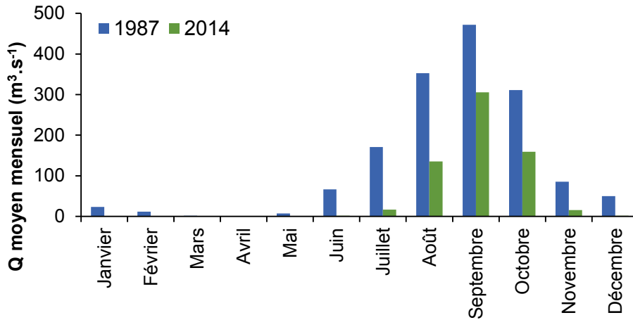
Figure 91 : Comparaison des débits mensuels entre les années 1987 et 2014
