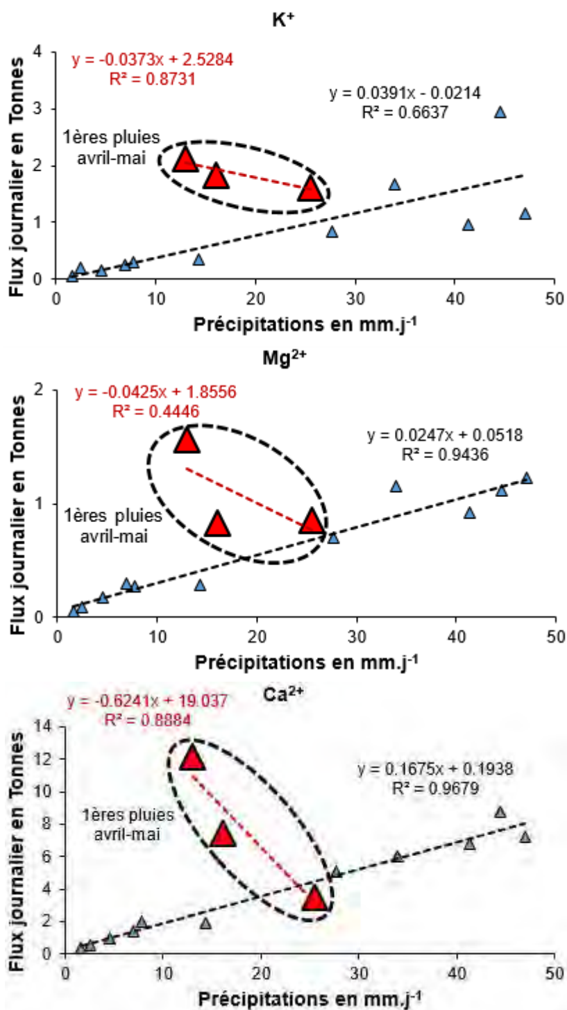
Figure 94 : Relation entre les flux journaliers d'éléments majeurs mesurés dans les eaux de pluies collectées à Kankan et ramenés à l'ensemble du bassin versant du Milo et l'intensité des précipitations mesurées à Kankan. Ces figures mettent en évidence le phénomène «wash-out» dans les eaux de pluies à Kankan lors des premiers évènements de l'année en avril et mai (triangles rouges)
