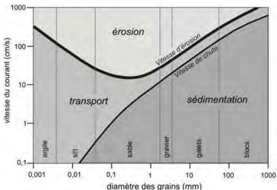
Figure 24 : Diagramme de Hjulström (1935) montrant le comportement des particules (érosion, transport, sédimentation) en fonction de leur taille et de la vitesse du courant
