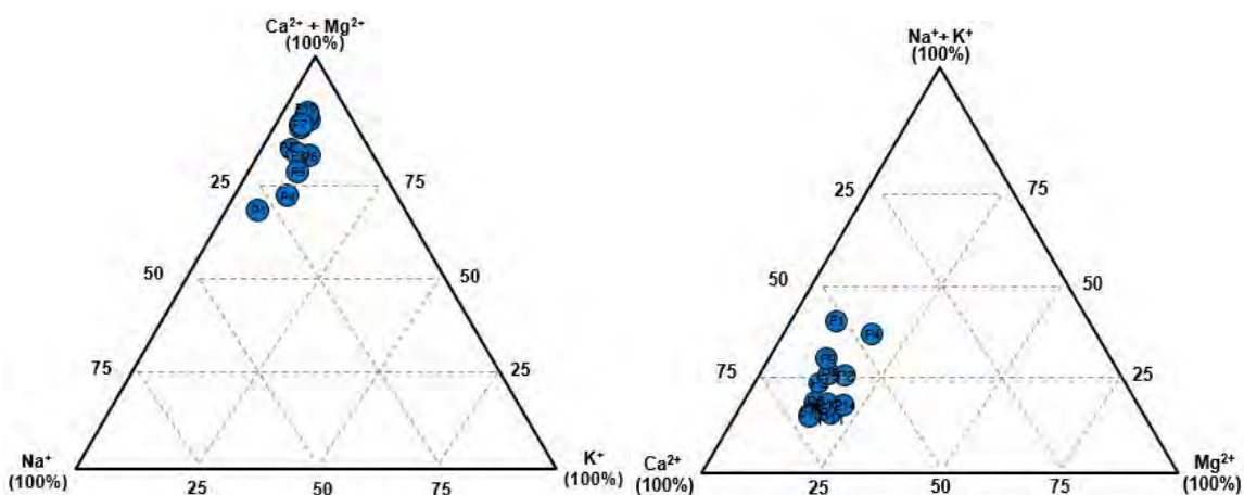
Figure 64 : Diagrammes ternaires de la composition des cations des eaux de pluie en 2015 à Kankan
