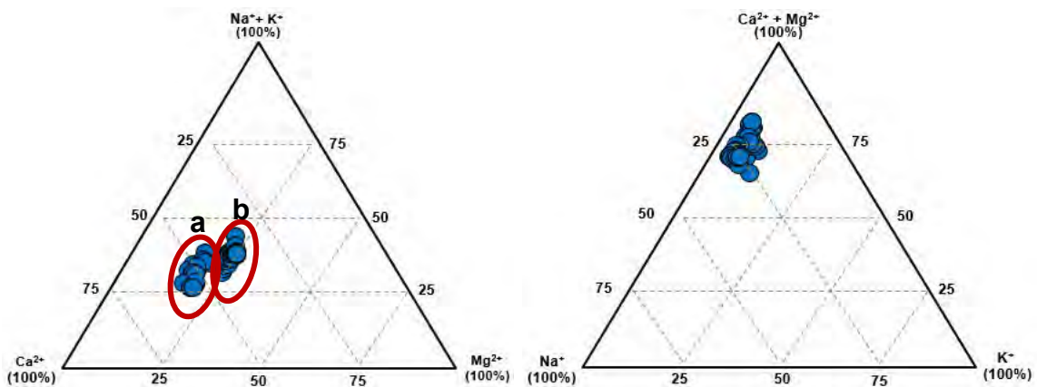
Figure 70 : Diagrammes ternaires de la composition des cations des eaux du Milo à la station aval de la ville de Kankan ; a montée des eaux, b décrue
