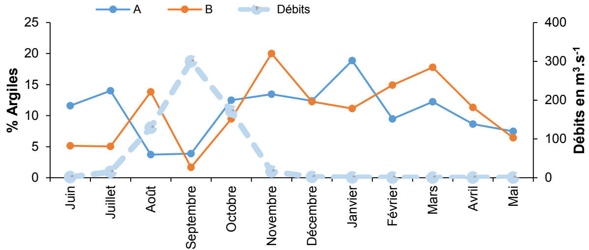
Figure 30 : Variations mensuelles des débits et des pourcentages d'argiles (<2 \mu m) dans les sédiments du Milo à Kankan. Stations amont A (ronds bleus) et aval B (ronds jaunes) de la ville de Kankan
