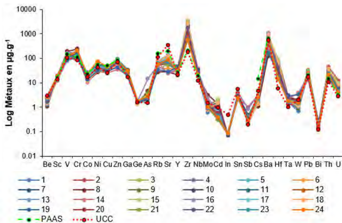
Figure 49 : Distribution des concentrations des éléments traces (ET) dans les sédiments du bassin versant du Milo (stations 1 à 24. Comparaison avec les teneurs dans le PAAS et l'UCC
