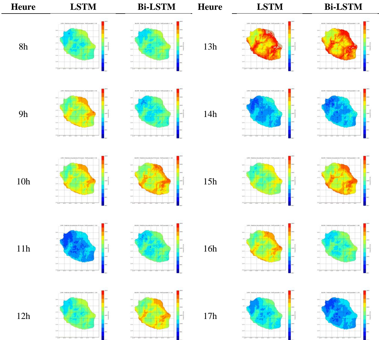
Figure A.16 Cartes de prédiction de production PV horaires sur une journée type de classe journalière 2 en 2018 pour les modèles LSTM et Bi-LSTM (de gauche à droite). L'échelle des couleurs de la production PV, comprise entre 4 kW et 28 kW
