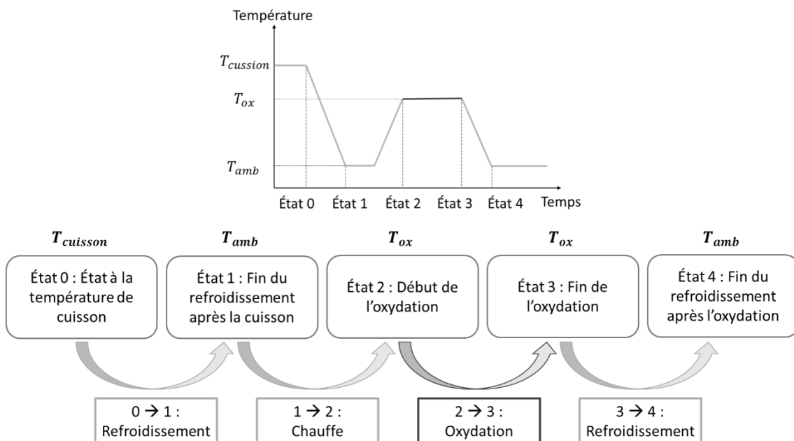
Figure 3-10. Présentation générale du modèle : schématisation des différentes étapes du processus d'oxydation simulées
