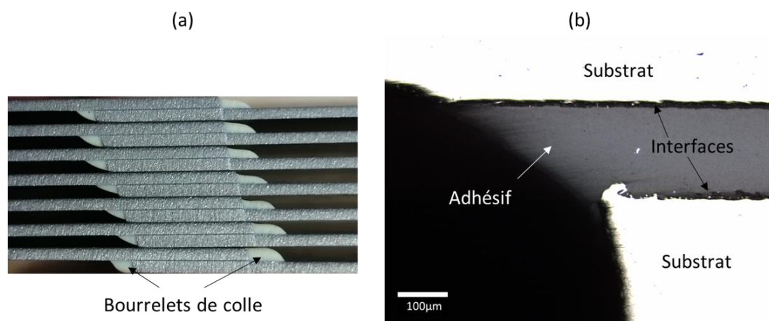
Figure 4-2. (a) Vue de la tranche d'un lot d'éprouvettes après découpe ; (b) Vue agrandie au microscope optique du bord de la zone de recouvrement d'une éprouvette après retrait du bourrelet de colle et polissage
