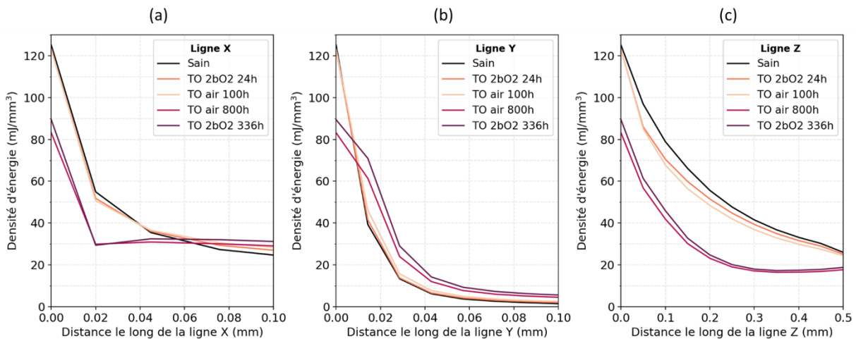
Figure 5-32. Evolution de la densité d'énergie suivant les 3 lignes (ligne X en (a), ligne Y en (b) et ligne Z en (c)) définies sur la Figure 5-31 au moment de l'amorçage pour les cas sain et thermo-oxydés (TO)
