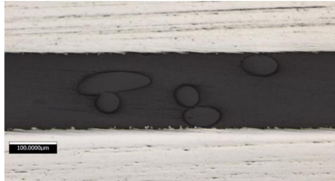
Figure A-2. Image au microscope optique du côté du joint collé avec le support en polyamide
