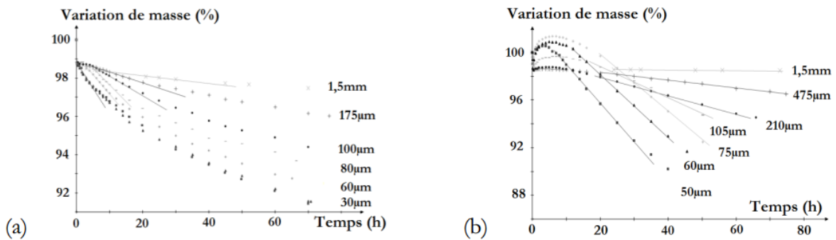
Figure 1-17. Courbes de suivi de masse d'échantillons de différentes épaisseurs au cours d'une oxydation (a) à 200°C sur une résine de type époxy et (b) à 240°C sur une résine de type bismaléimide (Colin, 2000)
