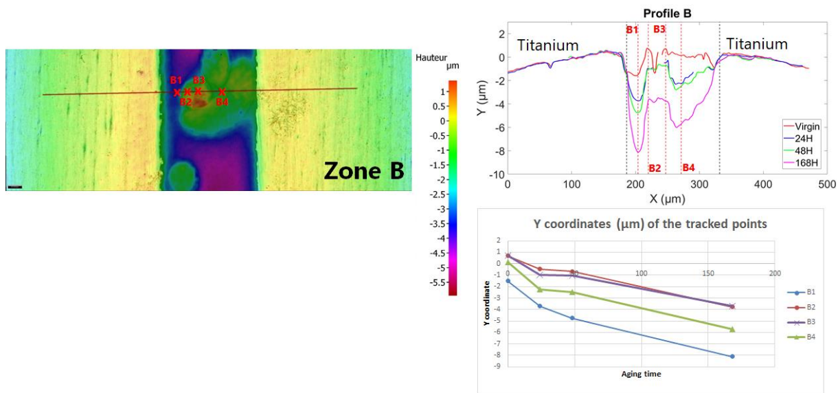
Figure A-7. Mesure du retrait et évolution du retrait avec la durée d'oxydation - zone B : effet du support en polyamide
