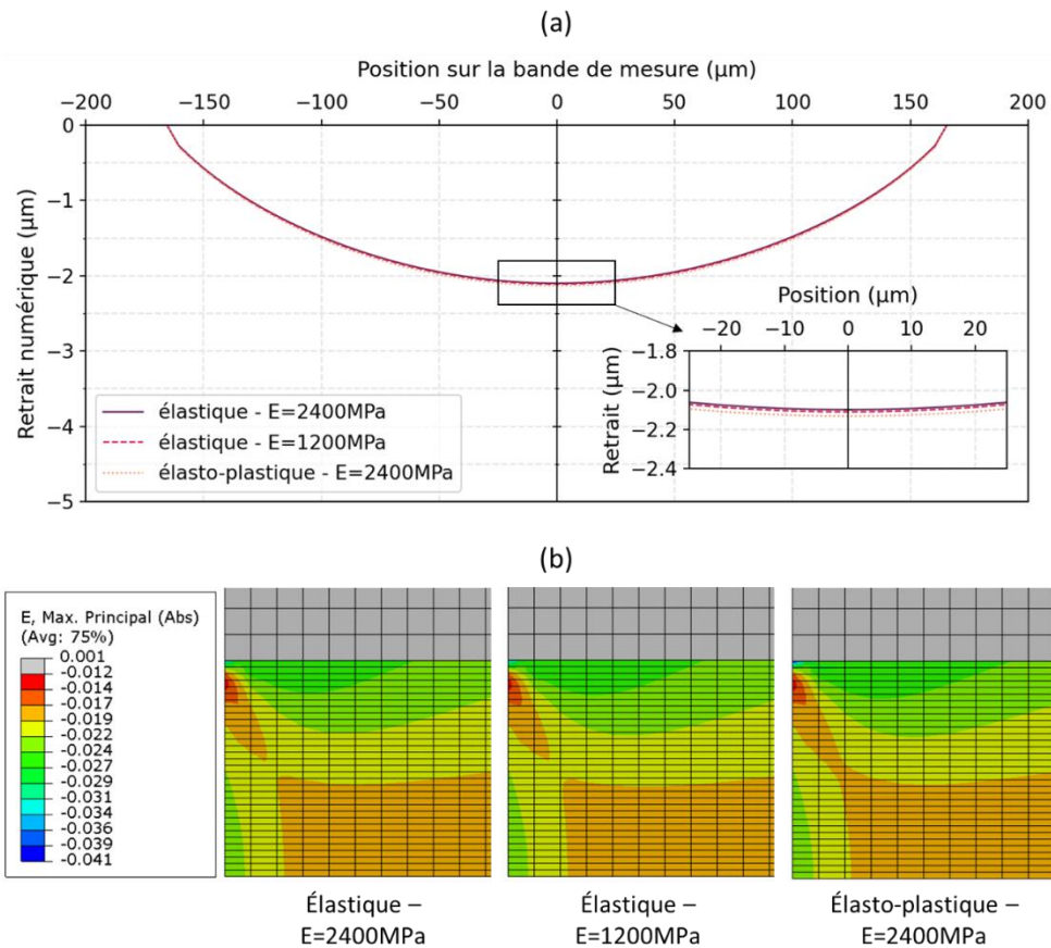
Figure 3-9. Comparaison (a) des profils de retrait initial dans l'assemblage collé et (b) des champs de déformation maximale pour différentes propriétés mécaniques de l'adhésif définies dans le modèle
