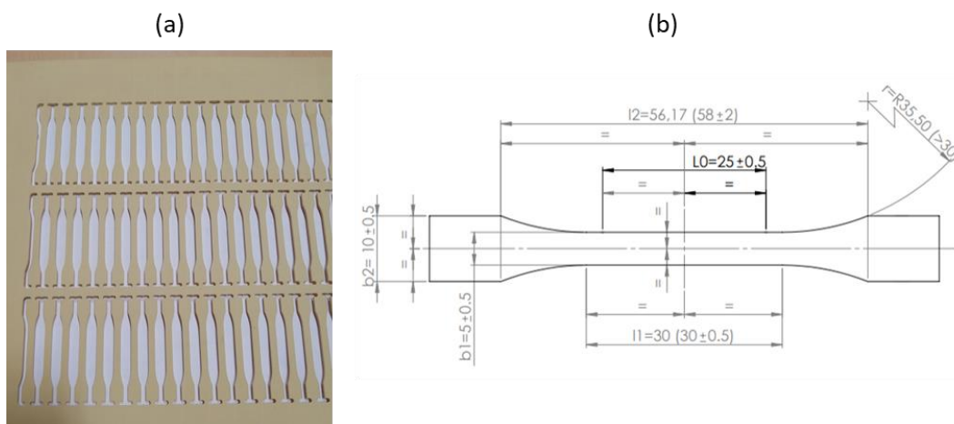
Figure 2-5. (a) Eprouvettes haltères découpées dans une des plaques d'adhésif ; (b) Dimensions des éprouvettes haltères suivant la norme ISO 527-2
