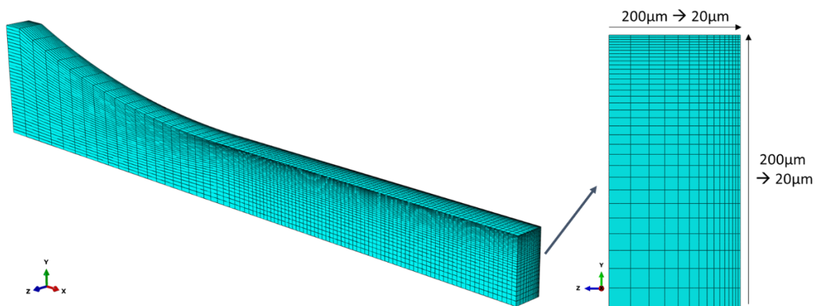
Figure 5-6. Maillage de l'éprouvette de traction modélisée
