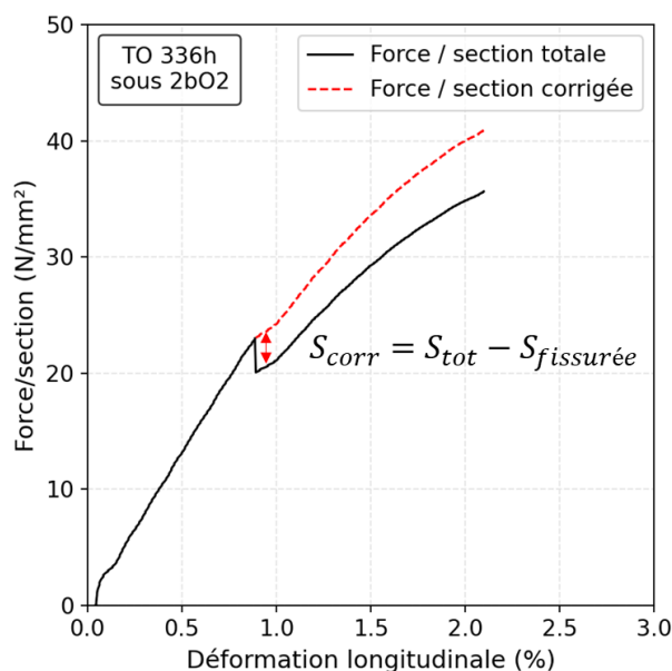
Figure 5-5. Comparaison de la courbe résultante de traction d'une éprouvette thermo-oxydée (TO) sous 2bar d'oxygène pendant 336h avec une courbe où la section est corrigée au cours de l'essai
