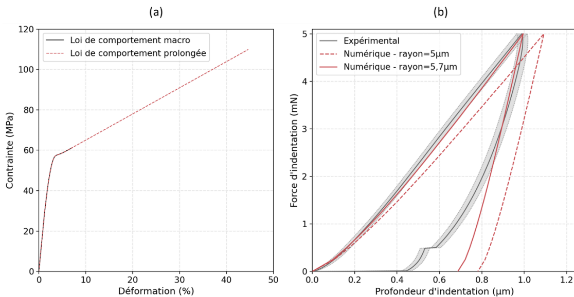
Figure 2-17. (a) Loi de comportement macroscopique prolongée ; (b) Comparaison des courbes d'indentation sur adhésif massif sain expérimentale et numériques pour deux rayons de la pointe de l'indenteur
