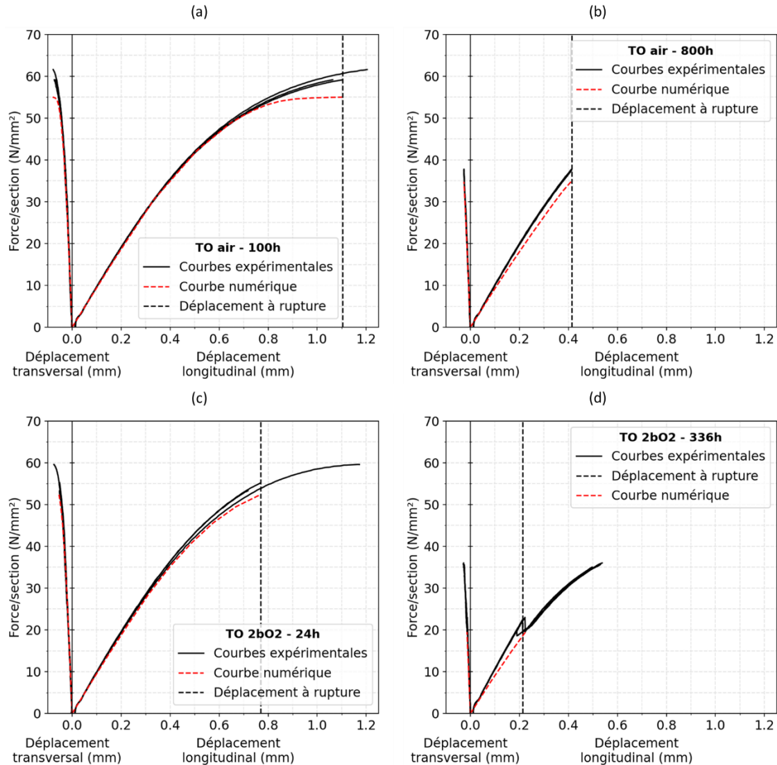
Figure 5-13. Comparaison entre les courbes résultantes de l'essai de traction expérimentales et numériques pour des éprouvettes d'adhésif massif thermo-oxydées (TO) à 150°C sous air (a) pendant 100h, (b) pendant 800h et sous 2bar d'oxygène (c) pendant 24h, (d) pendant 336h
