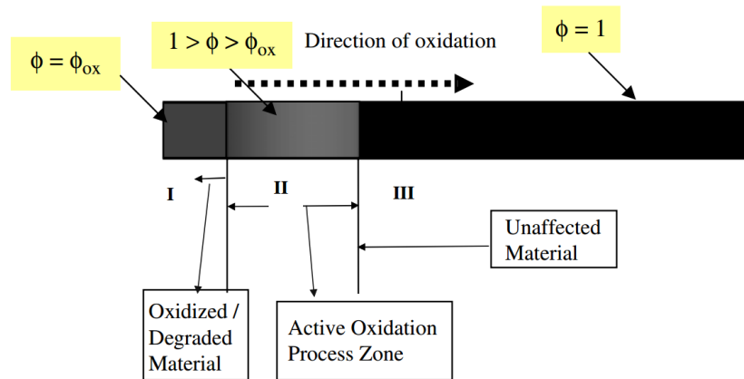
Figure 1-27. Schématisation de la couche oxydée en trois zones (Tandon et al., 2006)
