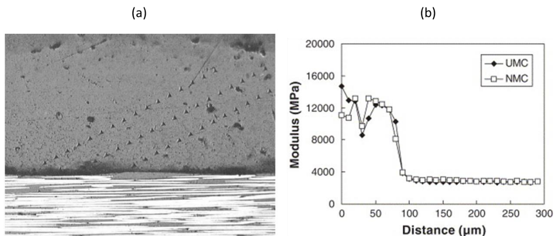
Figure 1-11. (a) Visualisation des séries d'indentation réalisées dans un assemblage collé ; (b) Evolution du module d'indentation au sein du substrat puis dans l'adhésif (Zheng and Ashcroft, 2005)
