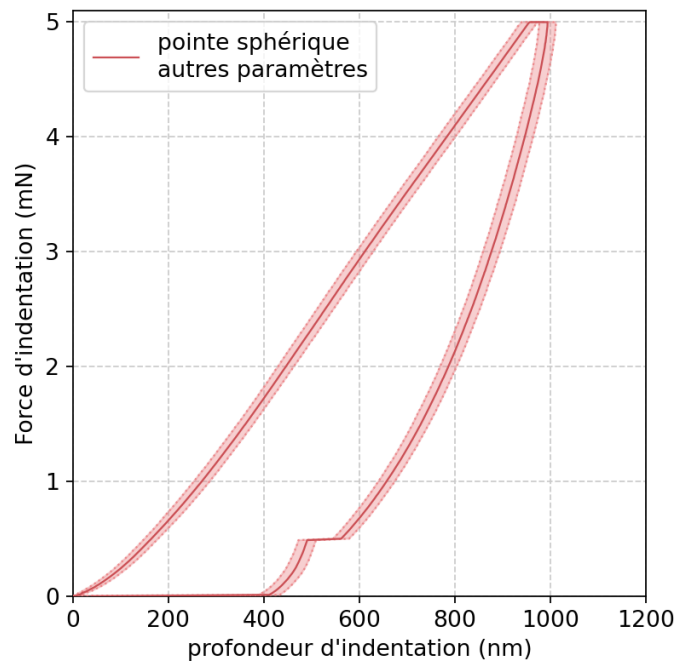
Figure C-3. Courbe d'indentation obtenue avec la pointe sphérique – paramètres différents d'indentation
