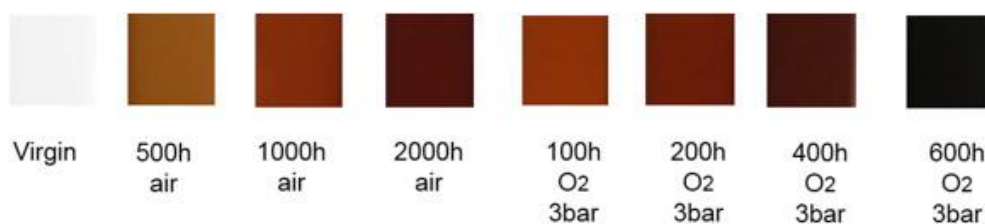
Figure 1-16. Echantillons de PR520, sain et oxydés dans différents environnements (Pecora et al., 2016)
