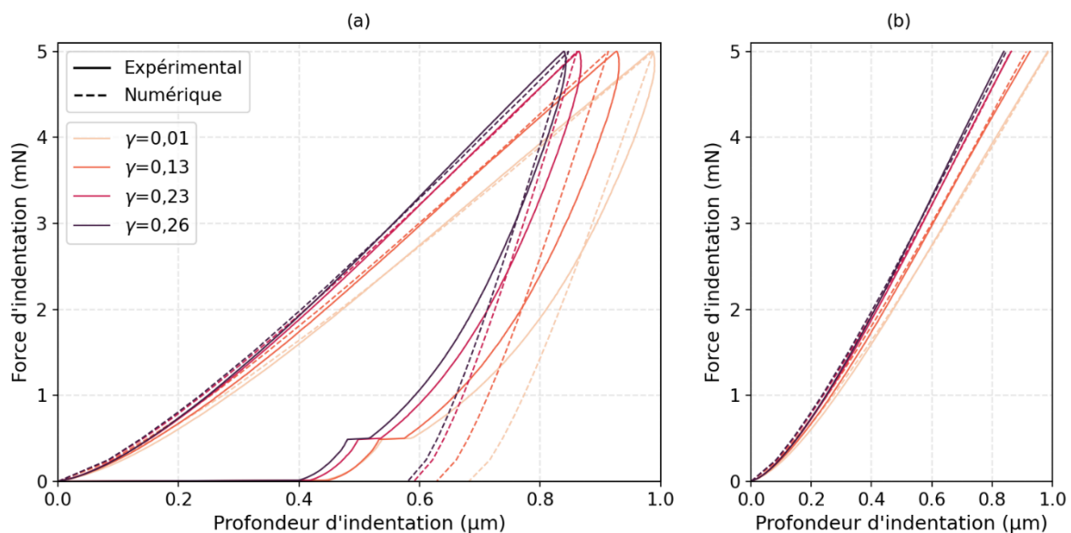
Figure 2-26. Comparaison des courbes d'indentation dans la couche oxydée expérimentales et numériques (a) sur le cycle total et (b) sur la phase de charge uniquement
