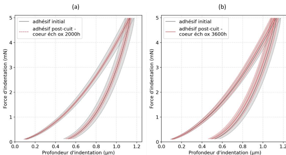
Figure 2-20. Comparaison des courbes d'indentation sur l'adhésif initial et l'adhésif à cœur d'échantillon oxydés à 150°C sous air à pression atmosphérique pendant : (a) 2000h et (b) 3600h
