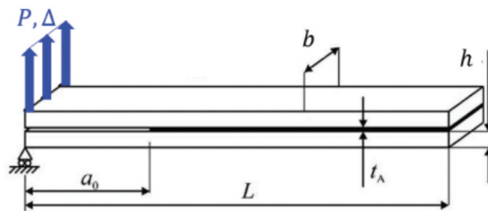
Figure 1-5. Représentation schématique d'une éprouvette DCB avec une fissure initiale de longueur a_0 sous un chargement P ou un déplacement \Delta (Budzik et al., 2022)
