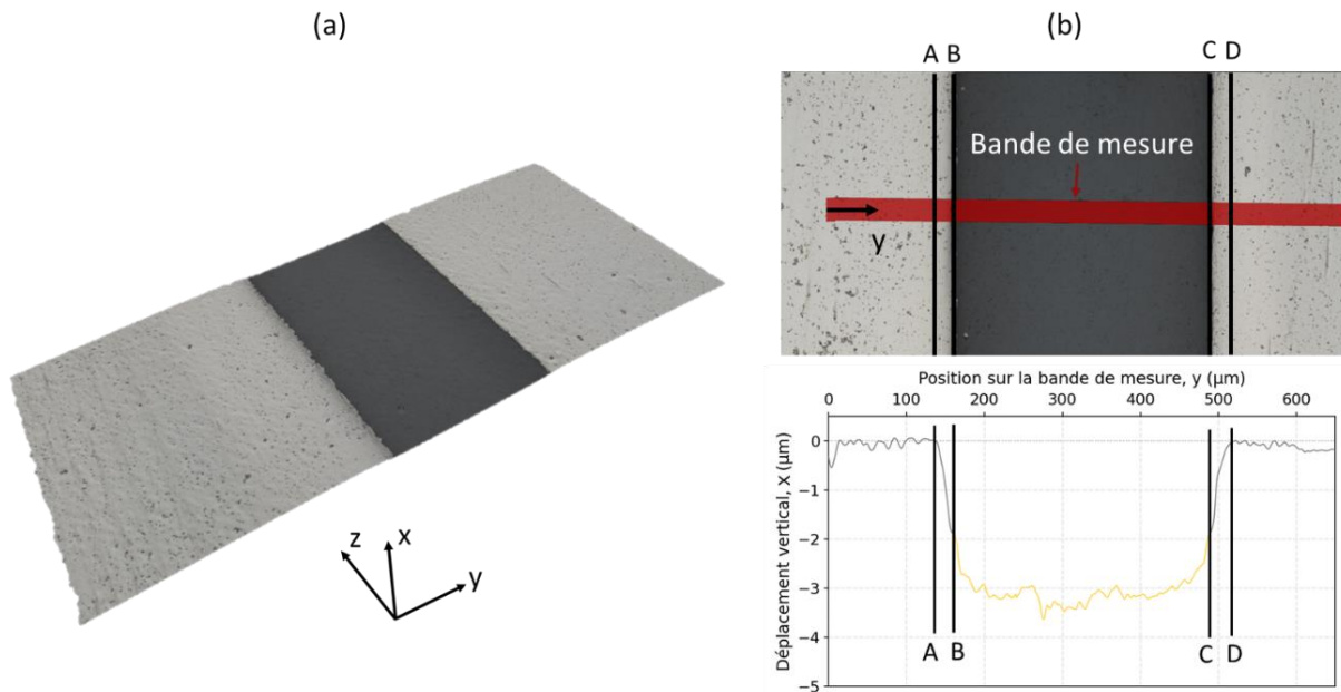
Figure 3-5. (a) Acquisition de la surface 3D de l'assemblage collé ; (b) Mesure et post-traitement du retrait au sein de l'assemblage collé
