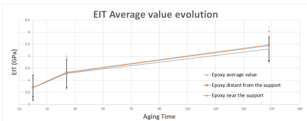
Figure A-9. Evolution du module EIT adimensionné en fonction de la durée de vieillissement dans la matrice : valeur moyenne et valeurs proches et loin des fibres
