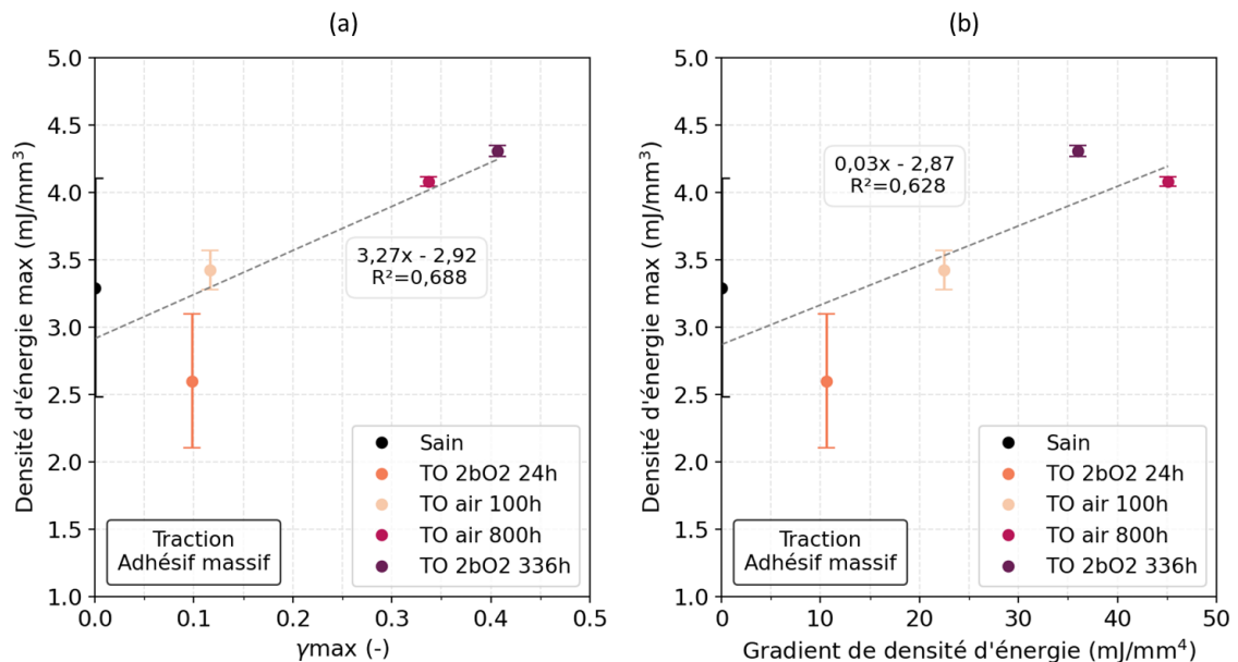
Figure 5-37. Comparaison de l'évolution de la densité d'énergie maximale au moment de l'amorçage de fissure dans l'adhésif massif sollicité en traction en fonction (a) de \gamma_{max} et (b) du gradient de densité d'énergie
