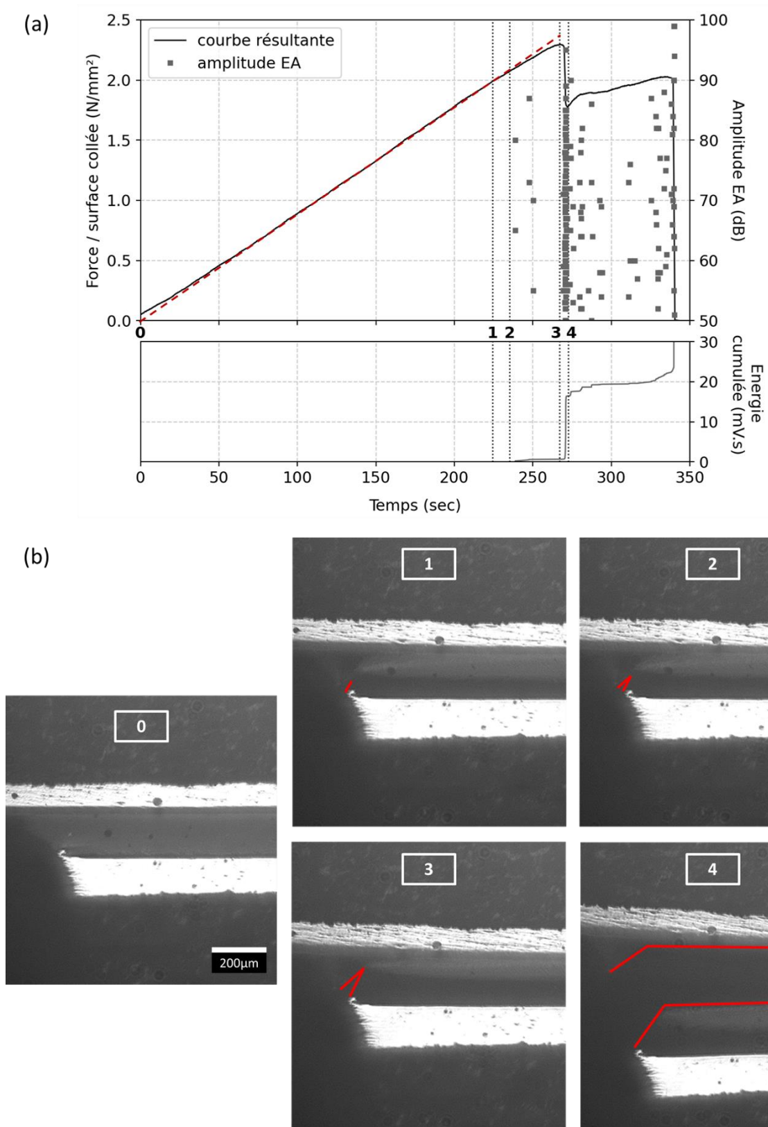
Figure 4-9. (a) Synchronisation de la courbe résultante de l'essai de flexion 3 points sur éprouvette saine avec les données d'émission acoustique en termes d'amplitude et d'énergie cumulée et identification des étapes de la fissuration avec en (b) les observations au microscope QUESTAR correspondantes
