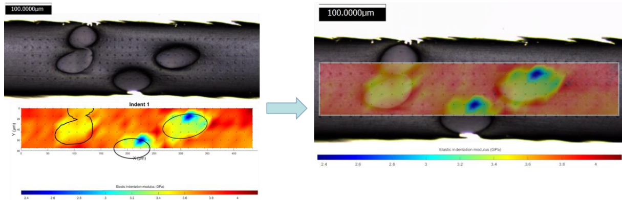
Figure A-4. Cartographie des modules élastiques d'indentation (EIT) superposée aux empreintes dans un joint collé supporté non vieilli
