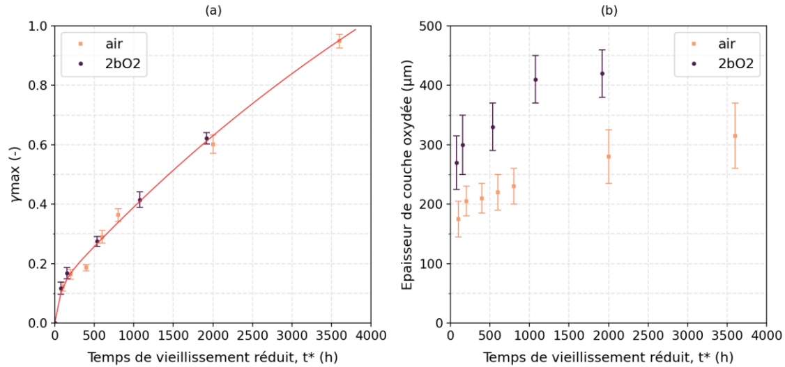
Figure 2-23. Comparaison des vieillissements sous air et sous 2bar d'O 2 en fonction d'un temps de vieillissement réduit : (a) \gamma_{max} ; (b) épaisseur de couche oxydée
