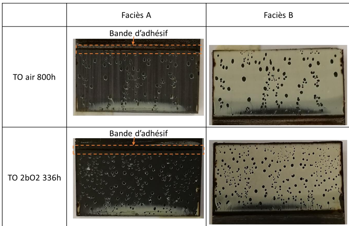
Figure 4-14. Faciès de rupture d'éprouvettes SLJ vieilles par thermo-oxydation (TO) après essai de flexion 3 points. Se référer à la Figure 4-11 pour la définition des faciès A et B
