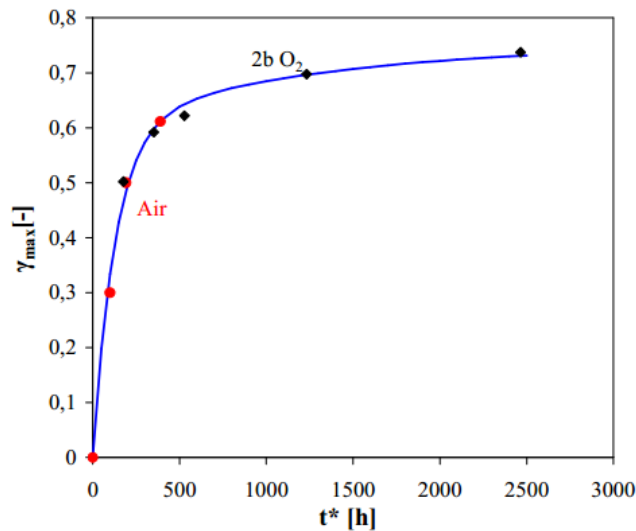
Figure 1-32. "Courbe maîtresse" de vieillissement à pression atmosphérique traçant l'évolution de \gamma_{max} jusqu'à 2500h pour une température d'oxydation de 150°C
