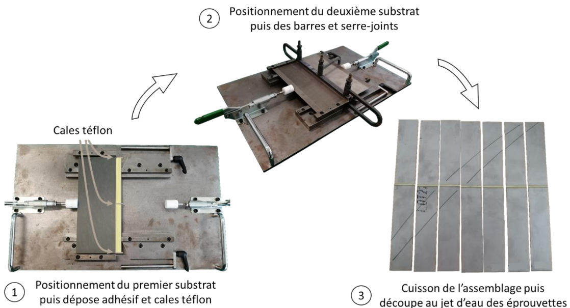
Figure 4-1. Étapes de fabrication des éprouvettes à simple recouvrement (Single Lap Joint ou SLJ)
