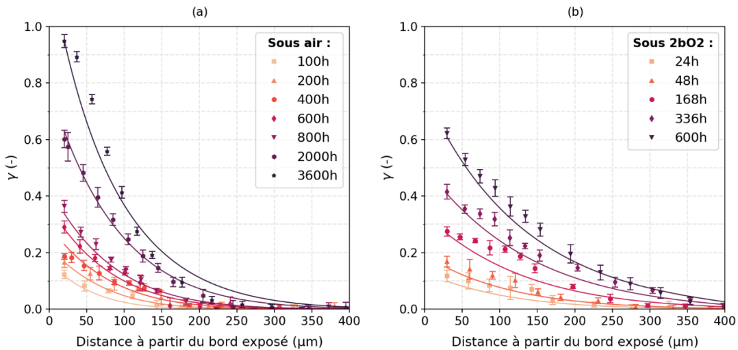
Figure 2-24. Comparaison des profils du paramètre \gamma expérimentaux et numériques (a) sous air et (b) sous 2bar d'O 2
