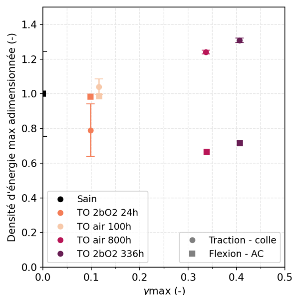
Figure 5-35. Comparaison de l'évolution de la densité d'énergie maximale adimensionnée par la valeur saine en fonction de \gamma_{max} entre les essais de traction sur l'adhésif massif et les essais de flexion 3 points sur l'assemblage collé
