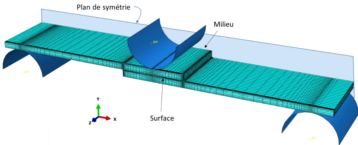
Figure 5-18. Modèle numérique de flexion 3 points sur assemblage collé et maillage de l'éprouvette SLJ
