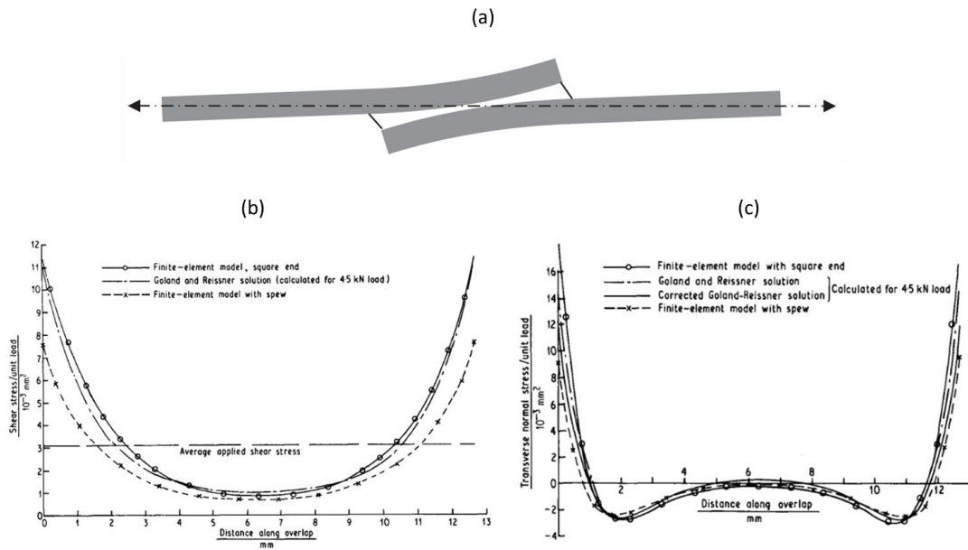
Figure 1-6. (a) Schématisation du mouvement de flexion induit par le désalignement des substrats lors du chargement d'un joint à simple recouvrement (SLJ) (da Silva, 2011) ; Distribution des contraintes de cisaillement (b) et de pelage (c) le long de la zone de recouvrement (Adams and Peppiatt, 1974)
