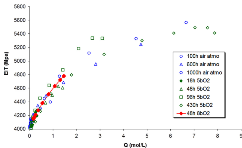
Figure 1-31. Corrélation entre le module EIT et la concentration en produits d'oxydation (Q) pour des vieillissements sous différentes pressions partielles d'oxygène (Grandidier et al., 2015)
