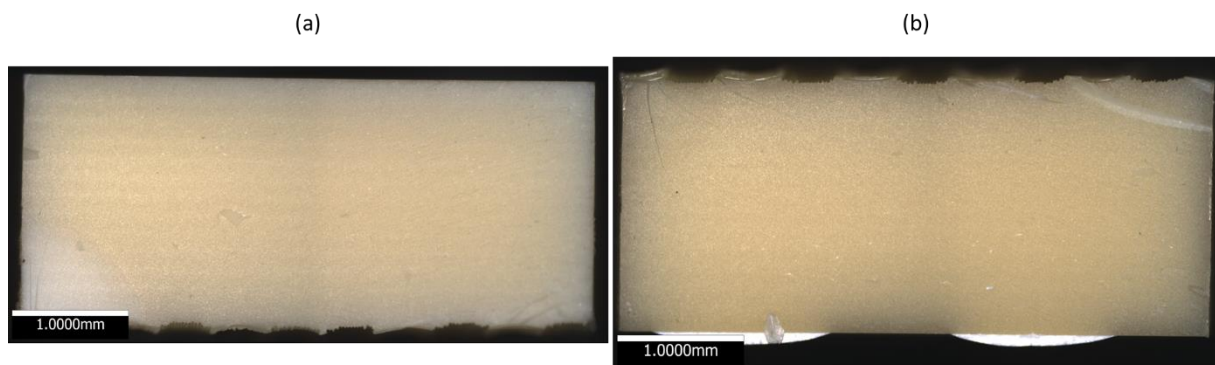
Figure 2-10. Observation au microscope optique des faciès de rupture d'éprouvettes testées en traction à 1mm/min à (a) 100°C et (b) 150°C
