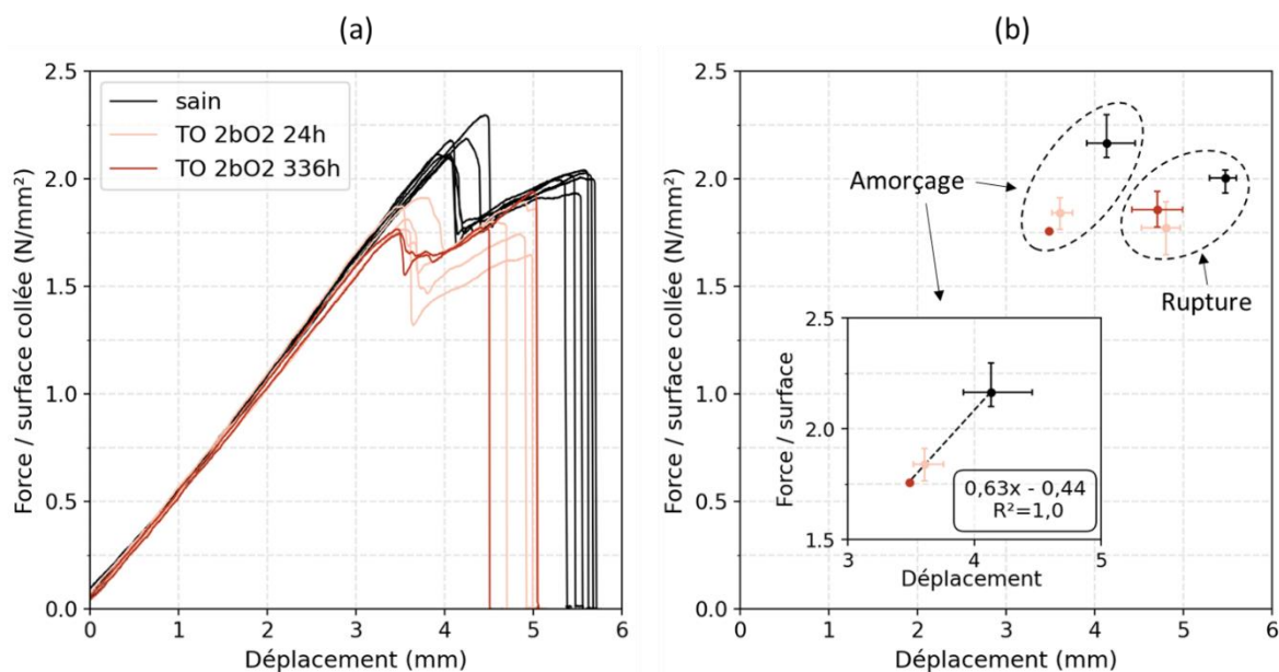
Figure 4-16. Comparaison entre cas sains et vieillis à 150°C sous 2bar d'O 2 pendant différentes durées en (a) des courbes résultantes des essais de flexion 3 points réalisés sur éprouvettes SLJ et en (b) des forces rapportées à la surface moyennes et des déplacements moyens à l'amorçage et à la rupture
