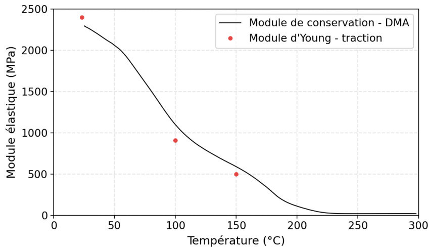
Figure 2-8. Comparaison des modules élastiques - DMA / traction
