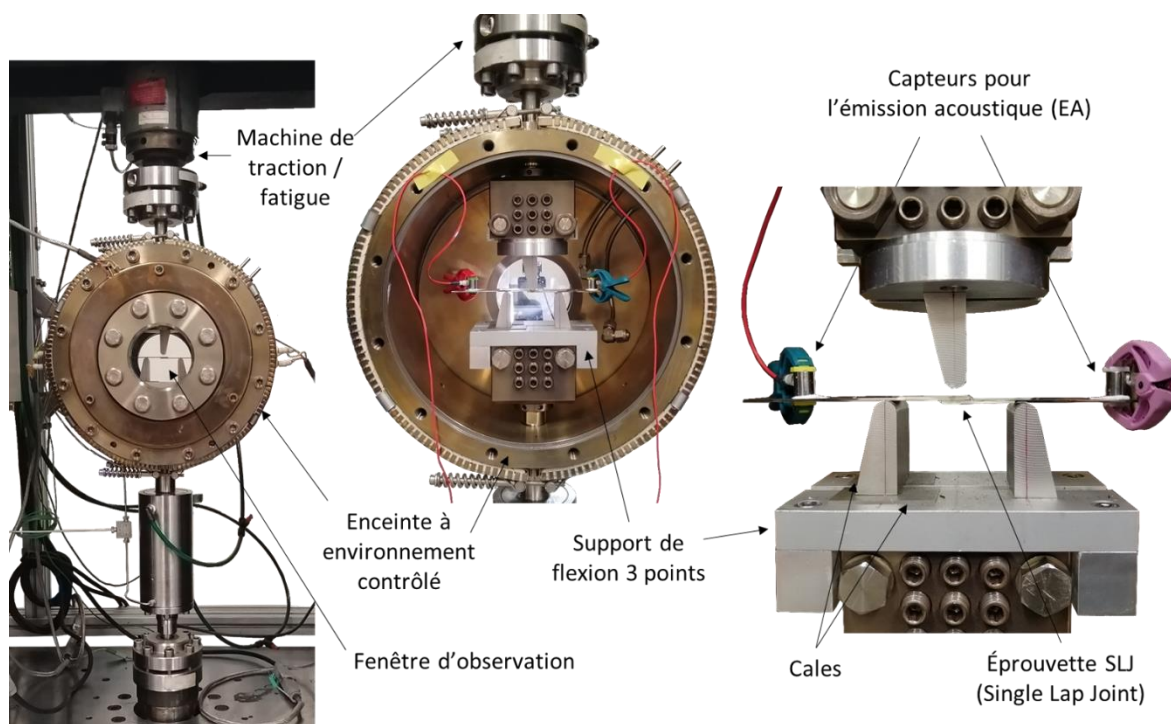
Figure 4-3. Présentation du montage multi-instrumenté avec la machine d'essai, l'enceinte à environnement contrôlé, le support de flexion 3 points, l'éprouvette SLJ et l'instrumentation pour l'émission acoustique
