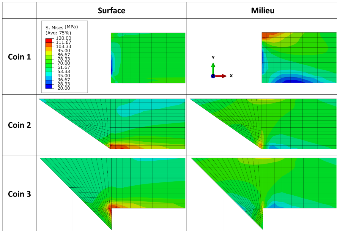
Figure 5-22. Comparaison pour les trois configurations au bord du joint de colle (coin 1, 2 et 3) des champs de contrainte de Von Mises à l'instant de l'amorçage sur la surface et au milieu d'une éprouvette SLJ saine sollicitée en flexion 3 points
