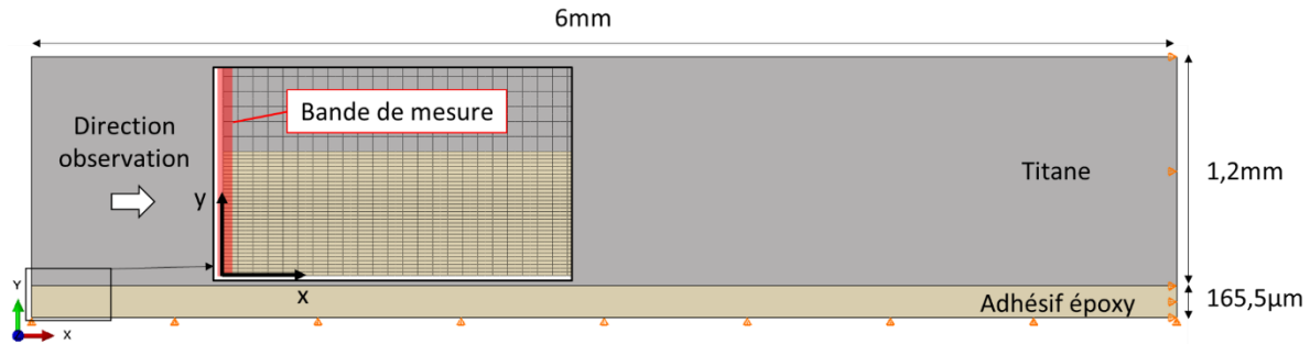
Figure 3-7. Modèle éléments finis 2D du joint collé pour simuler le retrait
