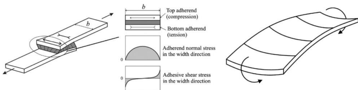
Figure 1-7. Contraintes transverses dans le joint à simple recouvrement (SLJ) dues à la courbure anticlastique des substrats schématisée sur l'image de droite (L. F. M. da Silva et al., 2009)
