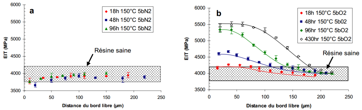
Figure 1-24. Distribution spatiale des modules élastiques d'indentation (EIT) mesurés sur des échantillons vieillis pendant différentes durées à 150°C sous 5bar (a) d'azote et (b) d'oxygène (Lafarie-Frenot et al., 2010)
