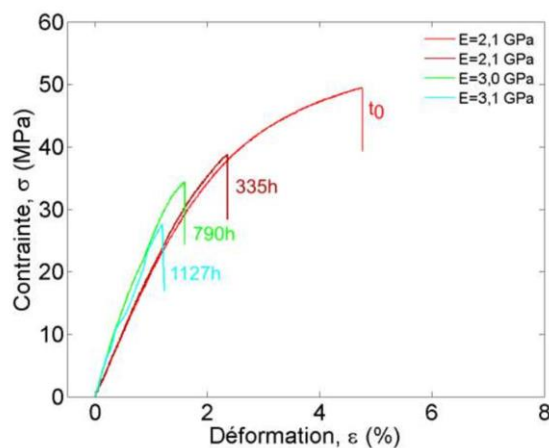
Figure 1-20. Courbes de traction sur des films de résine époxy pour différentes durées de vieillissement à 120°C (Delozanne, 2018)
