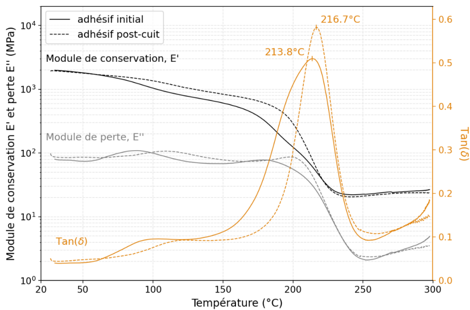
Figure 2-31. Comparaison des courbes DMA entre l'adhésif initial et l'adhésif post-cuit sous N_2 à 150^\circ C pendant 100h
