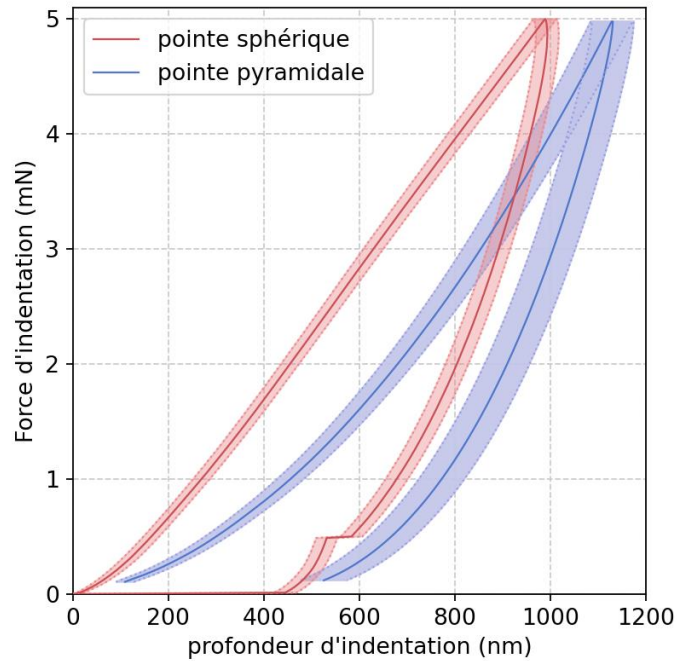
Figure C-2. Comparaison des réponses en indentation pour la machine à la pointe sphérique et celle à la pointe pyramidale
