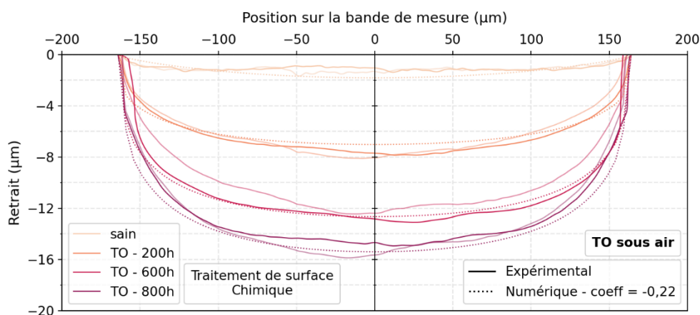
Figure 3-19. Comparaison des profils de retraits expérimentaux et numériques pour une thermo-oxydation (TO) à 150^{\circ}\text{C} sous air avec un traitement de surface chimique
