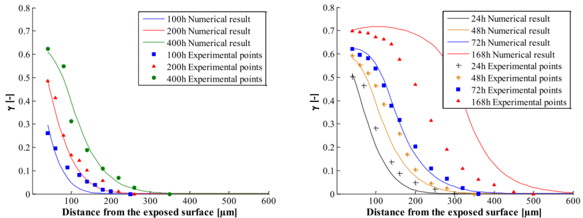
Figure 1-30. Comparaison des profils expérimentaux et numériques du paramètre \gamma pour des résines vieilles sous air à pression atmosphérique (a) et sous 2bar d'oxygène (b) à 150°C (Gigliotti et al., 2016c)
