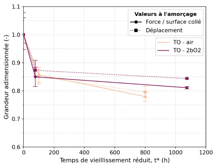
Figure 4-17. Evolution en fonction du temps réduit des grandeurs (force/surface collée et déplacement) à l'amorçage adimensionnées par la valeur saine pour les deux environnements considérés (air et 2bar d'O 2 )
