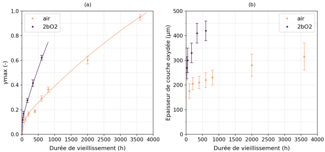
Figure 2-22. Comparaison des vieillissements sous air et sous 2bar d'O 2 : (a) \gamma_{max} ; (b) épaisseur de couche oxydée
