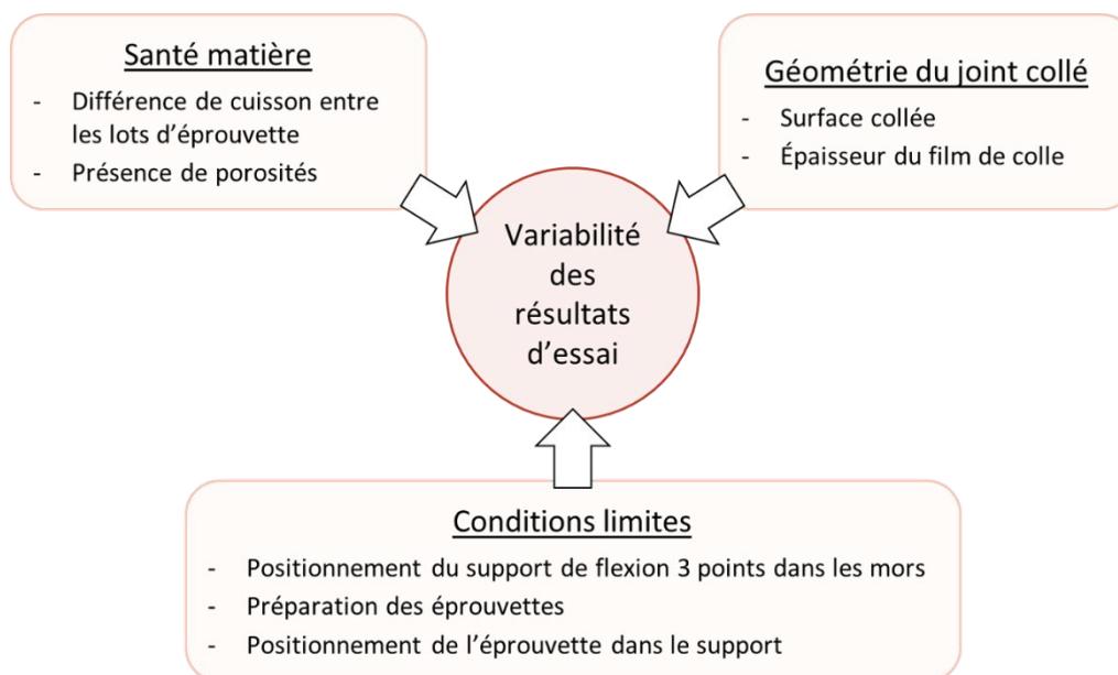
Figure 4-6. Schématisation des sources de variabilité des résultats d'essai
