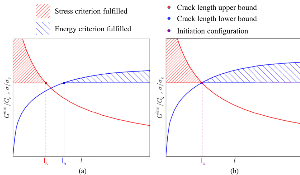
Figure 1-13. Evolution du rapport entre la contrainte appliquée et la résistance ( \sigma/\sigma_c ) et du rapport entre le taux de restitution d'énergie incrémental et la ténacité ( G^{inc}/G_c ) en fonction de la longueur à l'amorçage (Doitrand et al., 2020)
