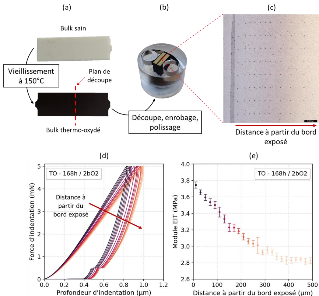
Figure 2-18. Illustration des étapes suivies pour les essais d'ultra-micro-indentation sur échantillon thermo-oxydé : (a) vieillissement de l'échantillon ; (b) échantillon découpé, enrobé et poli ; (c) série d'empreintes d'indentation dans la couche oxydée d'un échantillon ; (d) courbes d'indentation moyennes ; (e) évolution du module élastique d'indentation EIT le long de la couche oxydée
