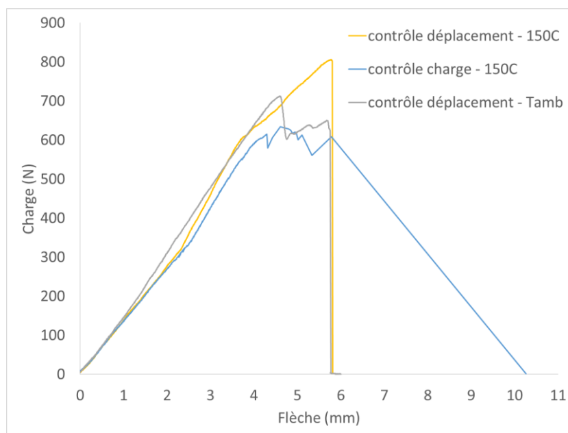
Figure E-1. Comparaison des réponses mécaniques d'éprouvettes SLJ sollicitées en flexion 3 points à différentes températures et différents asservissements
