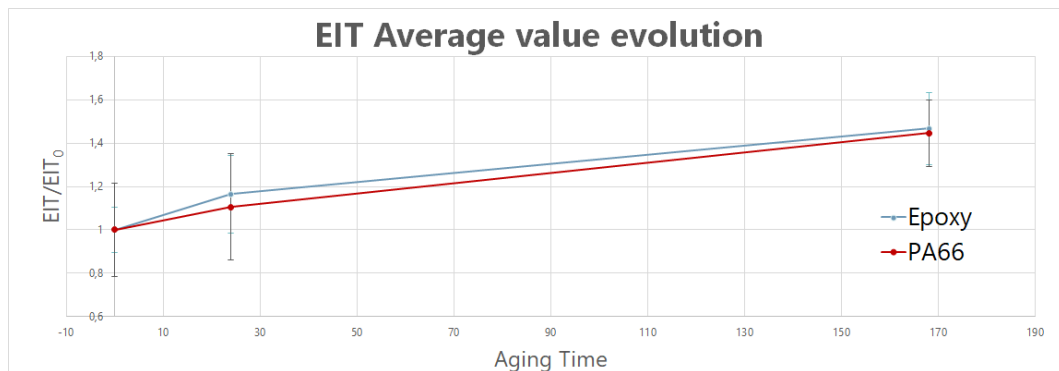
Figure A-8. Evolution du module EIT adimensionné en fonction de la durée de vieillissement dans la matrice et dans les fibres
