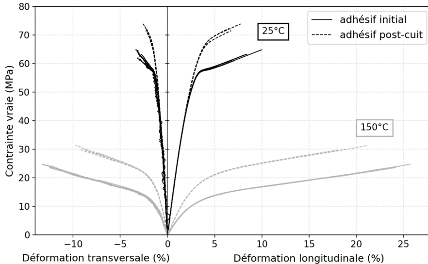
Figure 2-32. Comparaison des courbes de traction monotones à 1\text{mm/min} réalisés à 25^\circ C et 150^\circ C entre l'adhésif initial et l'adhésif post-cuit sous N_2 à 150^\circ C pendant 100h
