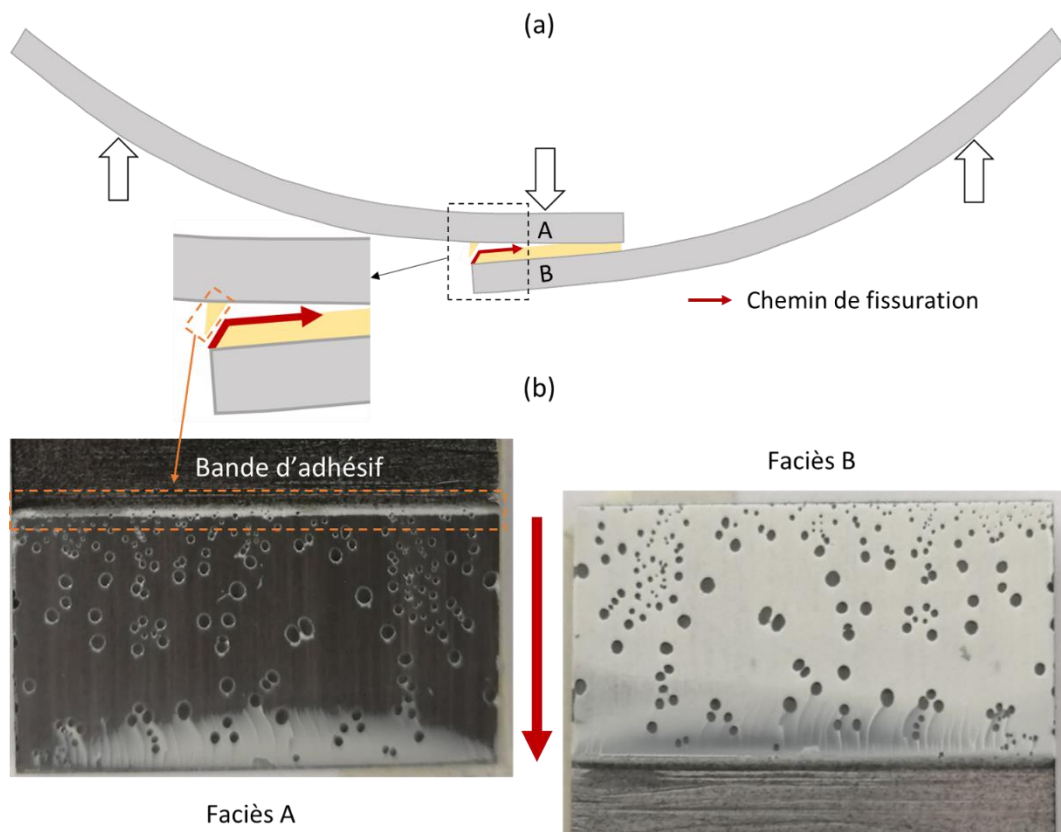
Figure 4-11. (a) Schématisation du mode de rupture de l'assemblage en flexion 3 points ; (b) Faciès de rupture d'une éprouvette SLJ saine après l'essai de flexion 3 points
