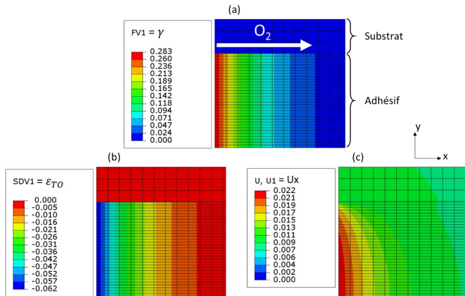
Figure 3-17. Champs (a) du paramètre \gamma , (b) des déformations chimiques dues à la thermo-oxydation et (c) des retraits associés aux déformations au sein de l'assemblage collé obtenus à l'issue du calcul avec le modèle de thermo-oxydation
