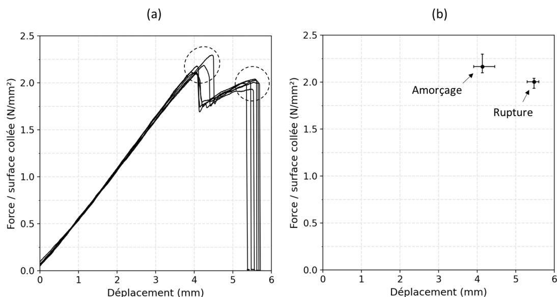
Figure 4-8. (a) Courbes résultantes de l'ensemble des essais de flexion 3 points réalisés sur éprouvettes SLJ saines ; (b) Identification des forces rapportées à la surface moyennes et des déplacements moyens à l'amorçage et à la rupture
