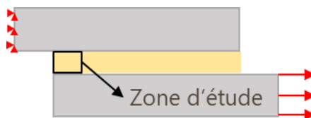
Figure D-2. Exemple de configuration étudiée : géométrie type SLJ avec un chargement de type cisaillement
