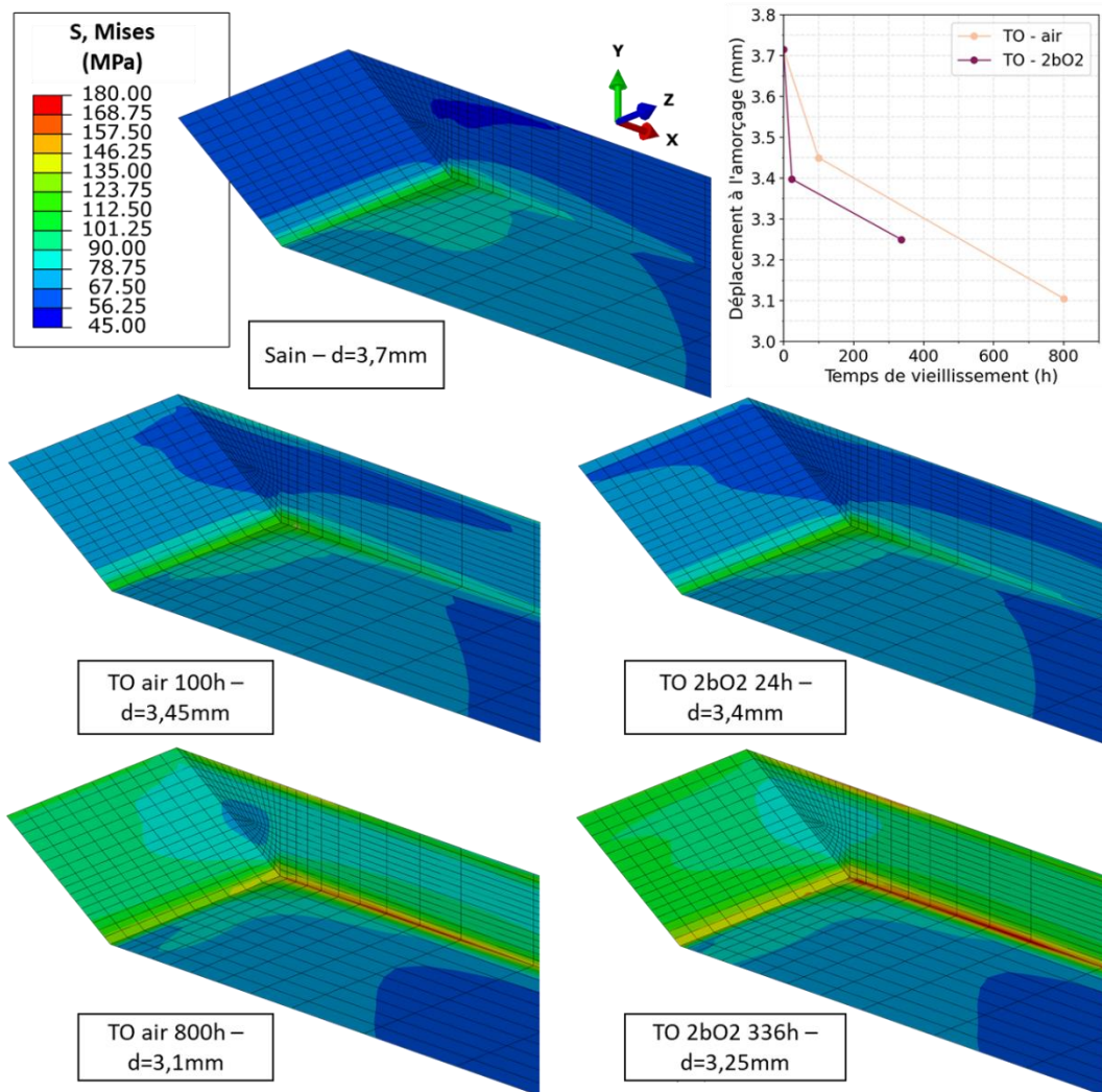
Figure 5-29. Distribution des contraintes de Von Mises à l'instant d'amorçage pour tous les cas étudiés (sain et vieillis) avec l'évolution du déplacement à l'amorçage en fonction de la durée d'oxydation
