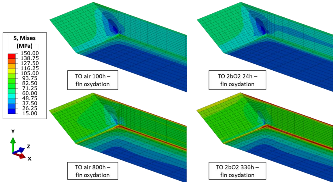
Figure 5-26. Distribution des contraintes de Von Mises dans la zone d'étude de l'adhésif confiné à l'issue de l'oxydation pour les quatre conditions de vieillissement étudiées : sous air pendant 100h et 800h et sous 2bar d'O 2 pendant 24h et 336h
