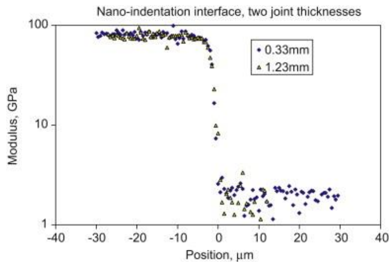
Figure 1-12. Variation du module d'indentation au niveau de l'interface d'un assemblage aluminium/époxy pour différentes épaisseurs (Davies et al., 2009)
