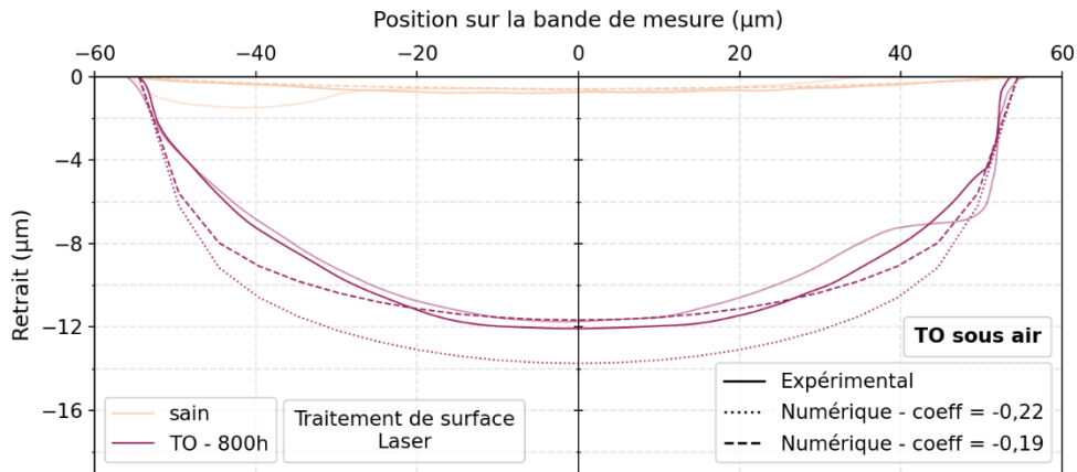
Figure 3-20. Comparaison des profils de retraits expérimentaux et numériques pour une thermo-oxydation (TO) à 150°C sous air avec un traitement de surface laser
