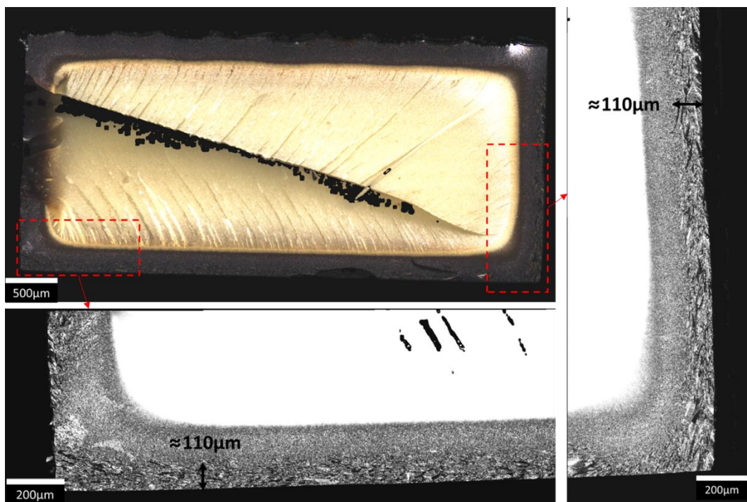
Figure 5-4. Observation au microscope Alicona du faciès de rupture d'une éprouvette vieillie à 150°C sous 2bar d'oxygène pendant 336h et identification d'une bande pré-fissurée
