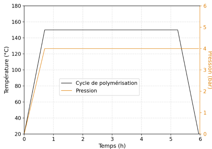
Figure 2-2. Cycle de polymérisation des plaques d'adhésif épaisses
