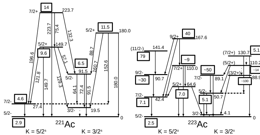
FIGURE 3 : Comparaison entre le schéma de niveaux proposé pour le noyau ^{221}\text{Ac} et le schéma de niveaux du noyau ^{223}\text{Ac} . Les facteurs d'empêchement sont indiqués dans les boîtes en gras.
