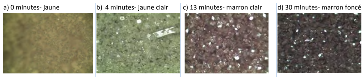
Figure 10. Changements de couleur de la phase solide au cours de la réaction. Conditions expérimentales: \text{AgNO}_3/\text{K}_2\text{S}_2\text{O}_8 (1: 1), \text{KH}_2\text{PO}_4/\text{K}_2\text{HPO}_4 (0,1: 0,1 M), 100 ° C, 30 minutes
