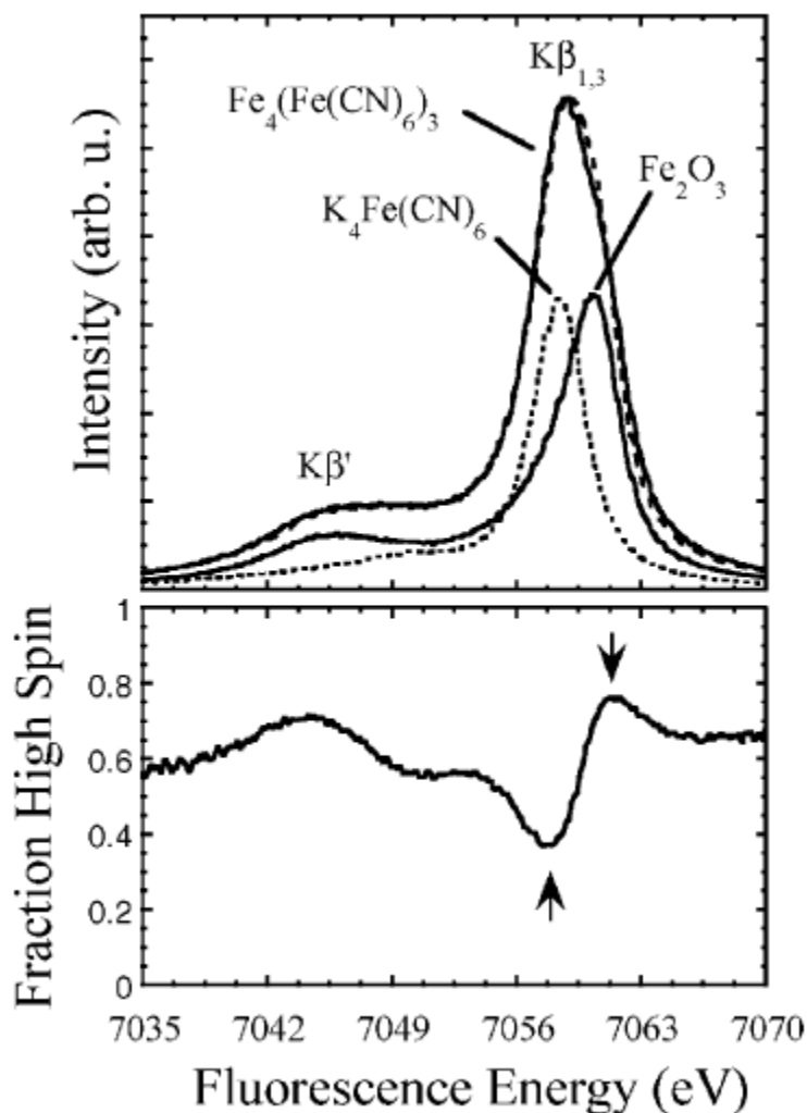
Figure 2-16 : Haut : Spectres d'émission issu des raies Kβ du bleu de Prusse ( \text{Fe}_4[\text{Fe}(\text{CN})_6]_3 ) avec les deux composés de références ( \text{Fe}_2\text{O}_3 et \text{K}_4\text{Fe}(\text{CN})_6 ). Bas : Estimation de la fraction en configuration haut-spin dans le bleu de Prusse en utilisant les références \text{Fe}_2\text{O}_3 et \text{K}_4\text{Fe}(\text{CN})_6 . Les flèches indiquent l'énergie de fluorescence à laquelle les spectres d'absorption ont été enregistrés [27].
