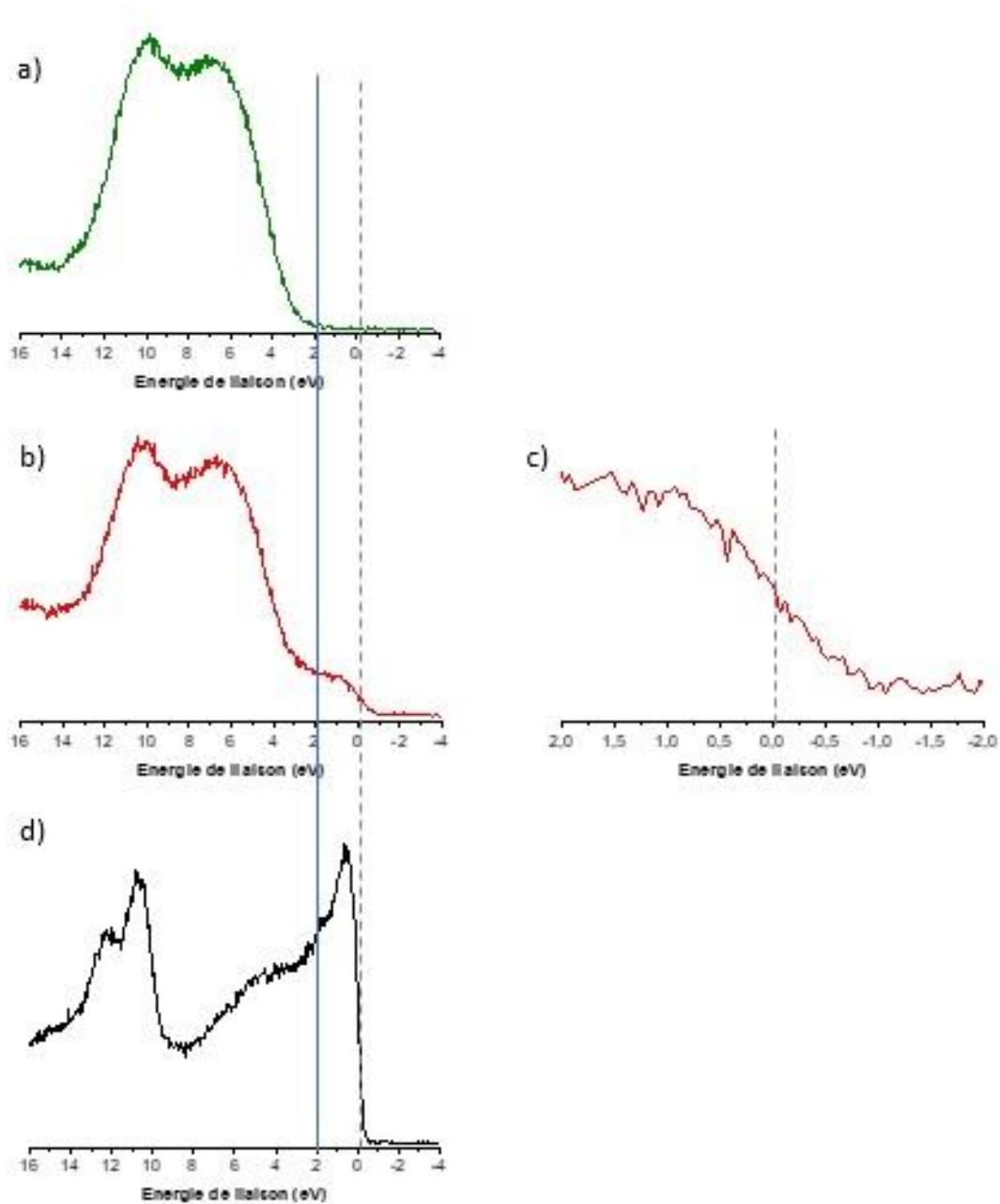
Figure 4-60 : Spectres XPS des bandes de valences de : a) \text{Al}_2\text{O}_3\text{-}\gamma , b) \text{CoEn}/\text{Al}_2\text{O}_3 sulfuré à 400^\circ\text{C} , c) Zoom entre 2 et - 2 eV pour \text{CoEn}/\text{Al}_2\text{O}_3 sulfuré à 400^\circ\text{C} , d) \text{Co}_9\text{S}_8 , ligne verticale : niveau de Fermi calibré à 0 eV.
