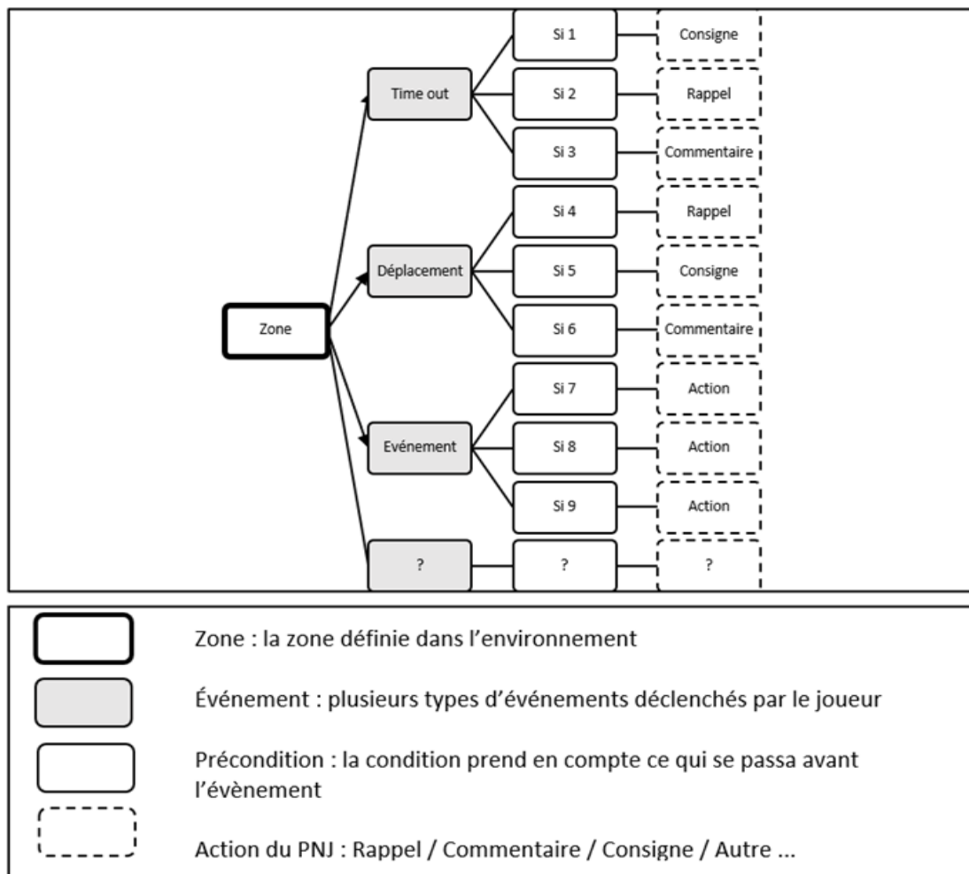
Figure 9. Structure du dialogue — Arbre à conditions, embranchements multiples avec états parallèles (Basé sur la structure de dialogue de Laurence Schmoll 2016).
