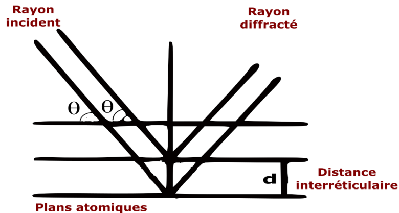
Figure 2.25. Schéma illustrant la diffraction des rayons sur deux plans réticulaires.
