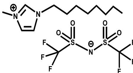
1-Méthyl-3-n-octylimidazolium bis(trifluorométhylsulfonyl)imide
