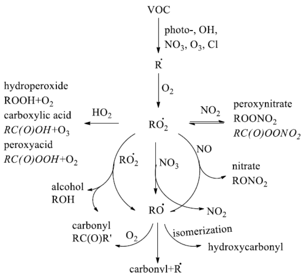
Figure 1-15 Réactions des radicaux alkylperoxy ( \text{RO}_2 ). Les produits en italique sont formés à partir de réactions de radicaux acylperoxy ( \text{RC(O)O}_2 ) (adaptation de Ziemann and Atkinson, 2012).
