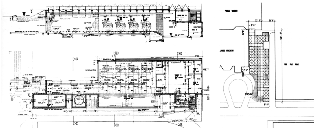
figure 1.2 Jeremy Dixon, projet de diplôme, chaufferie, 1961, AA Archives.
