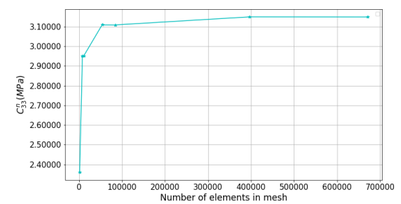
(d) C_{33}^n
