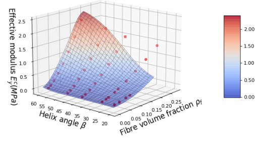
(b) E_y^c
