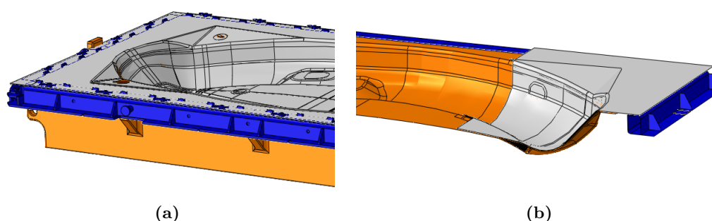
Figure 11 – CAO de l'ensemble moule cadre et tôle: (a) CAO 3D des pièces et (b) version surfaciues simplifiées
