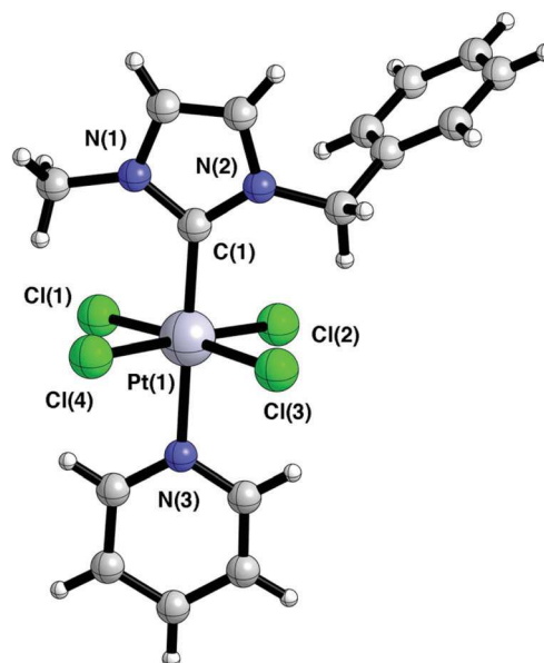
Fig. 1 Molecular structure of Pt(IV) NHC complex 1 Cl .† Selected bond distances (Å) and angles (°): C(1)–Pt(1), 2.034(11); Cl(1)–Pt(1), 2.329(3); Cl(2)–Pt(1), 2.327(3); Cl(3)–Pt(1), 2.336(3); Cl(4)–Pt, 2.330(3); N(3)–Pt(1), 2.127(9); C(1)–Pt(1)–N(3), 178.4(4); C(1)–Pt(1)–Cl(2), 91.6(4); N(3)–Pt(1)–Cl(2), 89.2(3); Cl(2)–Pt(1)–Cl(4), 177.34(12); Cl(1)–Pt(1)–Cl(4), 91.85(12).
