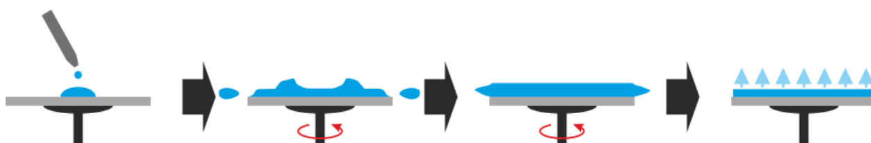
Figure 8. Schéma simplifié du procédé par enduction centrifuge. g
