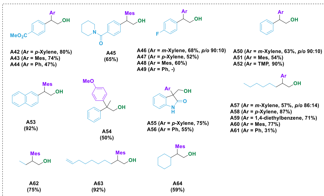
Schéma 2. Monoarylation d'époxydes. [a] A 0 °C. [b] [C] = 0.2 M. [c] En utilisant Bi(OTf) 3 /nBu 4 NPF 6 (5mol%) comme promoteur. [d] En présence de TfOH (0.1 mol%). Mes = 1,3,5-triméthylphényle. TMP = 1,3,5-triméthoxyphényle.
