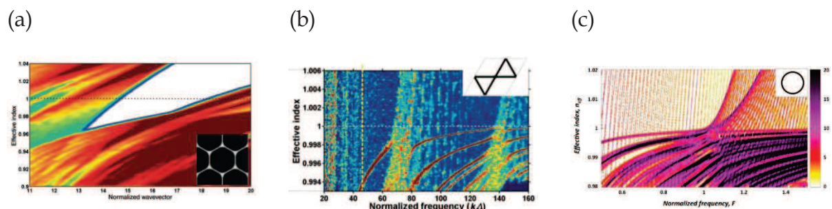
Figure 1-5 : DOPS de (a) BIP à cœur creux (b) structure Kagomé (c) Structure tubulaire.
