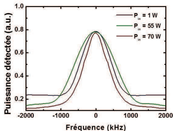
Figure 9-4 : Evolution de la largeur de bande de la pompe à travers la fibre pour différentes puissances d'entrée 1 W (courbe bleue), 55 W (courbe verte) et 70 W (courbe rouge)[125].
