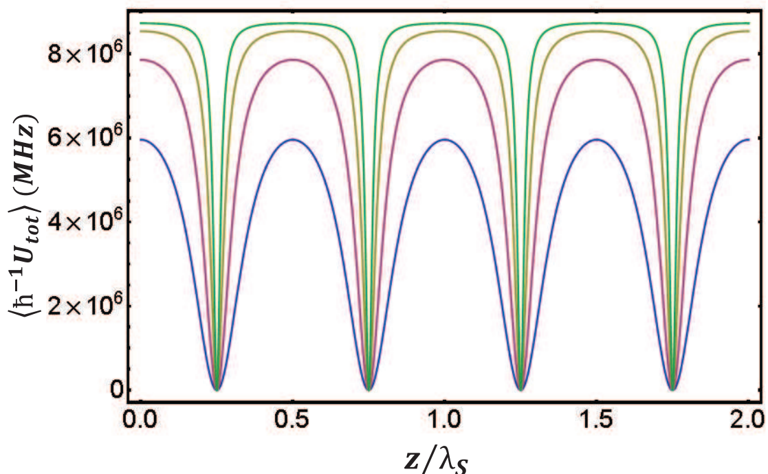
Figure 8-4 : Potentiel moyen total en fonction de z/\lambda_S .
