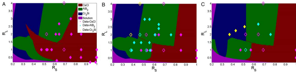
Figure 20 : Diagrammes de phases de nanoparticules d'or en fonction de la taille des nanoparticules (RS) ou de la longueur du linker (RL) pour trois stœchiométries différentes : (A) 1 :1, (B) 2 :1, (C) 3 :1. Les symboles r eprésentent les poi nts e xpérimentaux : l es symboles p leins r eprésentent l es s tructures p ures tandis que l es v ides r eprésentent de s s tructures p olymorphes. O n observe g lobalement une bonn e concordance entre points expérimentaux et résultats théoriques (Vo et al. , 2015).
