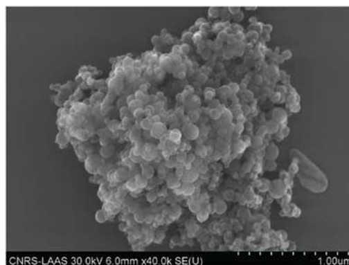
Figure 8 : Image MEB d'un nanocomposite obtenu à partir de l'auto-assemblage de nanoparticules d'Al et de CuO par ADN (Séverac et al. , 2012).
