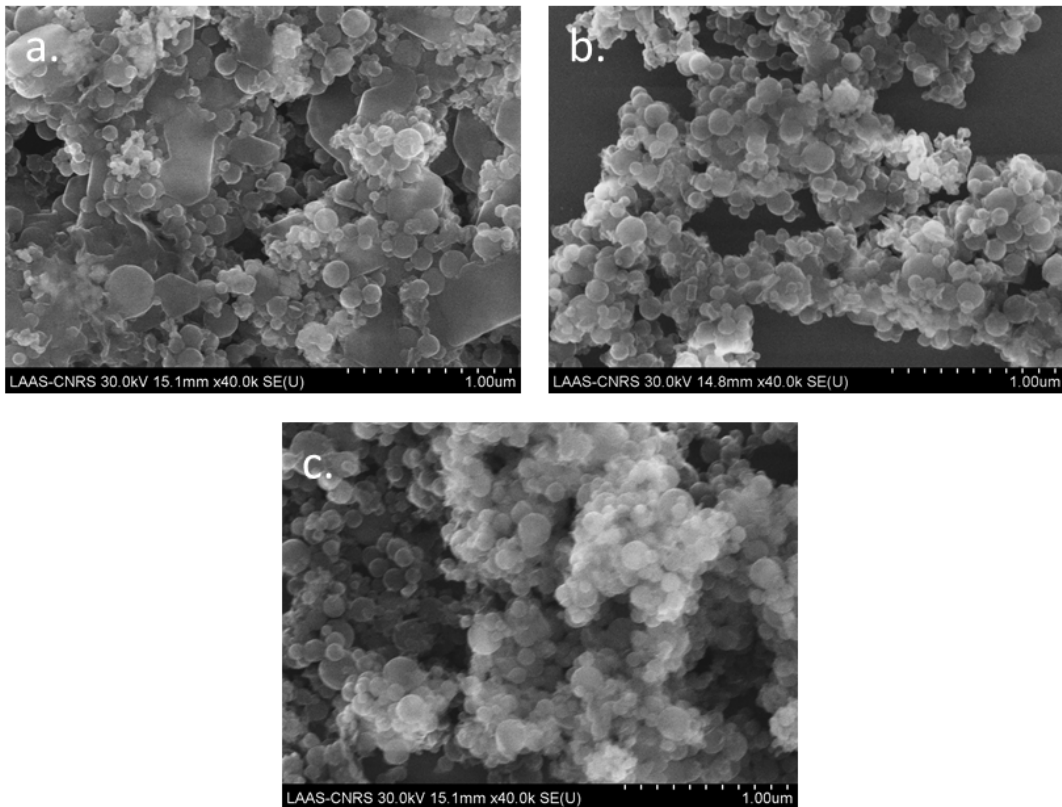
Figure 114 : Images SE Mc caractéristiques de nanocomposites Al-CuO ayant un rapport stœchiométrique de 1, 2 et 4 (images (a), (b) et (c) respectivement).
