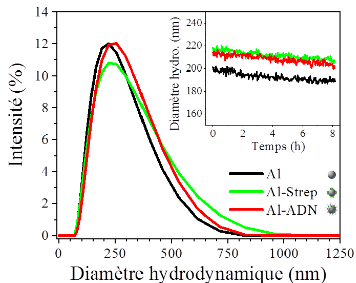
Figure 78 : Distribution en taille des nanoparticules d'Al avant (courbe noire), après greffage de la Streptavidine (courbe verte) et après greffage de l'ADN intermédiaire (courbe rouge) et stabilité des solutions colloïdales (encadré supérieur droit).
