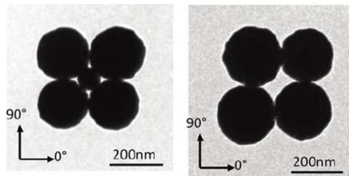
Figure 24 : Images TEM de structures anisotropes obtenues par auto-assemblage de deux types de nanoparticules d'or de taille différente. Fan et al. ont alors comparé les propriétés optiques de ces clusters avec ou sans nanoparticule de petite taille et ont montré une amélioration de celles-ci (Fan et al. , 2011).
