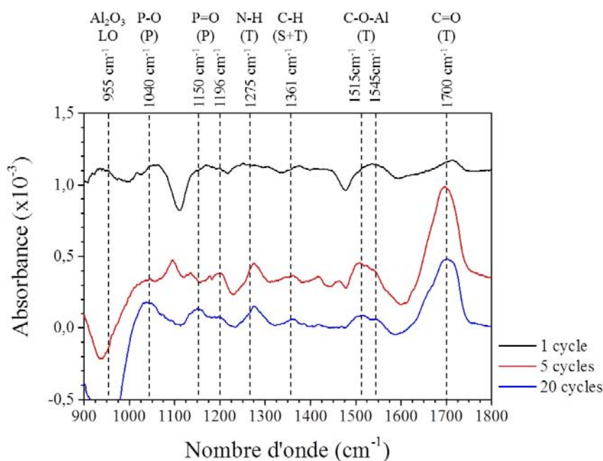
Figure 47 : Spectres d'absorbance de la surface d' \text{Al}_2\text{O}_3 après incubation dans une solution aqueuse de dTMP ( 50 \mu\text{M} ) pendant 1 h à 30^\circ\text{C} en fonction du nombre de cycles de dépôt par ALD (1, 5 et 20 cycles, c'est-à-dire 0,2 nm, 0,5 nm et 2 nm environ). La référence est prise sur la surface d' \text{Al}_2\text{O}_3 correspondante avant réaction.
