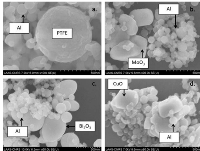
Figure 4 : Images SEM des nanothermites après mélange de poudre (a) Al-PTFE, (b) Al-MoO 3 , (c) Al-Bi 2 O 3 , (d) Al-CuO (Glavier et al., 2015).
