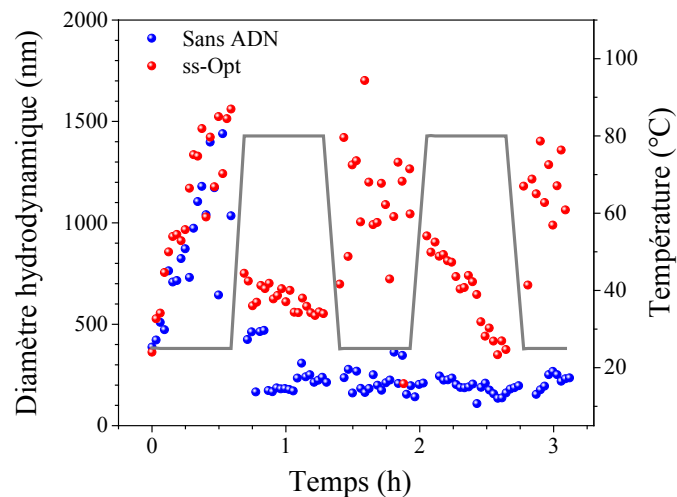
Figure 99 : Evolution du diamètre hydrodynamique moyen d'une solution colloïdale de nanoparticules d'Al et de CuO non-fonctionnalisées ( courbe bleue) et fonctionnalisées avec des brins d'ADN complémentaires (courbe rouge) pour une concentration en NaCl de 35 mM en fonction de la température (courbe grise).
