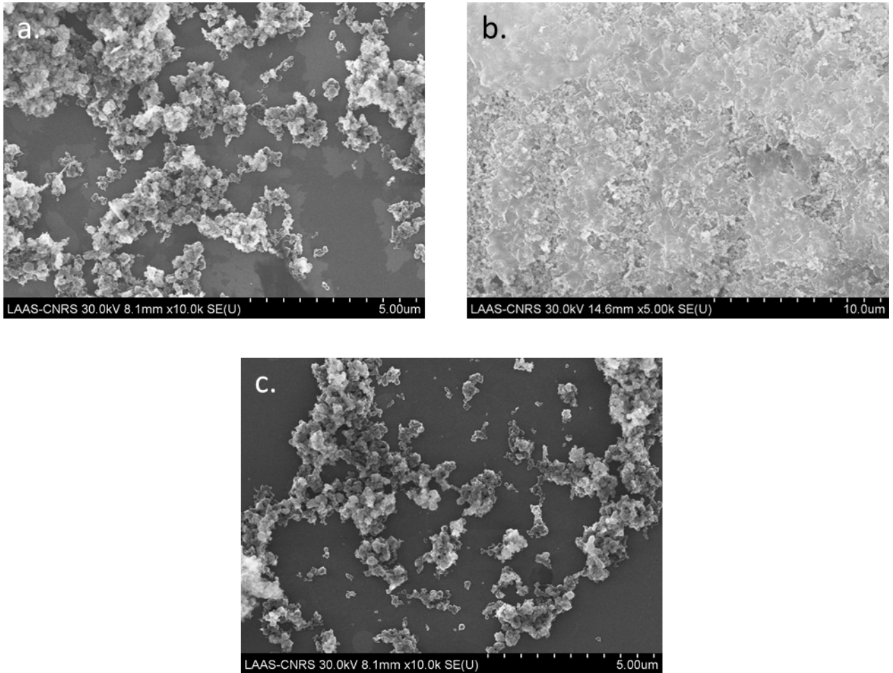
Figure 142 : Images SEM de nano biocomposites Al-CuO obtenus avec des brins d'ADN complémentaires et optimisés pour une concentration en NaCl 250 mM.
