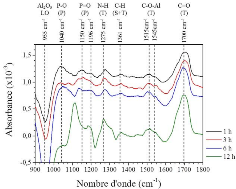
Figure 42 : Spectres d'absorbance des surfaces d' \text{Al}_2\text{O}_3 après incubation dans une solution de dTMP concentrée à 50 \mu\text{M} à 30 ^\circ\text{C} , en fonction de la durée d'incubation (1h, 3h, 6h et 12h). Pour chaque courbe, la référence est prise sur la surface d' \text{Al}_2\text{O}_3 propre, avant incubation.
