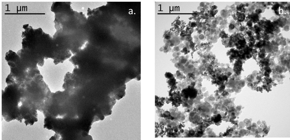
Figure 118 : Images TEM des nanocomposites réalisés par mélange de nanoparticules d'Al et de CuO (a) et par assemblage avec des brins d'ADN optimisés et complémentaires (b).
