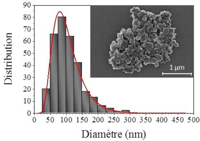
Figure 52 : Distribution statistique du diamètre de nanoparticules d'Al fournies par US Research Nanomaterials et image SEM de nanoparticules d'Al dispersées dans l'éthanol.
