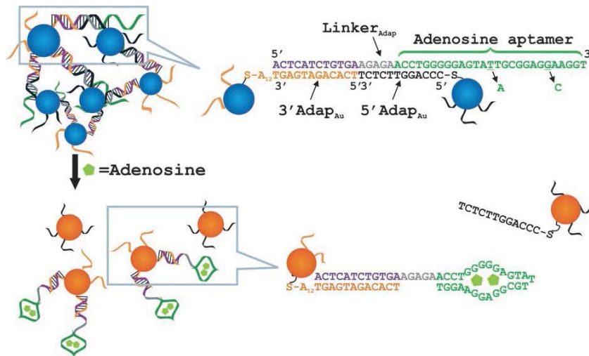
Figure 16 : Schéma de principe de la détection de l'Adénosine par méthode colorimétrique. Des nanoparticules d'or fonctionnalisées avec des brins d'ADN sont agrégées grâce à la présence d'un aptamère 8 complémentaire avec l'Adénosine. Ainsi, en présence de la molécule cible, les aptamères s'hybrident sur la molécule entraînant une désagrégation des nanoparticules et un changement colorimétrique de la solution, passant du bleu au rouge (Liu and Lu, 2006).
