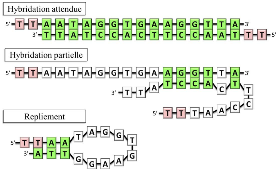
Figure 94 : Schéma représentant les interactions parasites possibles du brin d'ADN à la séquence issue de (Zhang et al. , 2013b). (a) hybridation attendue, sur la totalité du brin d'ADN, (b) hybridation partielle avec un brin complémentaire, (c) repliement du brin sur lui-même ou, a fortiori, avec un brin identique. Les doubles bases vertes indiquent les bases hybridées, les bases rouges indiquent les bases intégrant le spacer, et les bases blanches indiquent les bases neutres vis-à-vis de l'hybridation.
