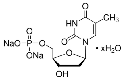
Figure 29 : Formule chimique de la Thymidine 5'-monophosphate de sodium salin hydratée (Sigma Aldrich).
