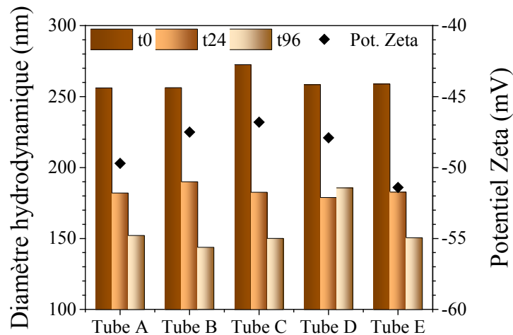
Figure 59 : Diamètre hydrodynamique moyen et potentiel Zeta de la solution colloïdale de CuO en fonction de la durée de sédimentation et de la composition de la solution.
