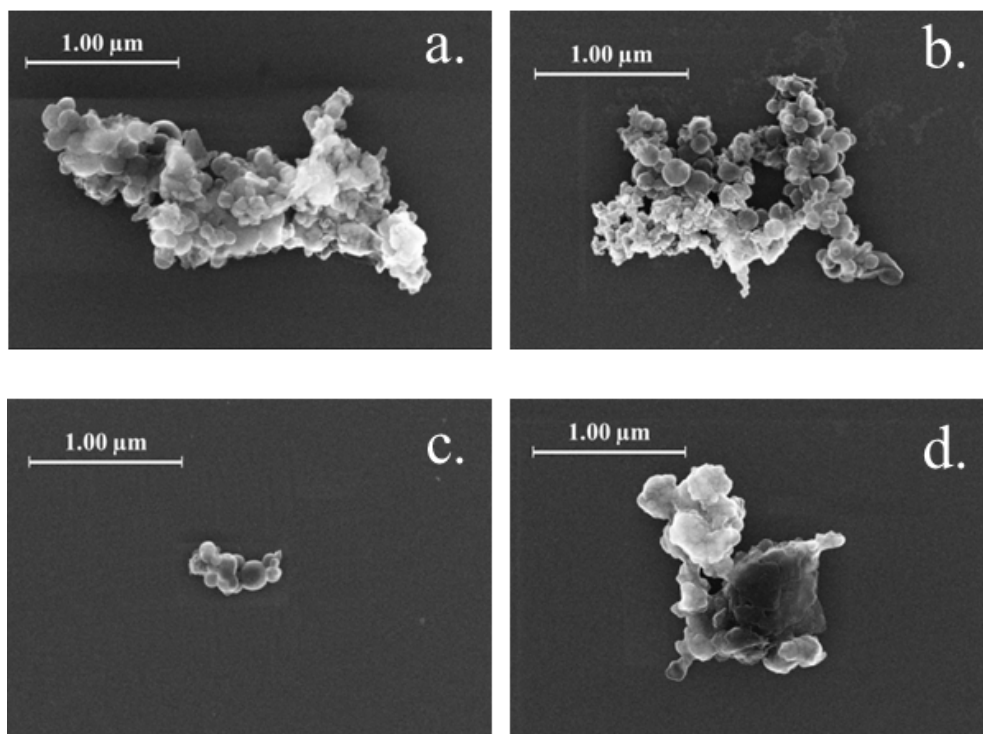
Figure 111 : ( a, b ) Images SEM de nano biocomposites Al-CuO obtenus par agrégation de nanoparticules fonctionnalisées avec des brins d'ADN optimisés, complémentaires et non-complémentaires respectivement. ( c, d ) Images SEM de nano biocomposites Al-CuO obtenus par agrégation de nanoparticules fonctionnalisées avec des brins d'ADN non-optimisés, complémentaires et non-complémentaires respectivement.
