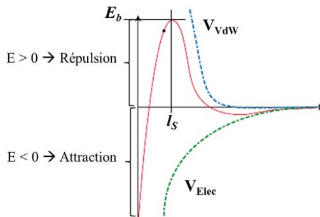
Figure 90 : Visualisation graphique du potentiel d'interaction s'appliquant entre deux nanoparticules, comme étant la somme du potentiel électrostatique (ici en interaction répulsive) et du potentiel de Van der Waals, interaction attractive. Représentation de la barrière énergétique E_b et de la longueur d'écran l_s .
