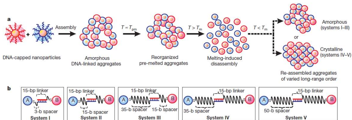
Figure 21 : Schéma présentant le comportement de s agrégats de n anoparticules issus de l'auto-assemblage par ADN face à la température et de la longueur des brins d'ADN utilisés (Nykypanchuk et al. , 2008).
