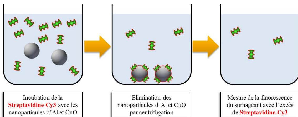
Figure 81 : Schéma présentant la stratégie de quantification indirecte de la Streptavidine fluorescente (en rouge) greffée sur les nanoparticules d'Al ou de CuO, en trois étapes.
