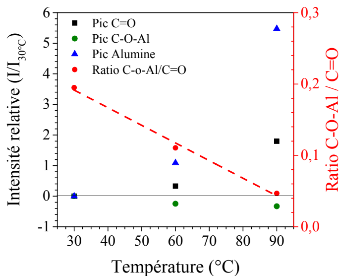
Figure 40 : Evolution de l'intensité relative des pics à 1700 cm -1 (courbe noire), à 1515 cm -1 (courbe verte) et à 955 cm -1 (courbe bleue), normalisées par rapport à l'intensité obtenue pour une température d'incubation de 30 °C) et du ratio C-O-Al / C=O (courbe rouge), en fonction de la température.
