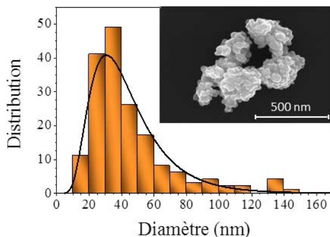
Figure 51 : Distribution statistique du diamètre de nanoparticules de CuO fournies par Sigma Aldrich, et image SEM de nanoparticules de CuO dispersées dans l'éthanol.
