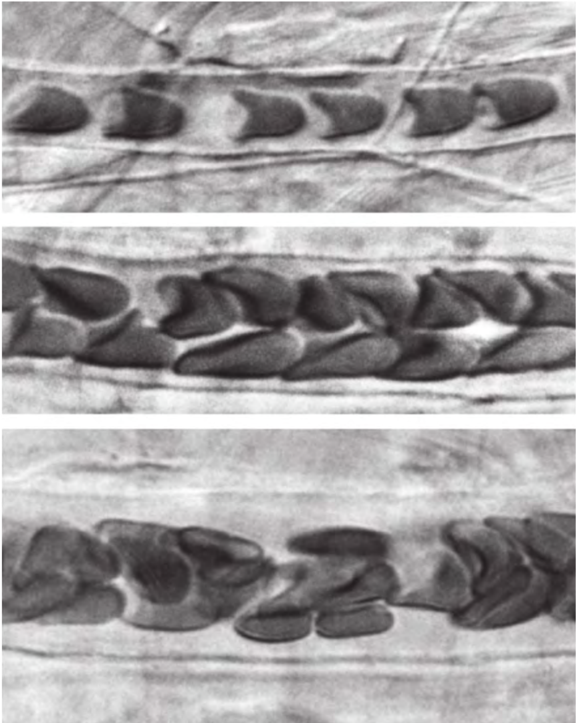
Figure 3.2 – Effet Fâhareus in vivo dans le mésentère du rat pour des vaisseaux de 7, 12 et 16 \mu\text{m} de diamètres .Le sang s'écoule de gauche à droite. Extrait de TUMA et collab. [2002]
