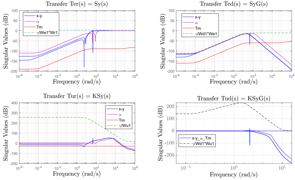
Figure 7: Réponse fréquentielle de la boucle fermée avec les gabarits fréquentiels (pointillés) avec schéma de synthèse \mathcal{H}_\infty à quatre blocs.
