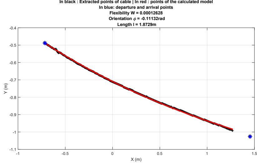
Figure 5: La reconstruction du câble à partir de la vidéo
