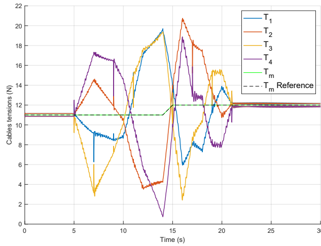
Figure 11: Tensions des câbles et tension moyenne de référence avec la synthèse \mathcal{H}_\infty .
