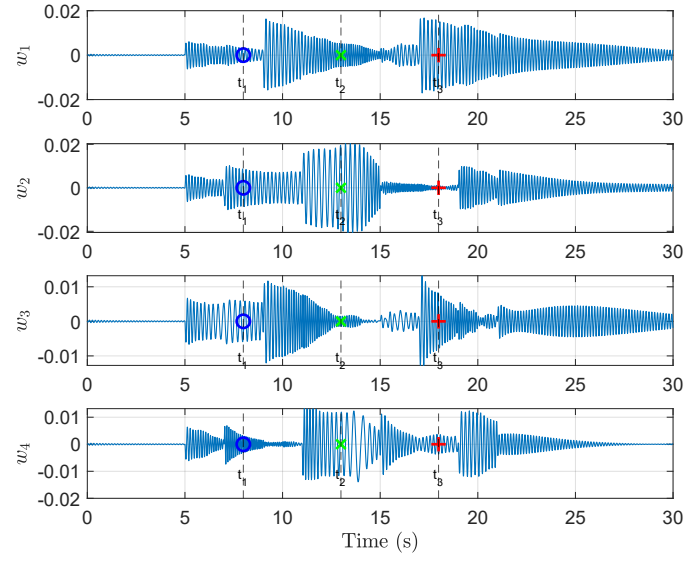
Figure 12: Coordonnées modales pour la flexibilité des câbles avec la synthèse \mathcal{H}_\infty .
