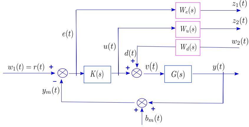
Figure 6: Le schéma de synthèse à quatre blocs.
