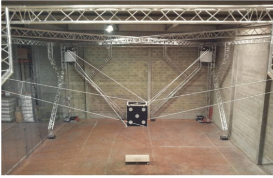
(b) The CoGiRo robot (source: www.lirmm.fr/cogiro )
