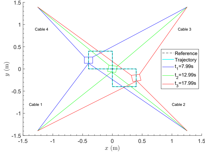
Figure 8: Trajectoires de la plate-forme et des câbles dans le plan x - y avec le correcteur \mathcal{H}_\infty .
