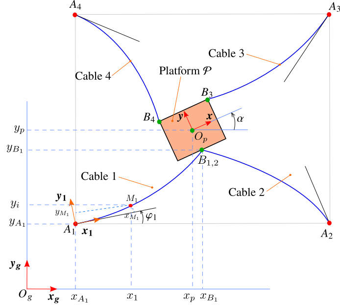
Figure 2: Représentation d'un robot parallèle plan à 4 câbles flexibles.
