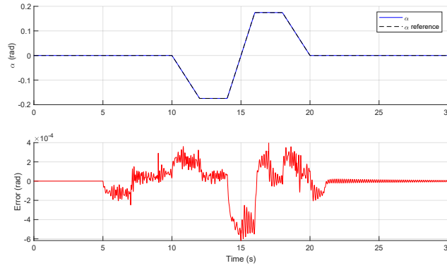
Figure 9: Trajectoires d'orientation de la plate-forme pour le contrôle \mathcal{H}_\infty avec la synthèse à quatre blocs.
