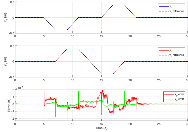
Figure 10: Suivi et erreur des trajectoires x_p et y_p avec correcteur \mathcal{H}_\infty avec la synthèse à quatre blocs.
