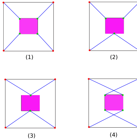
Figure 3: Différents scénarios pour différents points d'attache de câbles.
