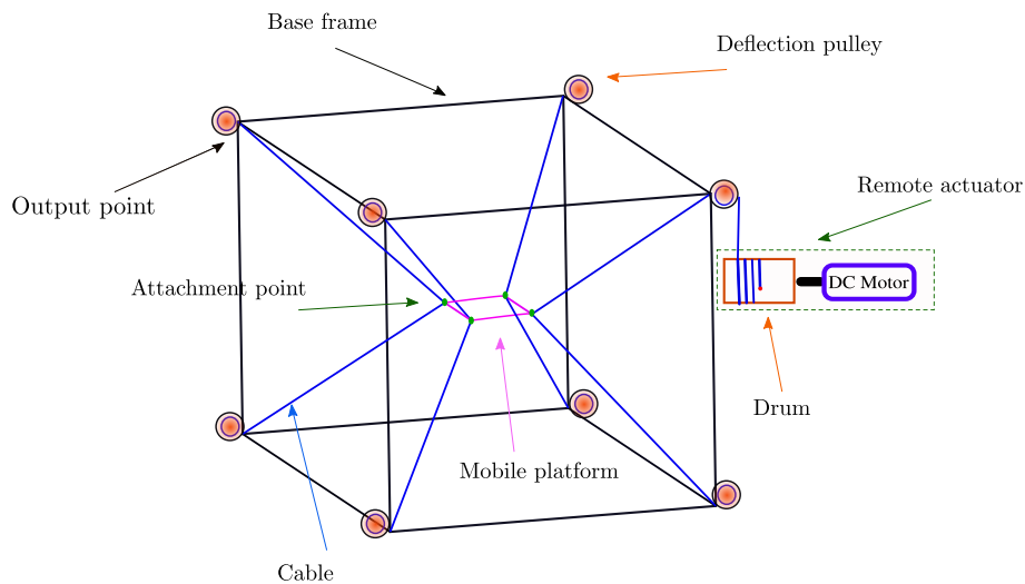
Figure 1: Structure d'un robot parallèle à 8 câbles et 6 degrés de liberté.
