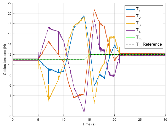
Figure 11: Tensions des câbles et tension moyenne de référence avec la synthèse \mathcal{H}_\infty .
