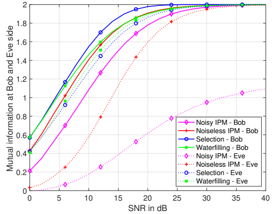
(b) 16-QAM(2bpcu)
