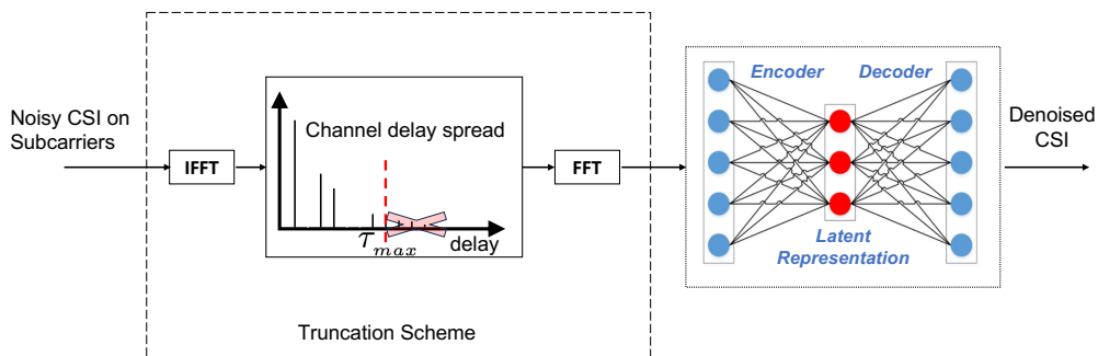
Algorithme DAE HybDenoisedSecNet proposé.
