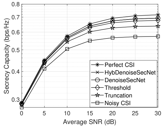
(b) Performances en matière de sécurité avec DenoiseSecNet.
