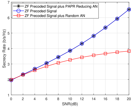
(a) Zero-Forcing à \theta = 0.9 .
