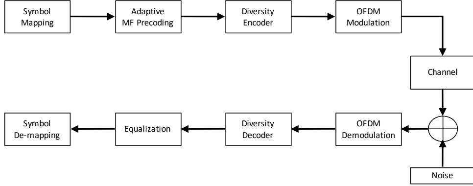
Modèle de système OFDM utilisant la diversité et la technique PLS adaptative.
