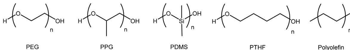
Figure 2-6 : Structures Chimiques de quelques polymères liquides utilisés comme solvants (gauche à droite) : Polyéthylène Glycol, Polypropylène Glycol, Poly(diméthylsiloxane) (PDMS), poly(tétrahydrofurane) (PTHF) et une polyoléfine.
