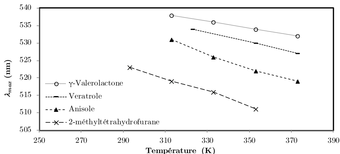
Figure 5-7 : Variation de \lambda_{max} avec la température du Rouge de Nil dans l'anisole, le vératrole, la \gamma -valerolactone et le 2-méthyltétrahydrofurane.
