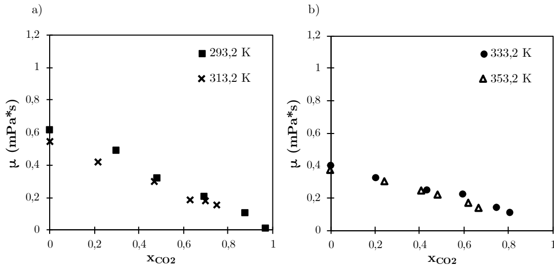
Figure 7-14 : Viscosité vs fraction molaire pour le système \text{CO}_2 + 2 -méthyletetrahydrofurane : a) 293,2K et 313,2K, et b) 333,2K et 353,2K.
