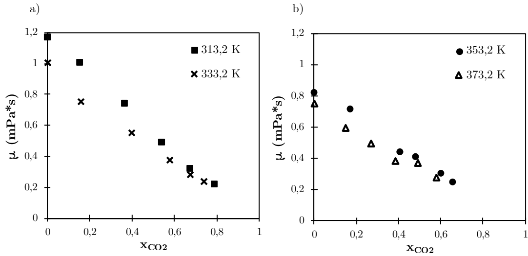
Figure 7-13 : Viscosité vs fraction molaire pour le système \text{CO}_2 + \gamma -valérolactone : a) 313,2K et 333,2K, et b) 353,2K et 373,2K.
