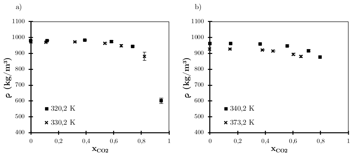
Figure 6-6 : Masse volumique vs fraction molaire pour le système CO_2 +carbonate de diéthyle : a) 320,2K et 330,2K et b) 340,2K et 373,2K.
